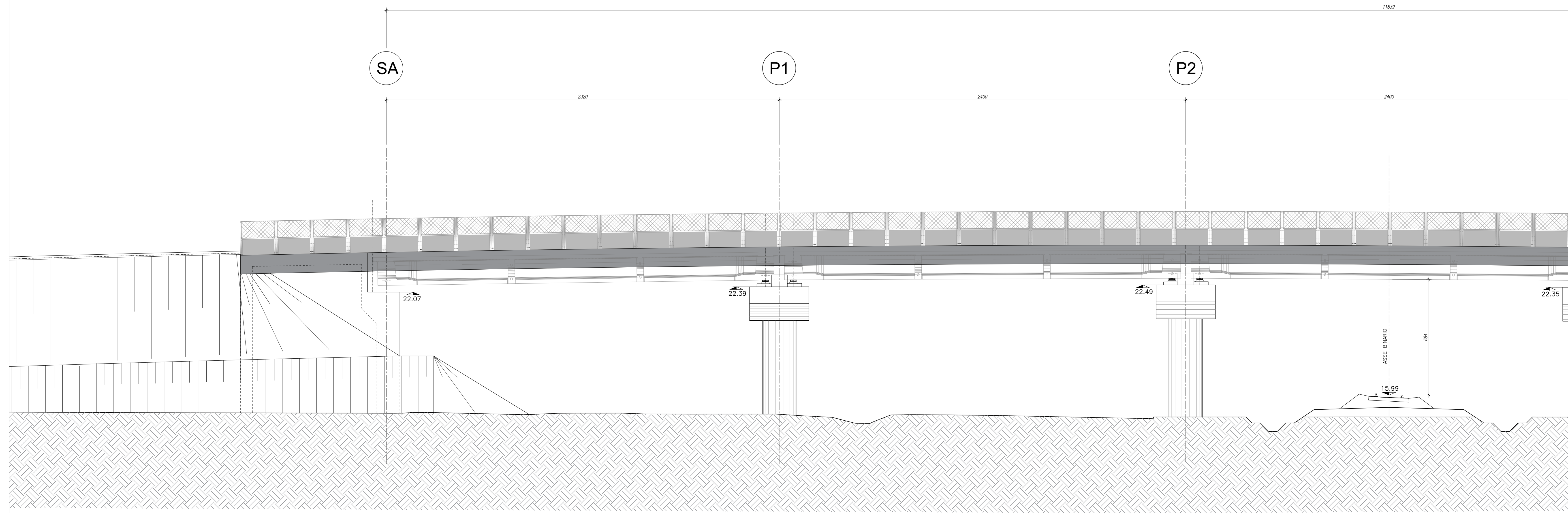
PROSPETTO LATERALE 1/2 Scala 1:100
