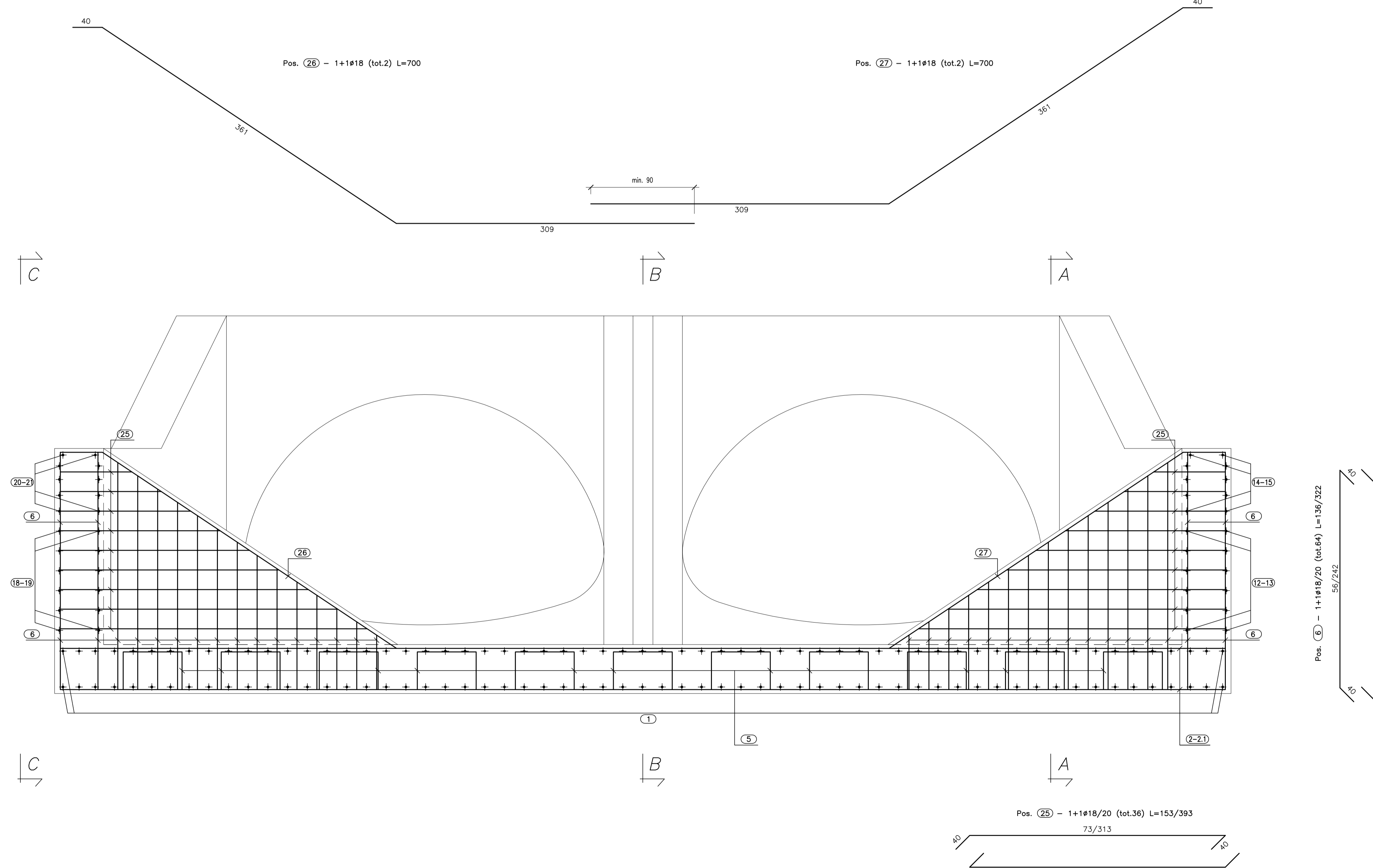
VISTA. D-D (SCALA 1:25)
