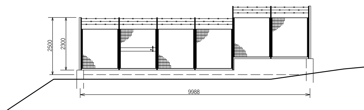
PROSPETTO A – Scala 1:100
