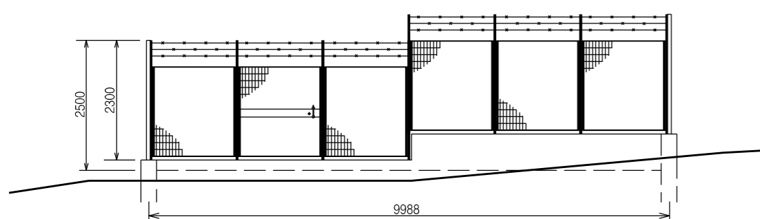
PROSPETTO A – Scala 1:100
