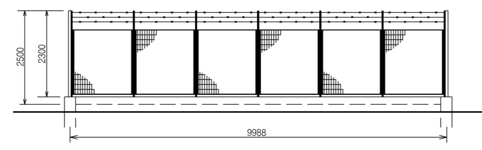
PROSPETTO B – Scala 1:100
