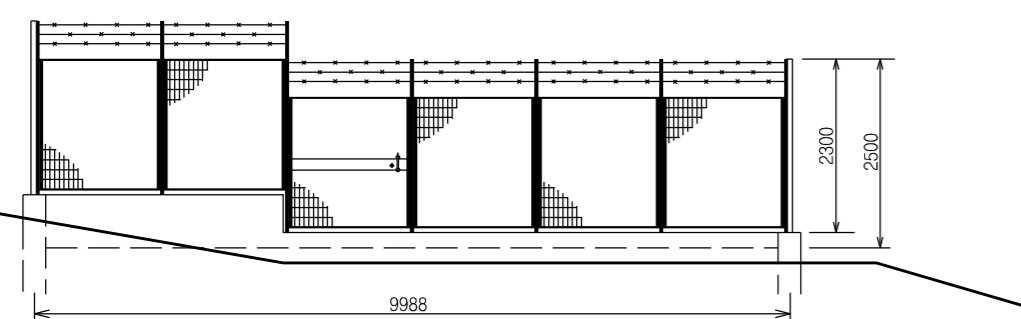
PROSPETTO A – Scala 1:100
