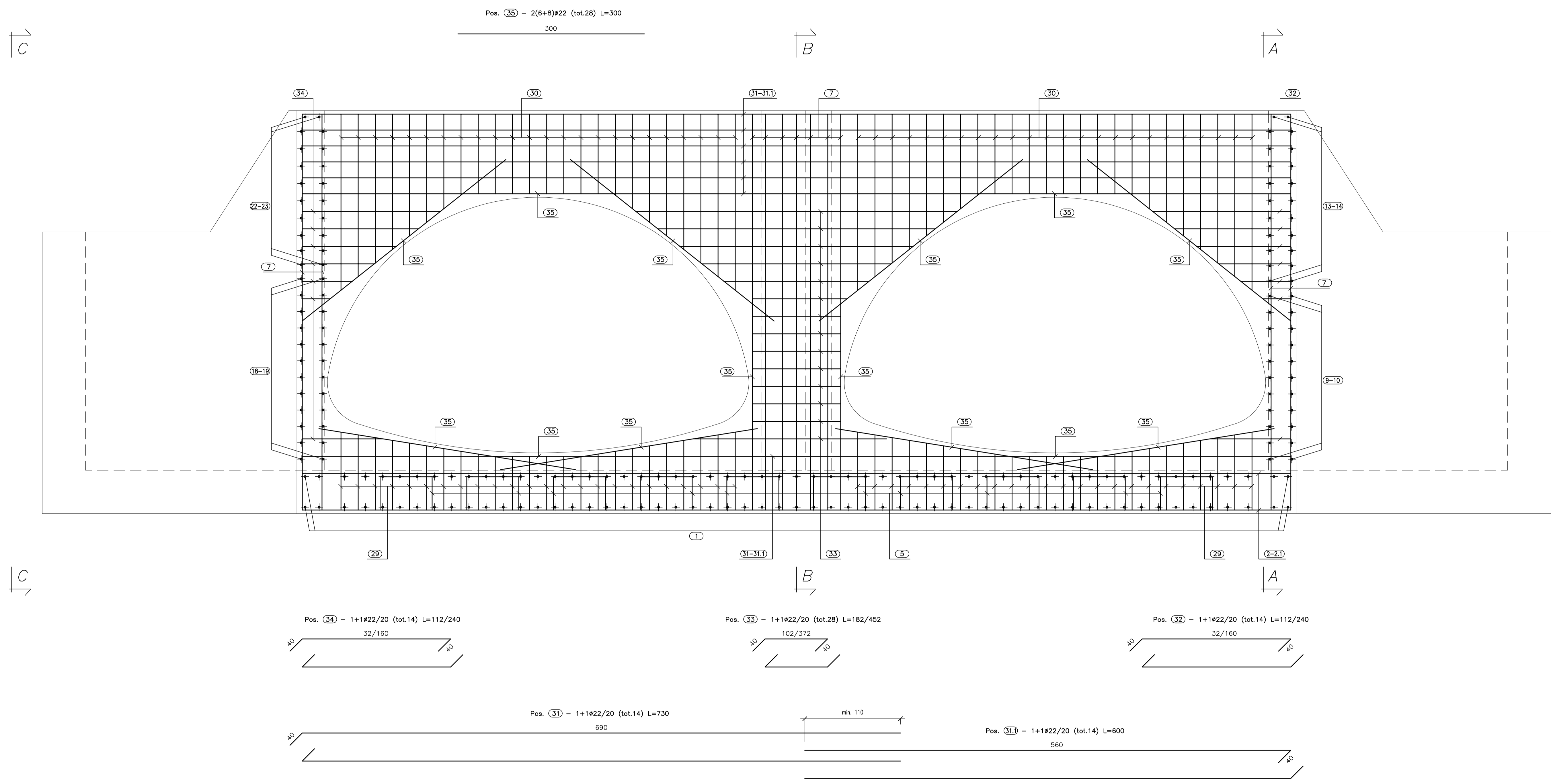
VISTA. E-E (SCALA 1:25)
