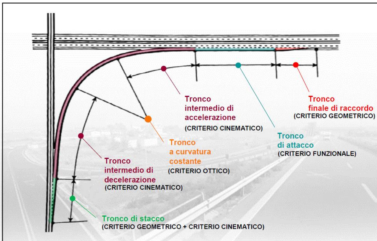
Figura 24: elementi planimetrici rampa
