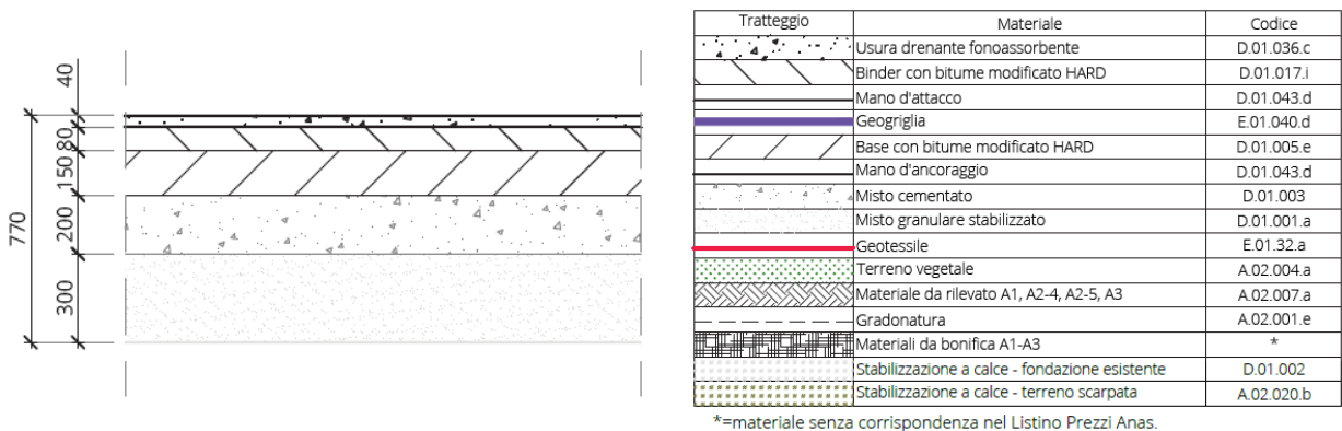
Figura 14: strati e spessori pavimentazione stradale
