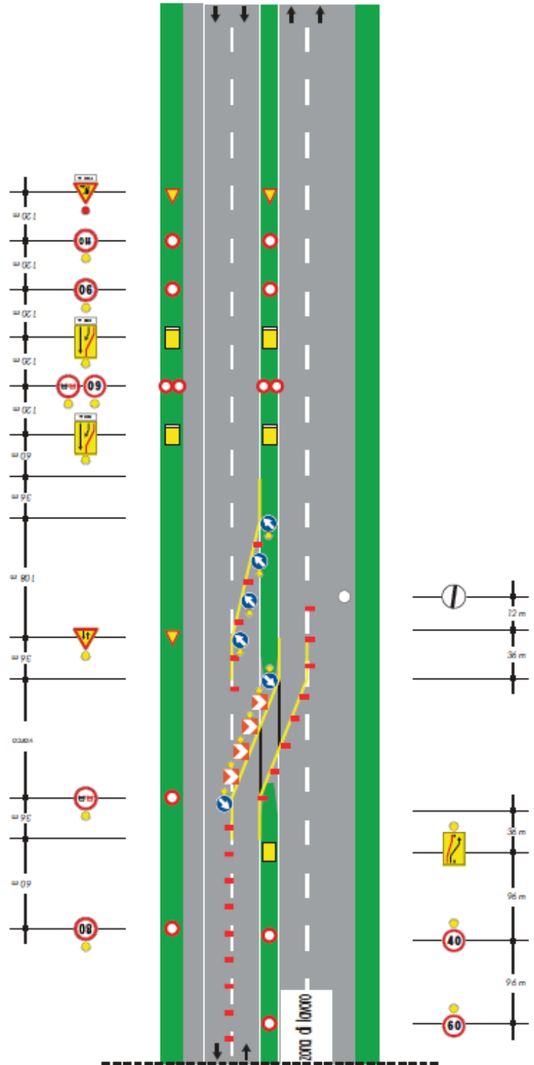
Figura 32: Segnaletica di cantiere - tavola 25a
