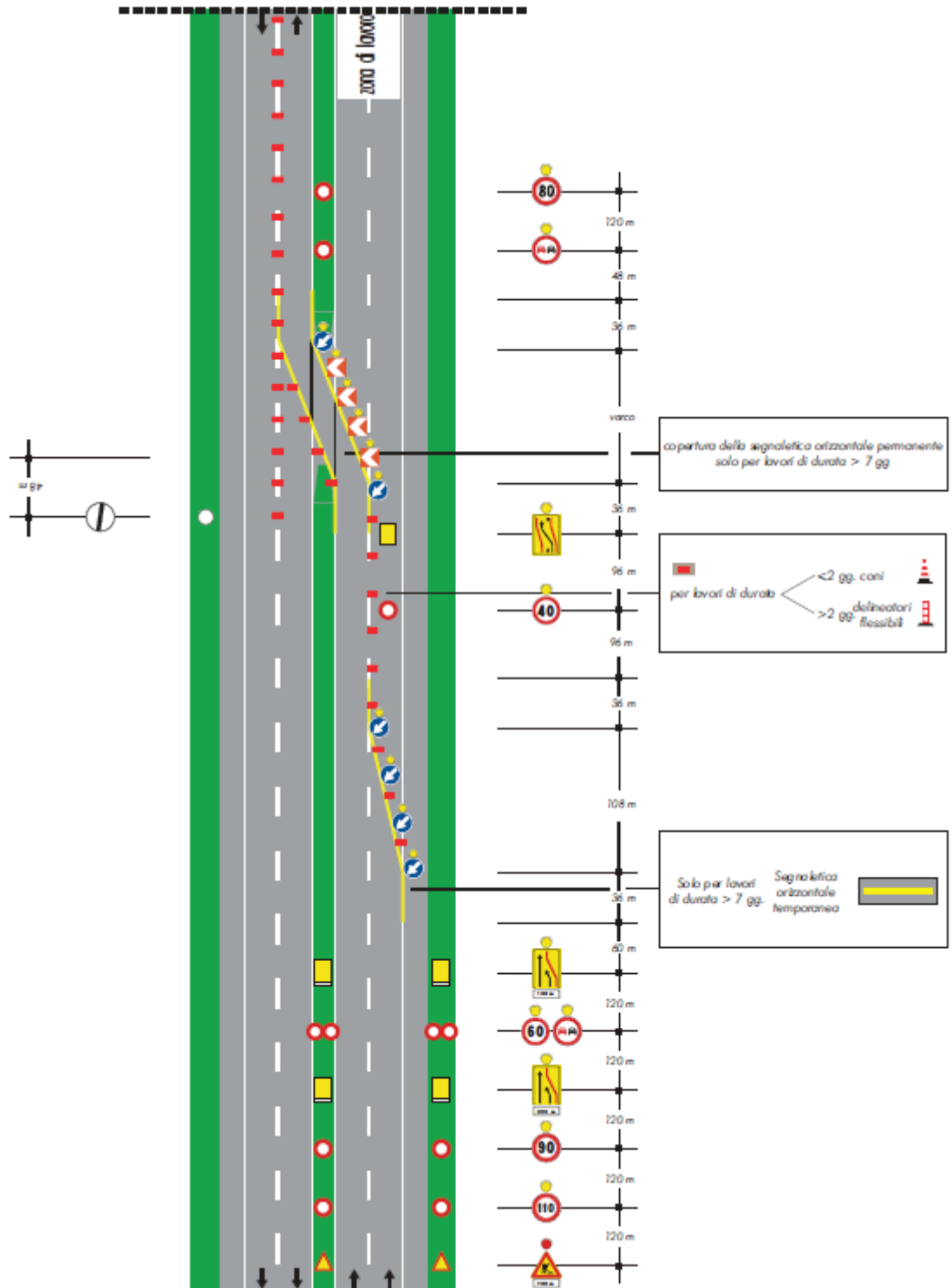
Figura 33: Segnaletica di cantiere - tavola 25b
