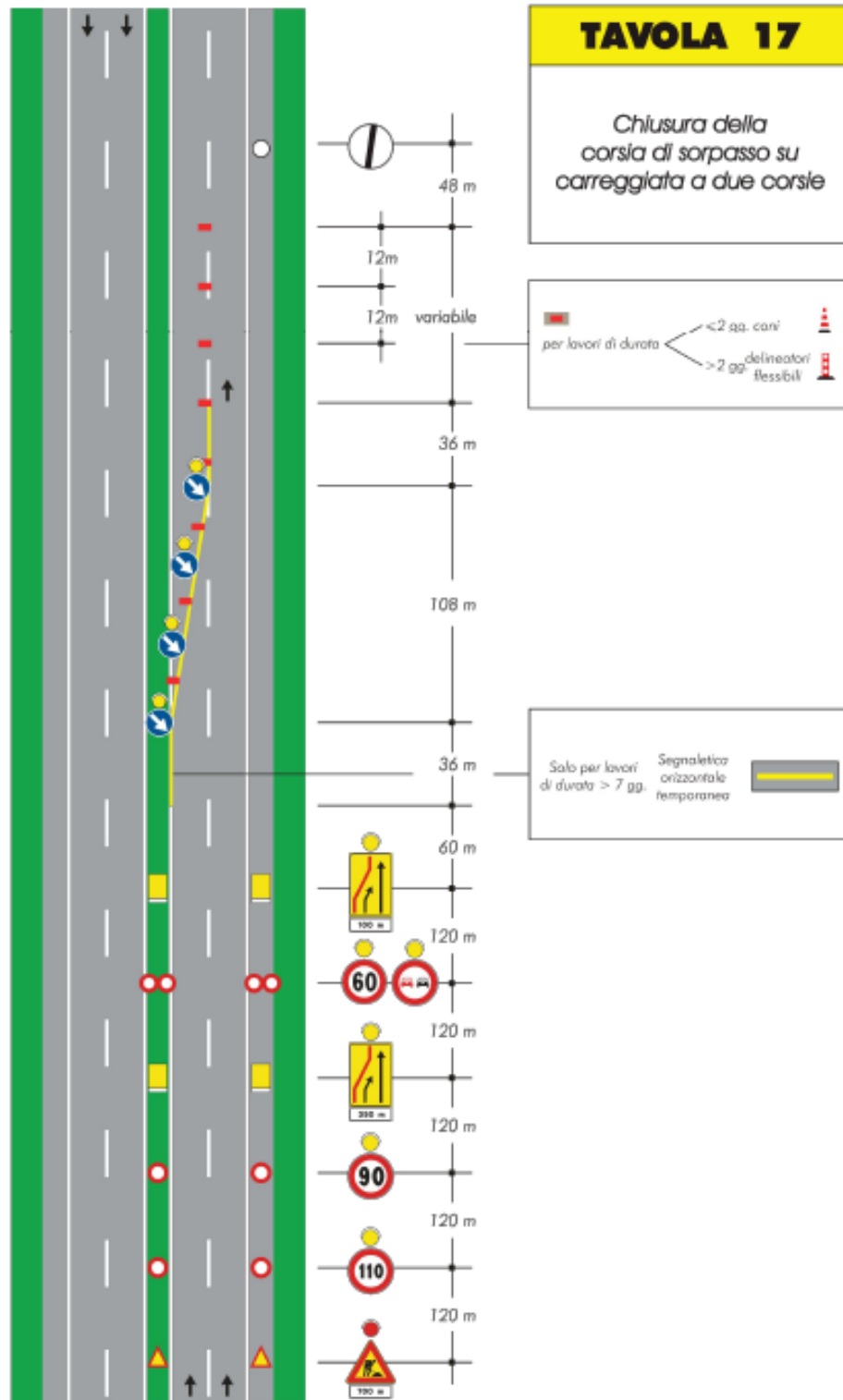
Figura 31: Segnaletica di cantiere - tavola 17
