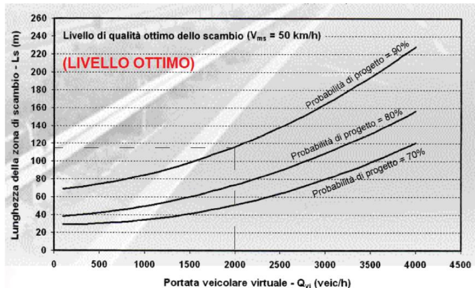
Figura 21: abaco per la determinazione della lunghezza della zona di scambio a livello ottimo
