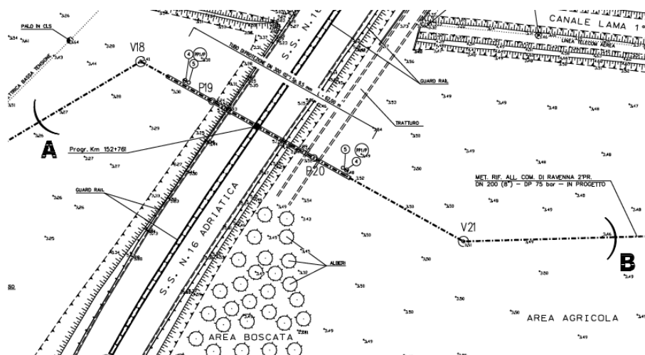
Figura 29: planimetria interferenza futura – Fonte Snam S.p.A.
