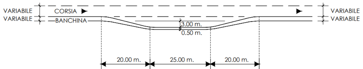
Figura 22: configurazione piazzola di sosta
