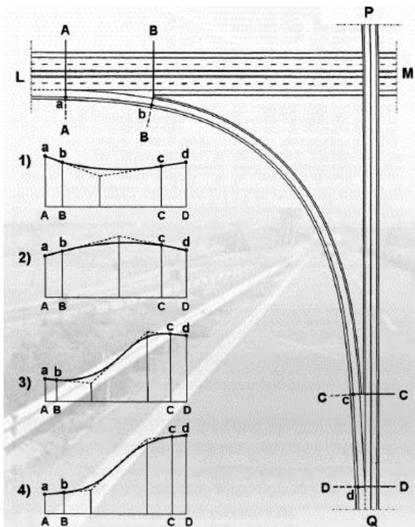
Figura 25: configurazione altimetria rampa
