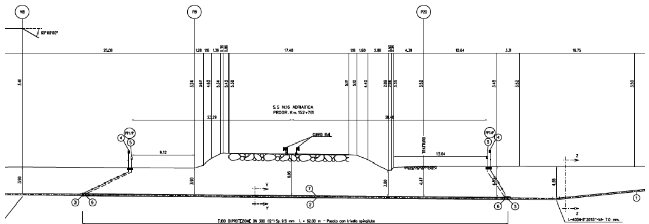
Figura 30: sezione interferenza futura – Fonte Snam S.p.A.
