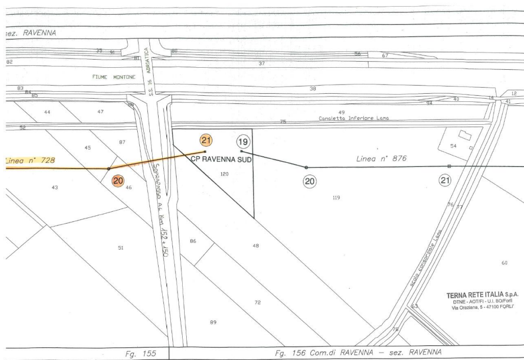
Figura 27: planimetria interferenza - Fonte Terna S.p.A.
