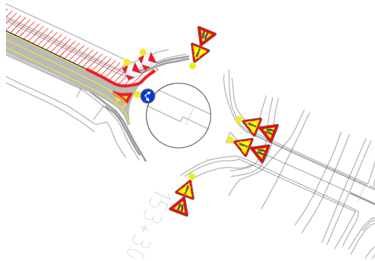
Figura 34: Segnaletica di cantiere intersezione a rotatoria
