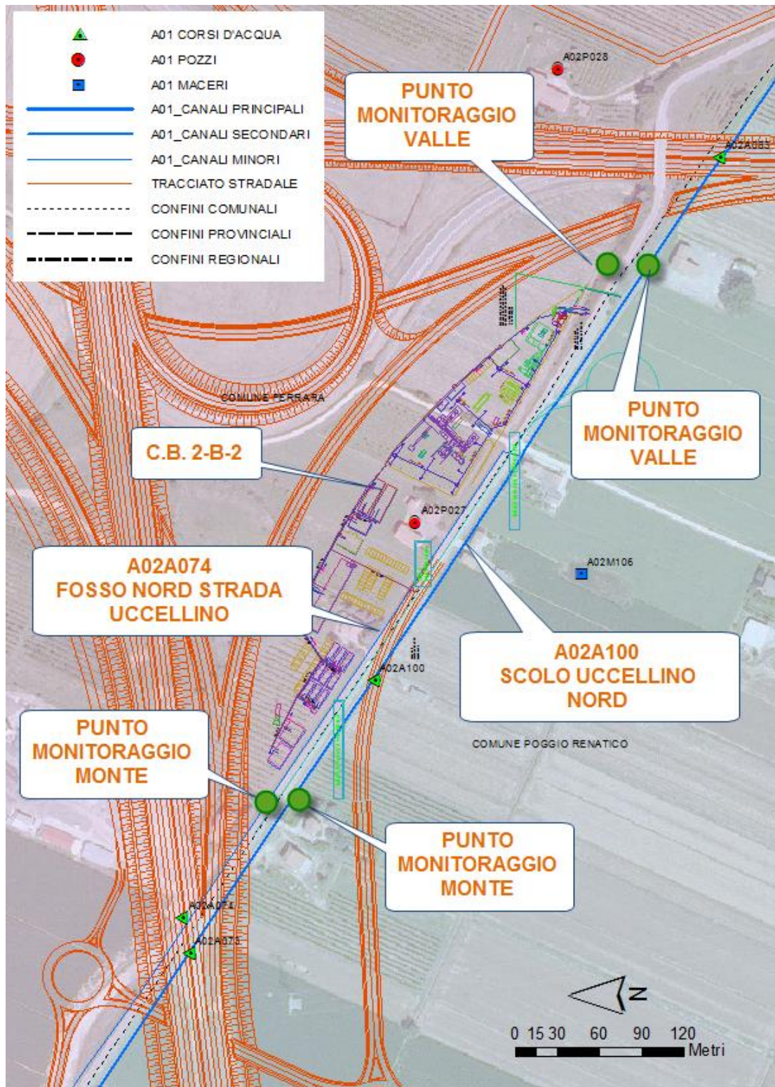
FIGURA 2.4-4 – LOCALIZZAZIONE DEI PUNTI DI MONITORAGGIO AGGIUNTIVI IN PROSSIMITÀ DEL C.B. 2-B.2
