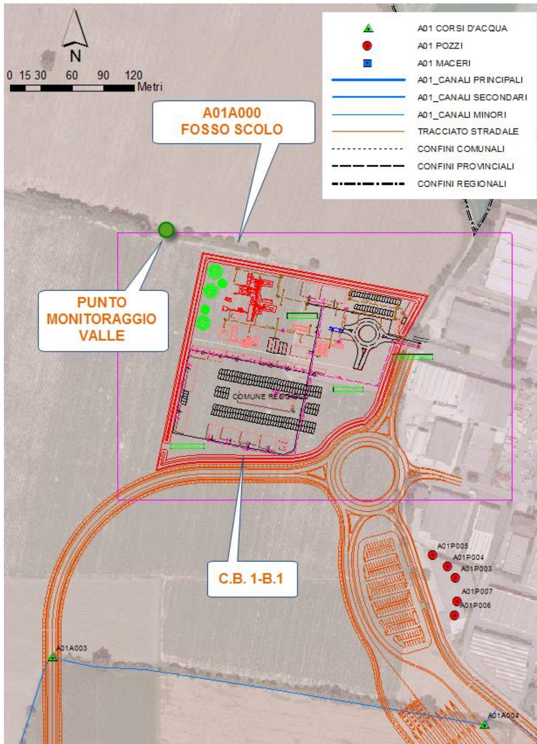
FIGURA 2.4-1 – LOCALIZZAZIONE DEL PUNTO DI MONITORAGGIO AGGIUNTIVO IN PROSSIMITÀ DEL C.B. 1-B.1
