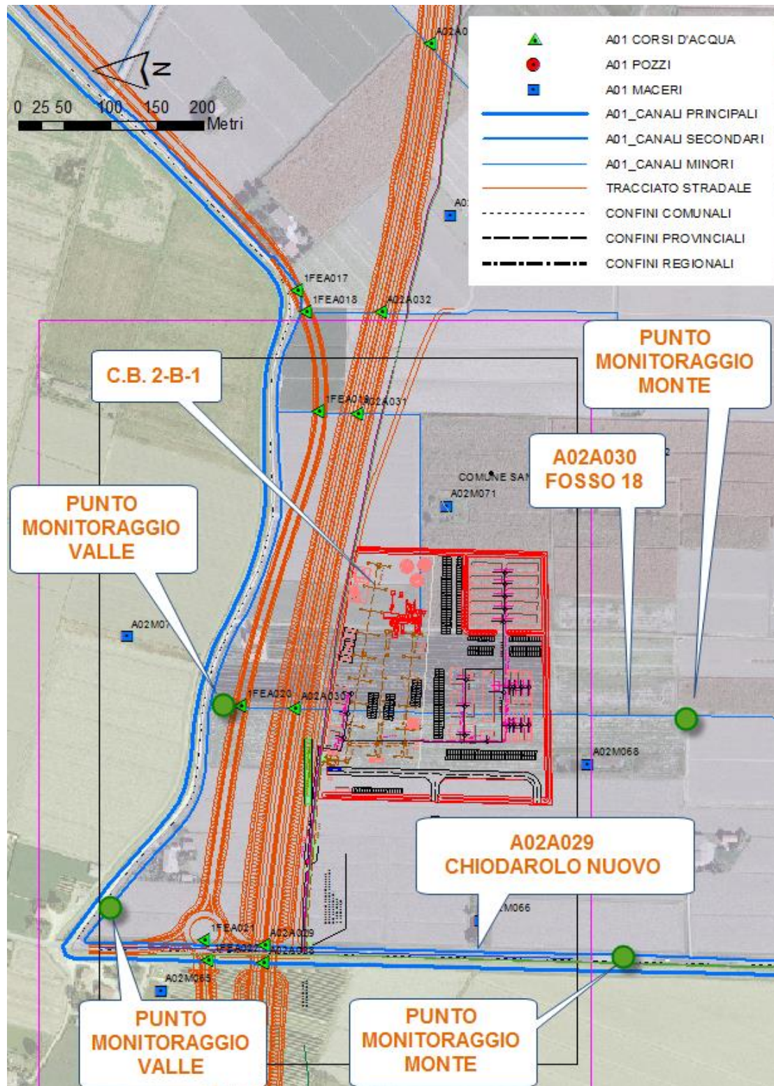
FIGURA 2.4-3 – LOCALIZZAZIONE DEI PUNTI DI MONITORAGGIO AGGIUNTIVI IN PROSSIMITÀ DEL C.B. 2-B.1
