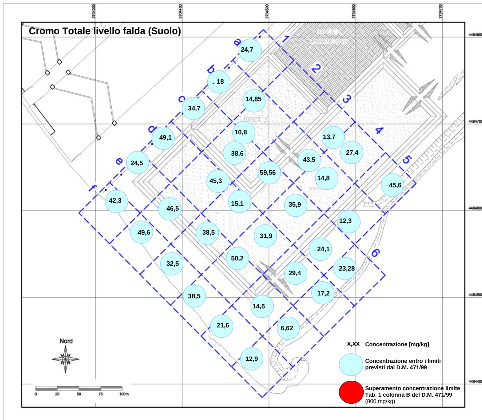
Tav. 3: b) Cromo Totale livello falda (Suolo)
