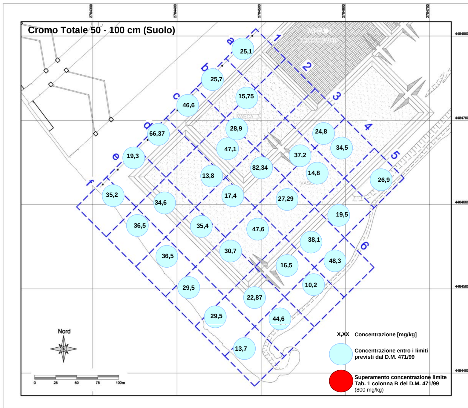
Tav. 3: a) Cromo Totale 50 – 100 cm (Suolo)
