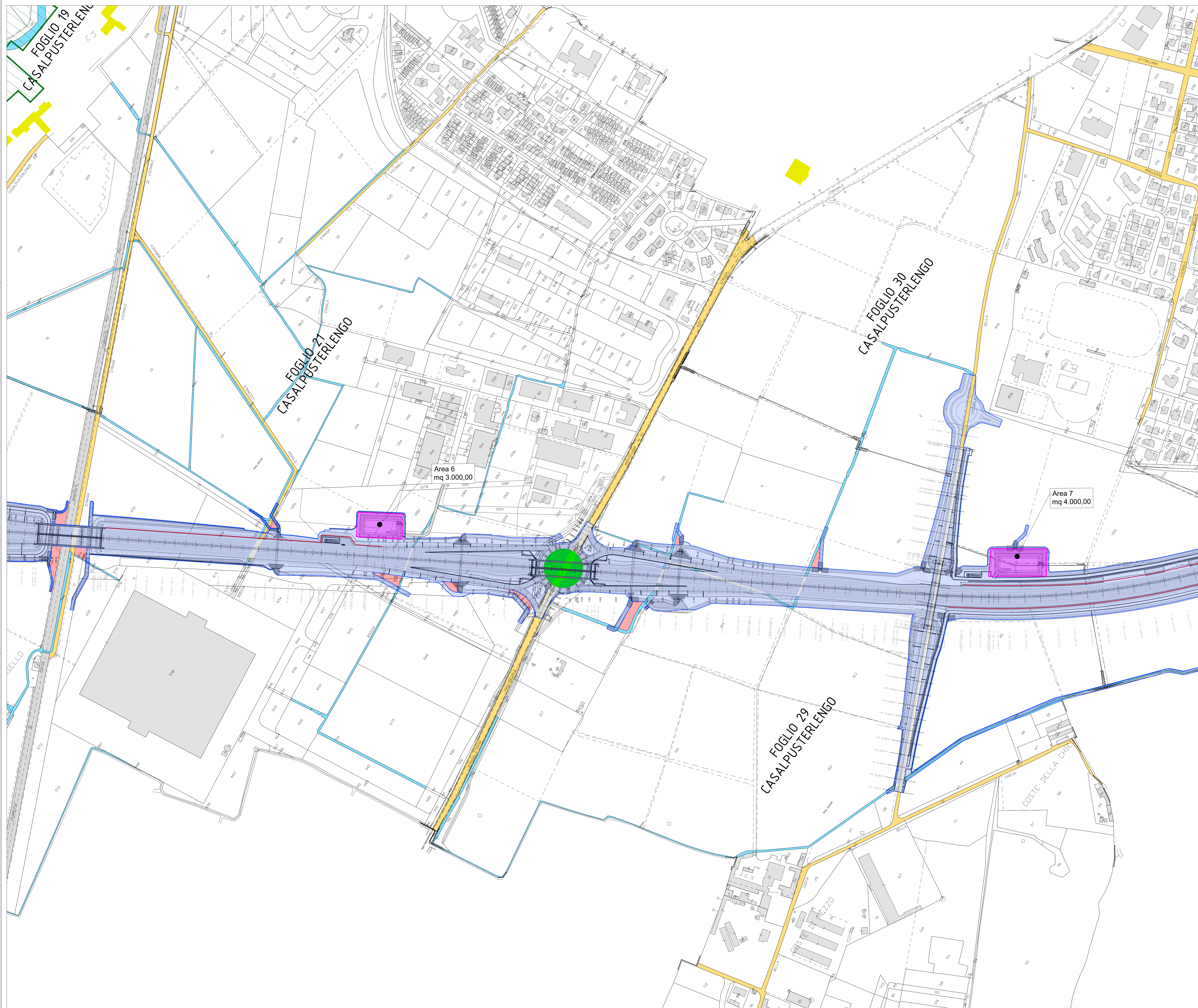
KEY-PLAN
