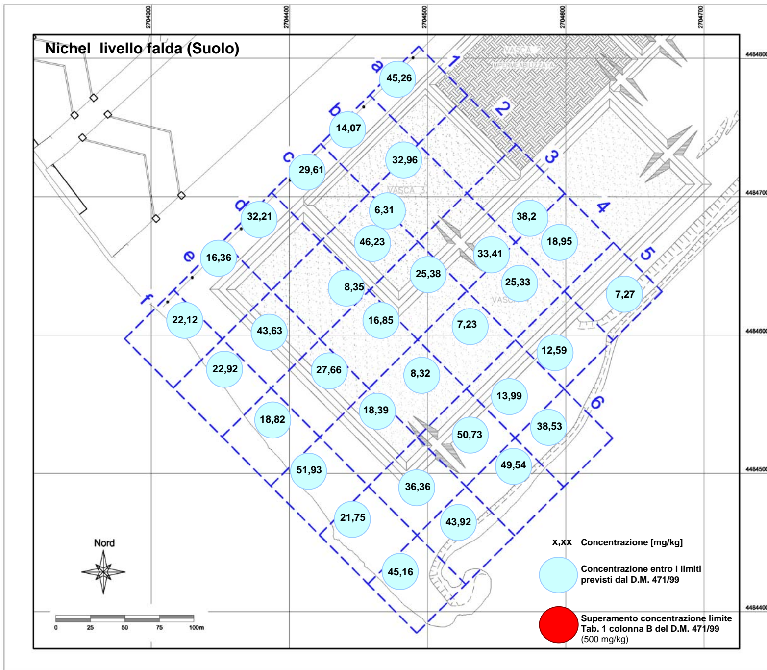
Tav. 6: b) Nichel livello falda (Suolo)
