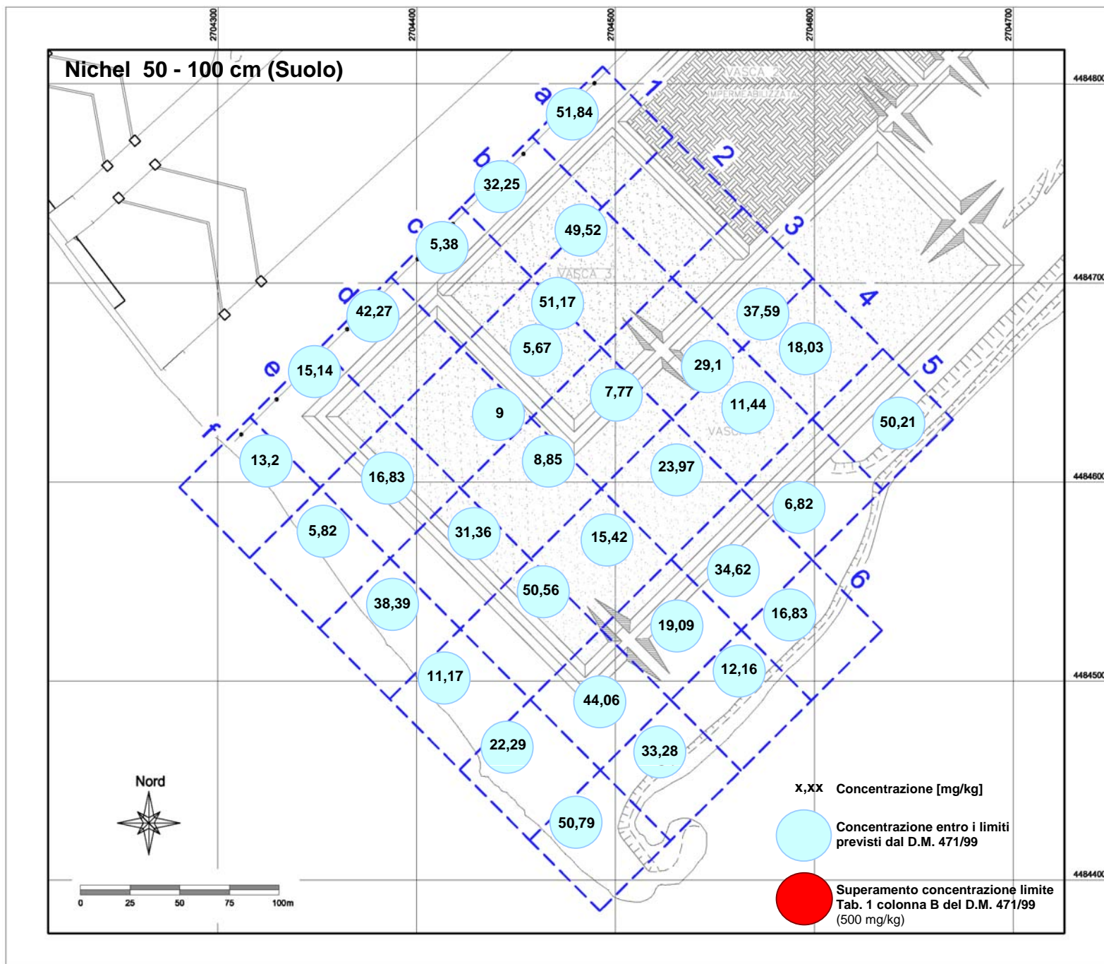
Tav. 6: a) Nichel 50 – 100 cm (Suolo)
