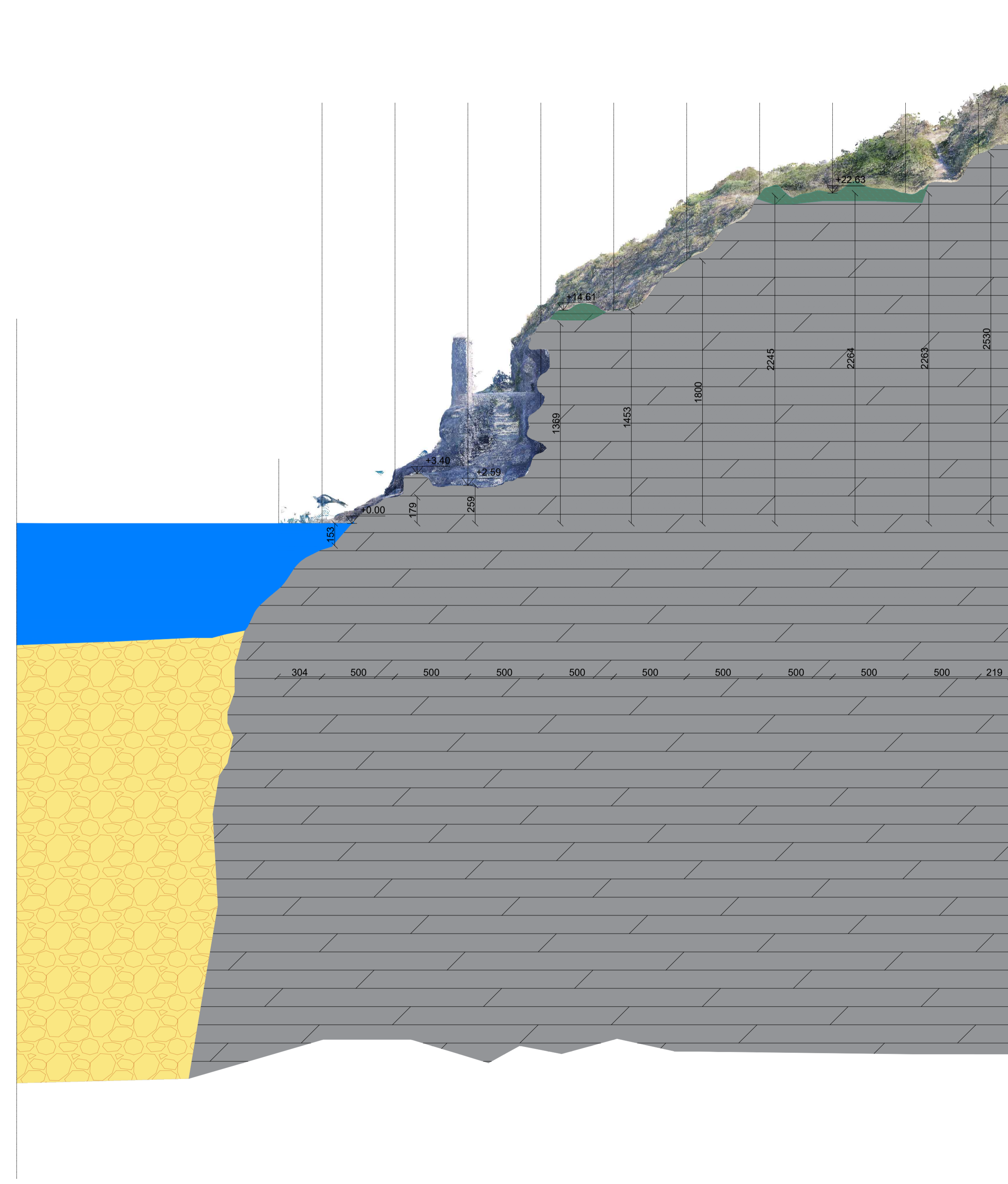
SEZIONE C-C', scala 1:200
