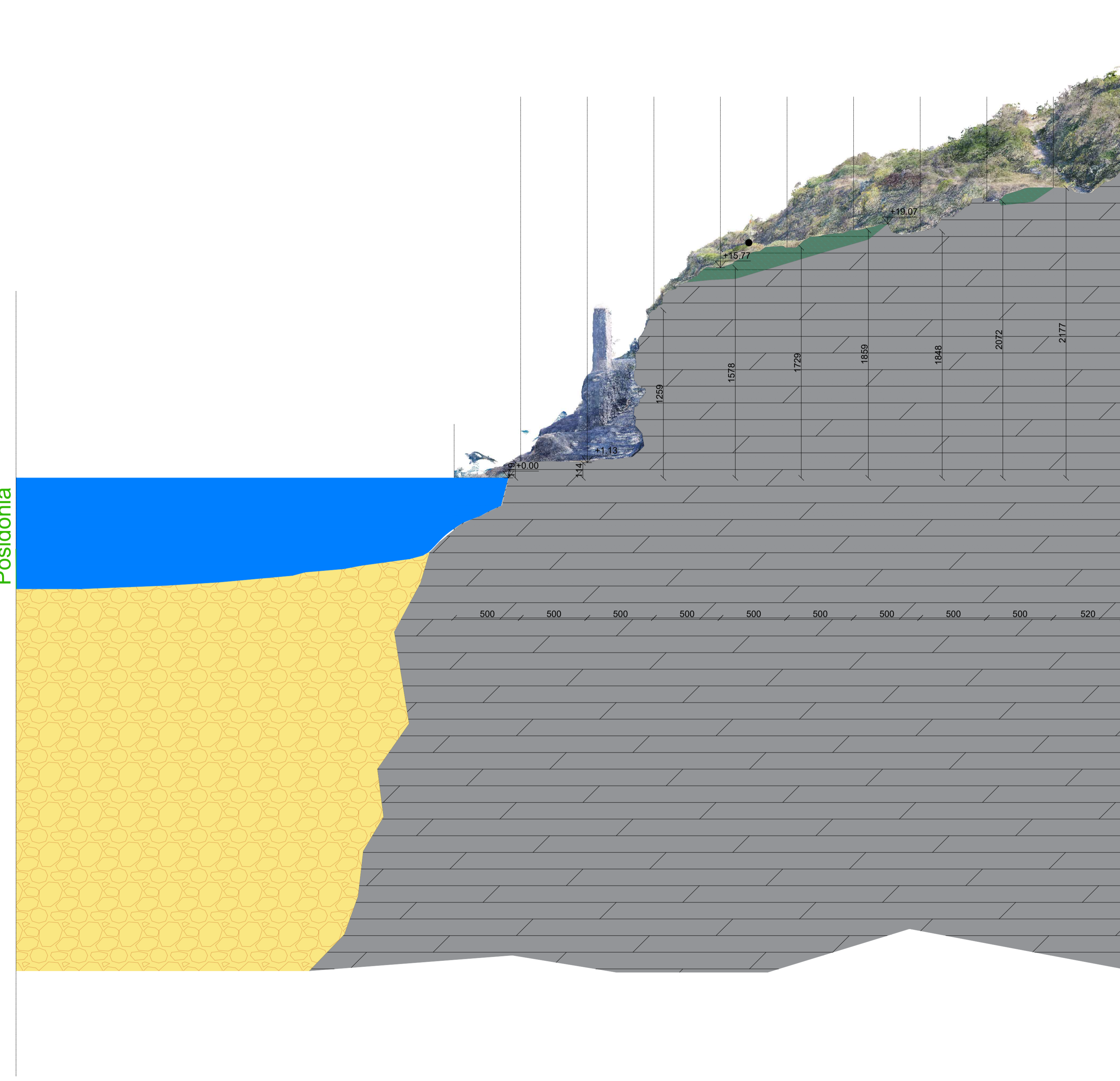
SEZIONE A-A', scala 1:200
