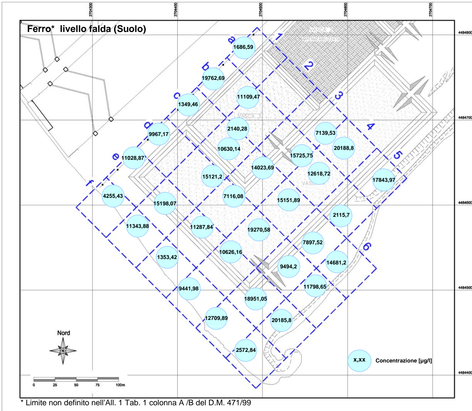
Tav. 10: b) Ferro livello falda (Suolo)
