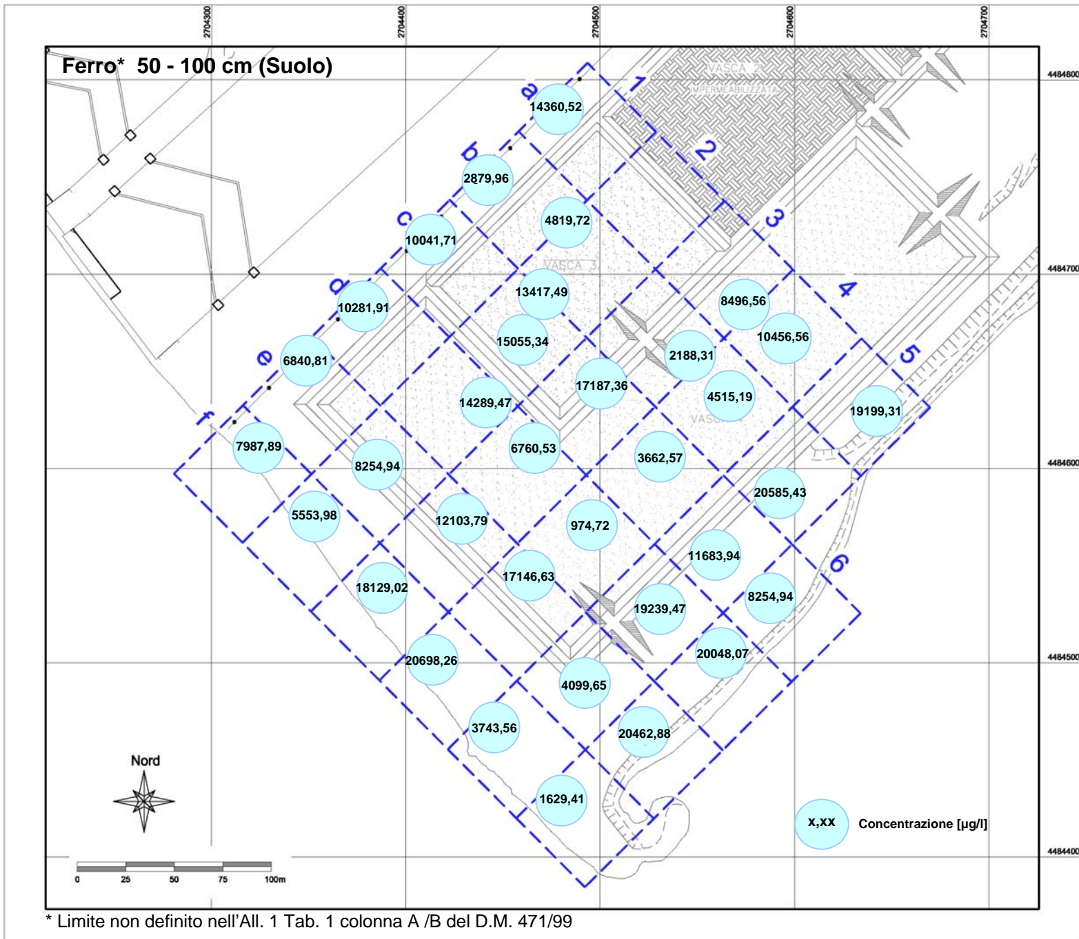
Tav. 10: a) Ferro 50 – 100 cm (Suolo)
