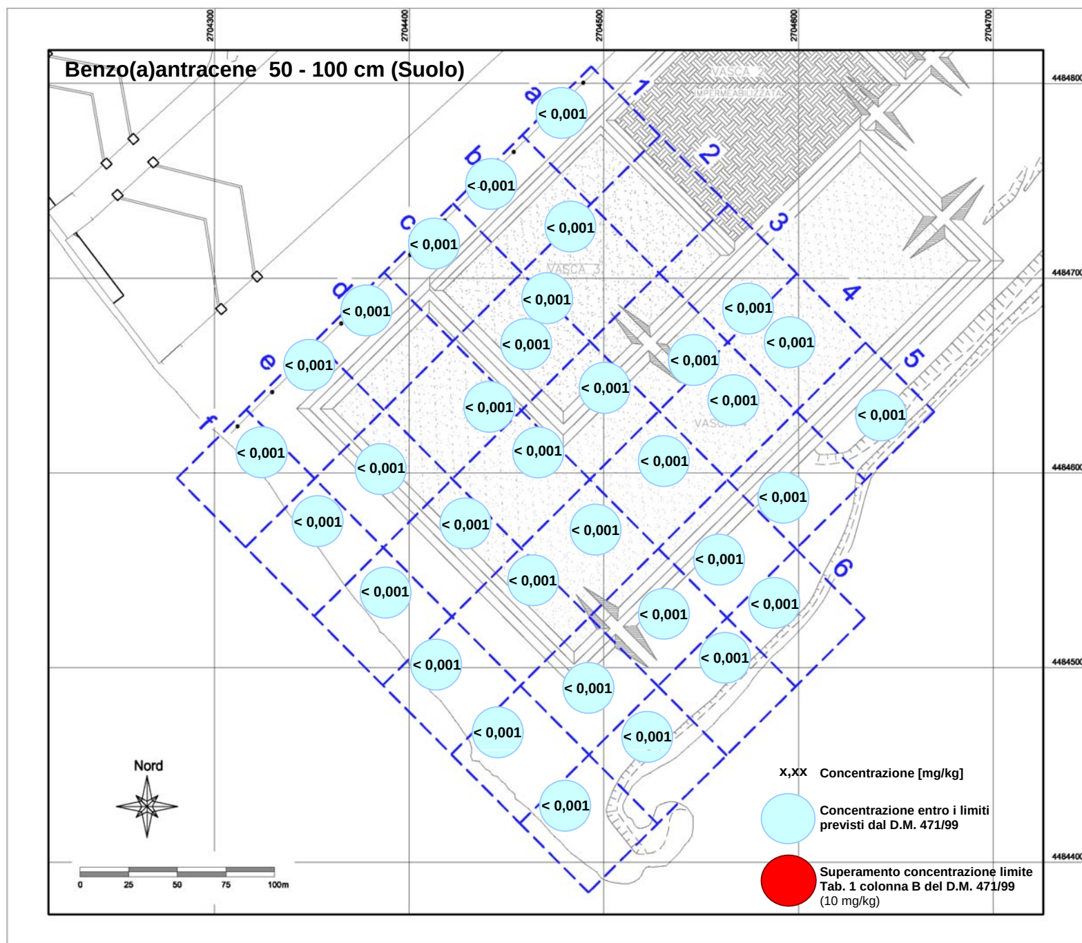
Tav. 12: a) Benzo(a)antracene 50 – 100 cm (Suolo)
