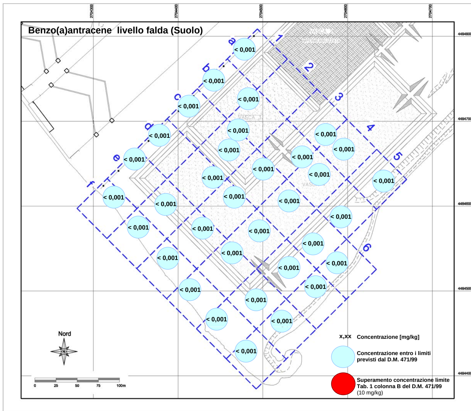
Tav. 12: b) Benzo(a)antracene livello falda (Suolo)
