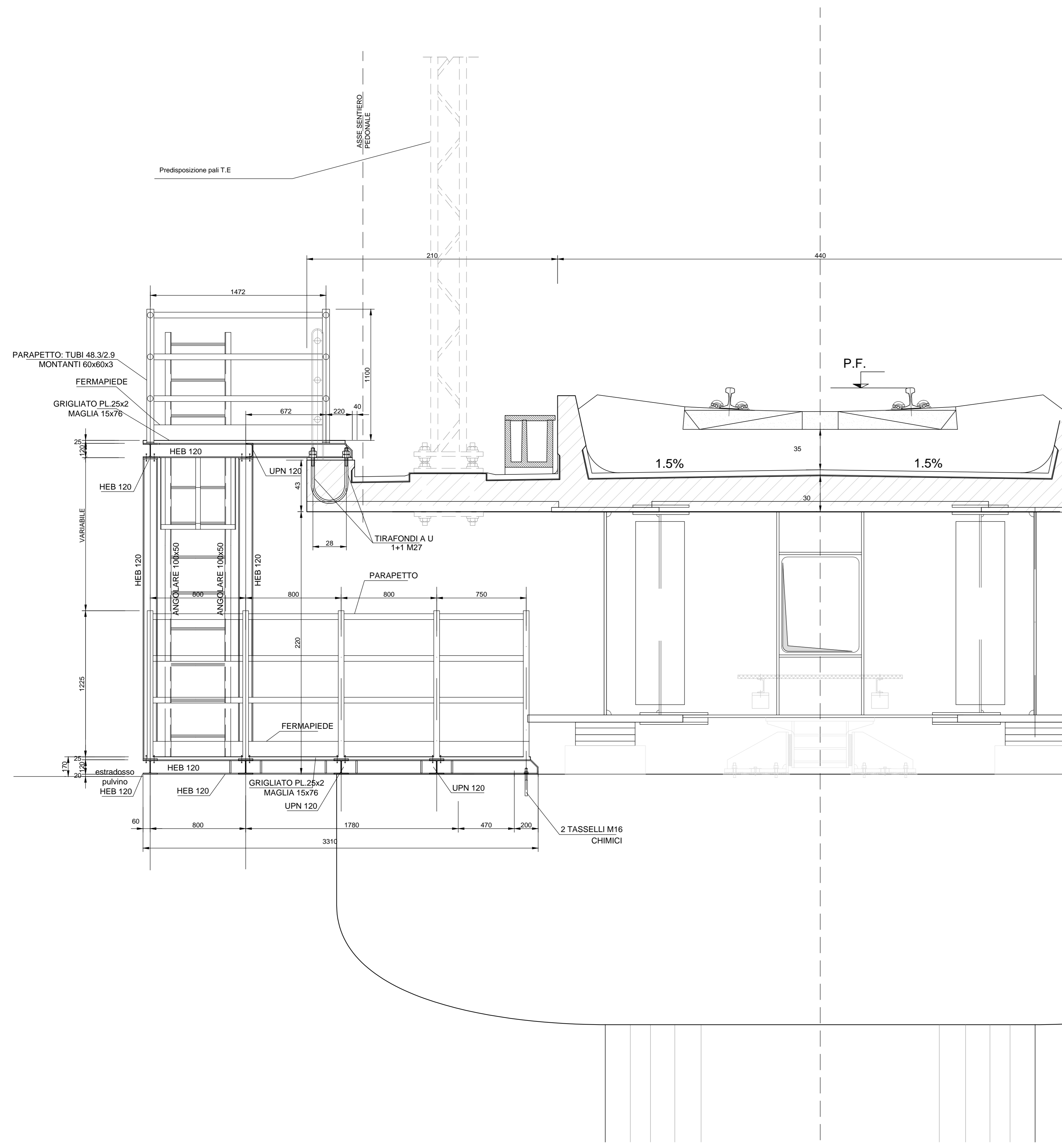
SEZIONE B-B SCALA 1:20
