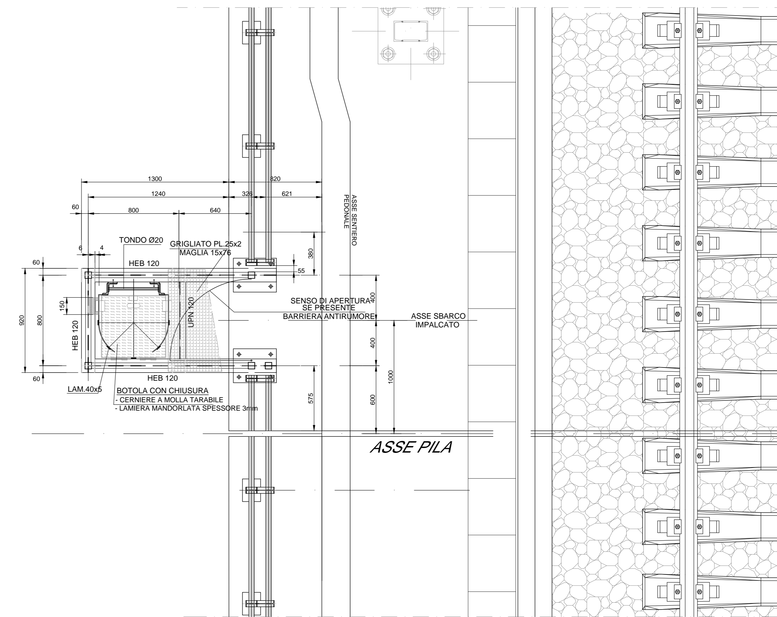
PIANTA SCALA 1:20
