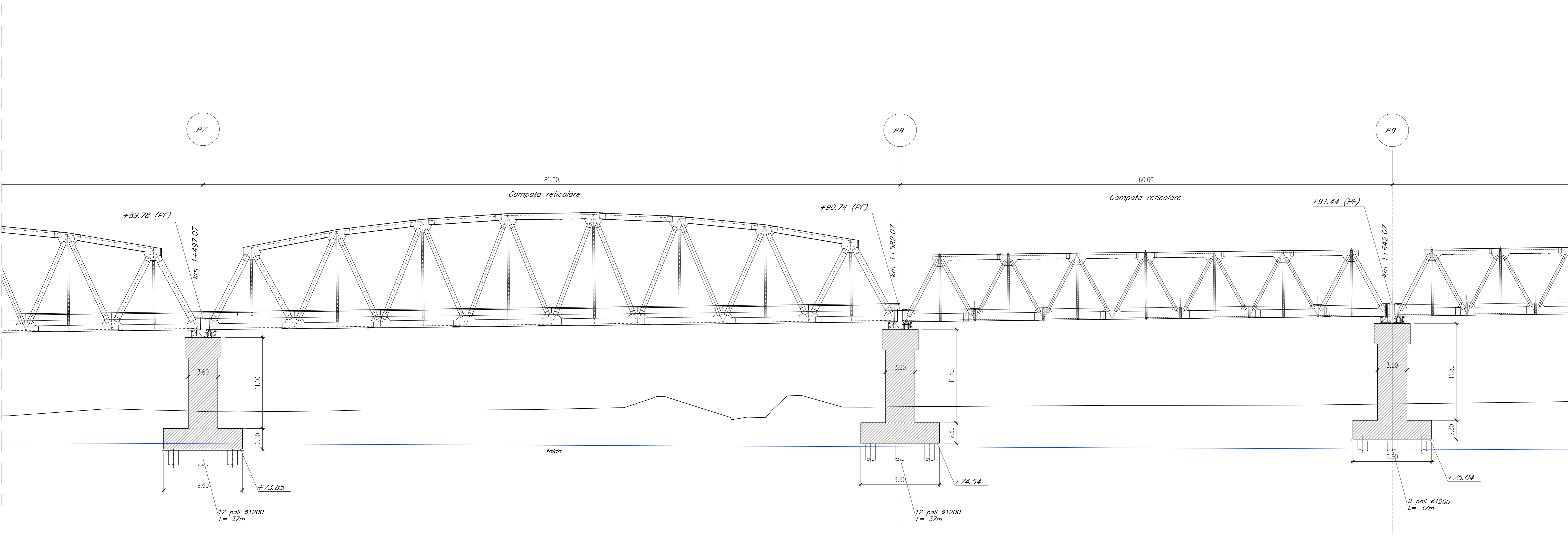
SEZIONE LONGITUDINALE Scala 1:200
