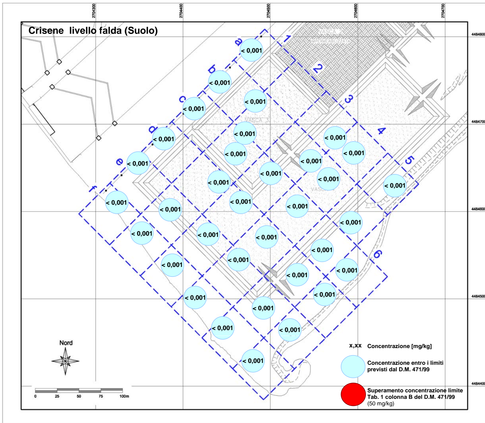
Tav. 17: b) Crisene livello falda (Suolo)
