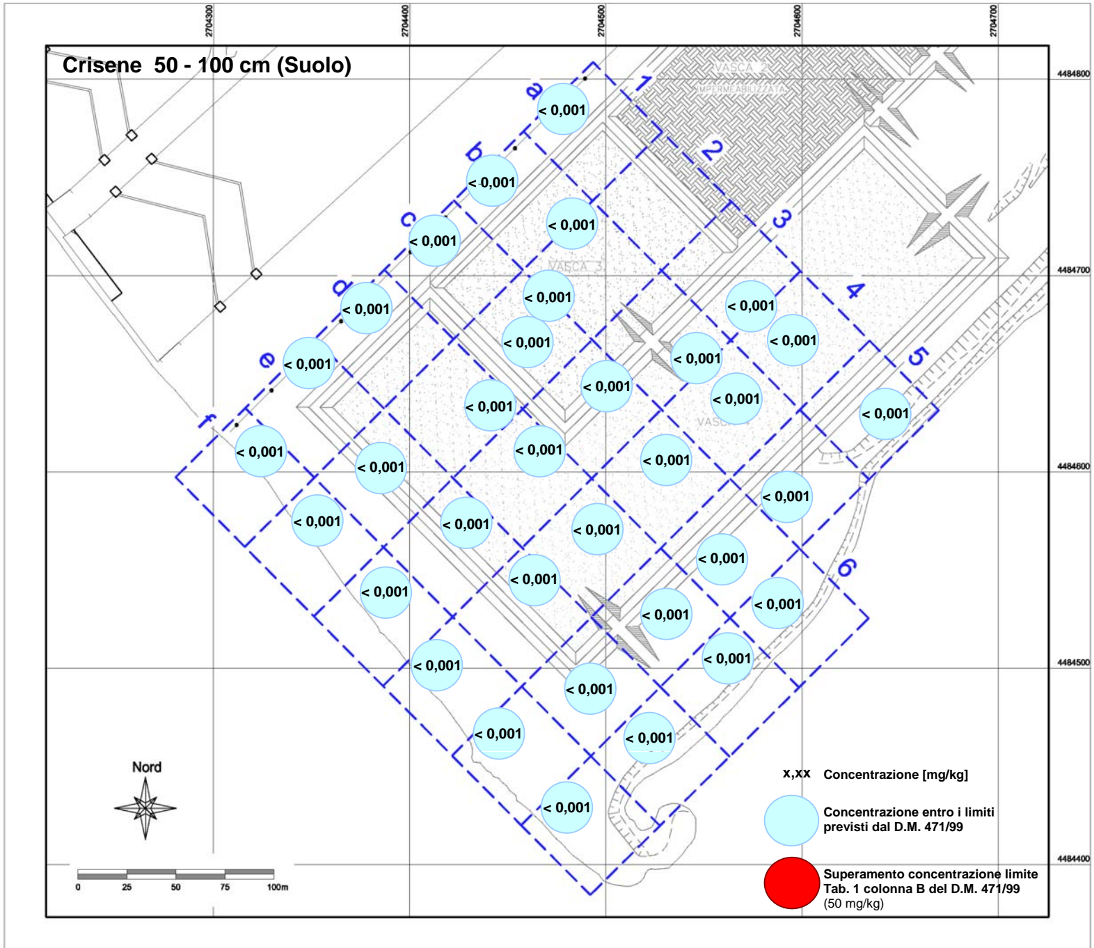
Tav.17: a) Crisene 50 – 100 cm (Suolo)
