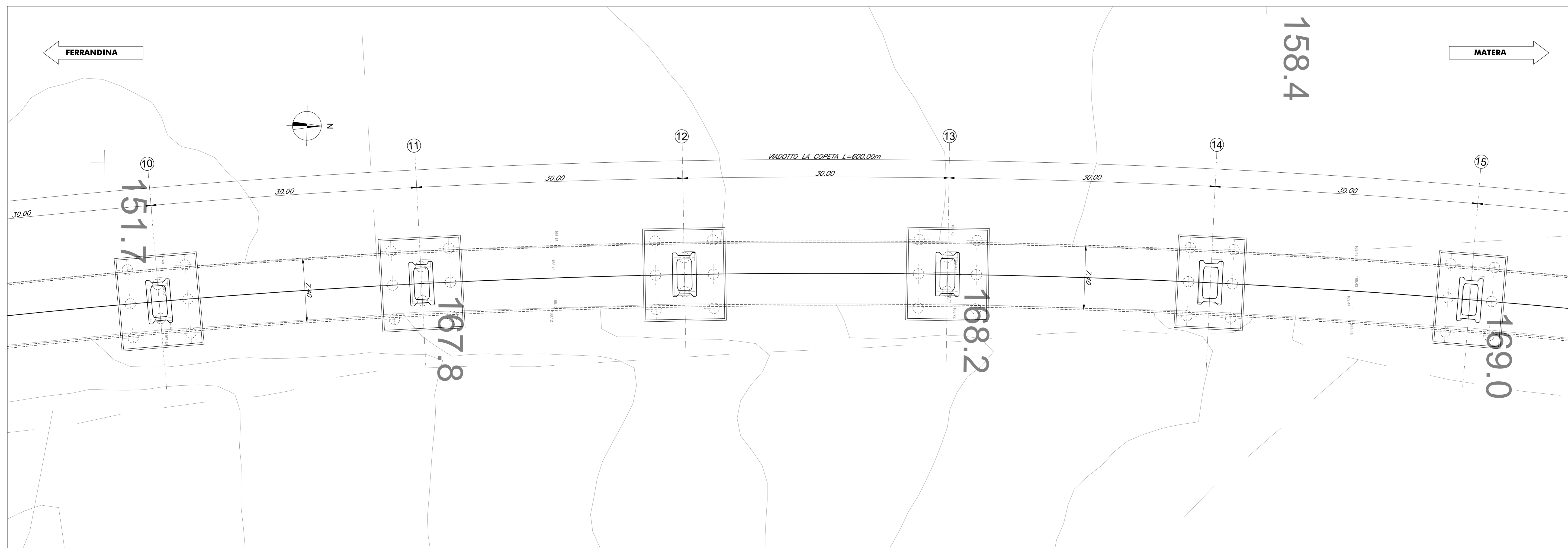
PIANTA scala 1:200
