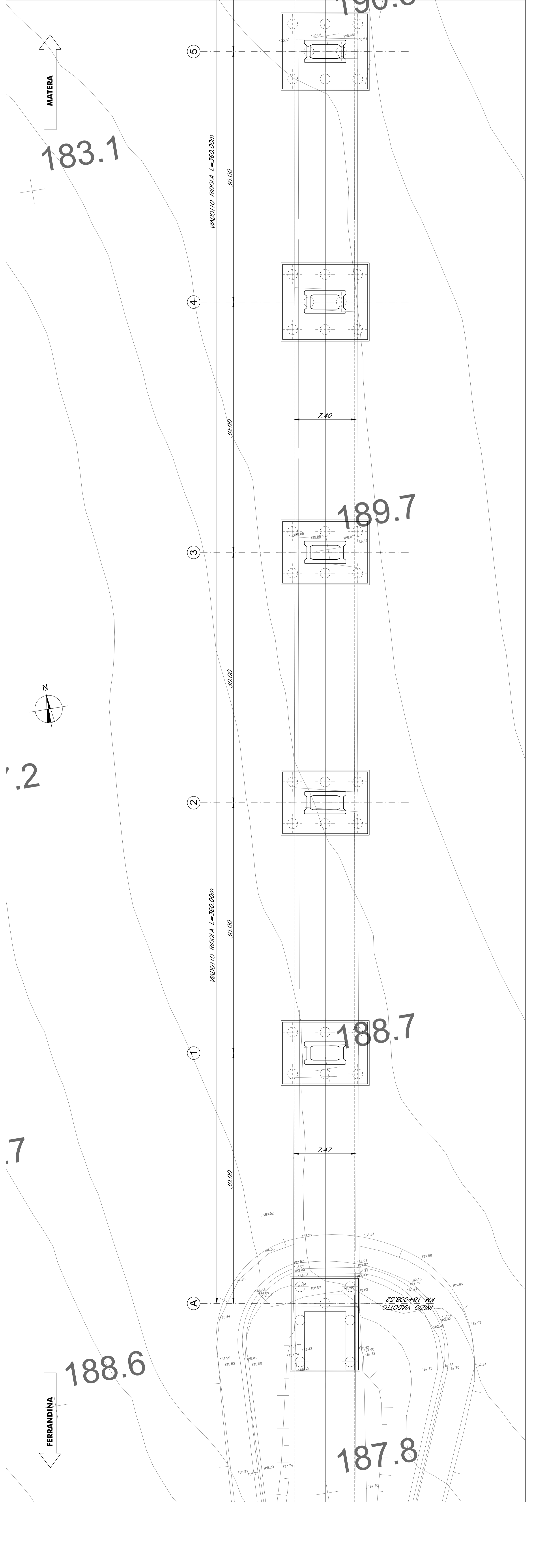
PIANTA scala 1:200
