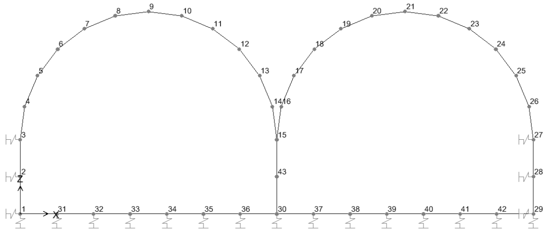
Figura 2.2: Vista frontale del modello di calcolo della galleria
