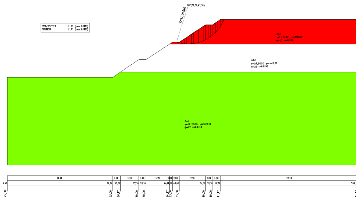
Figura 3.3: Cerchio di rottura in termini di tensioni efficaci
