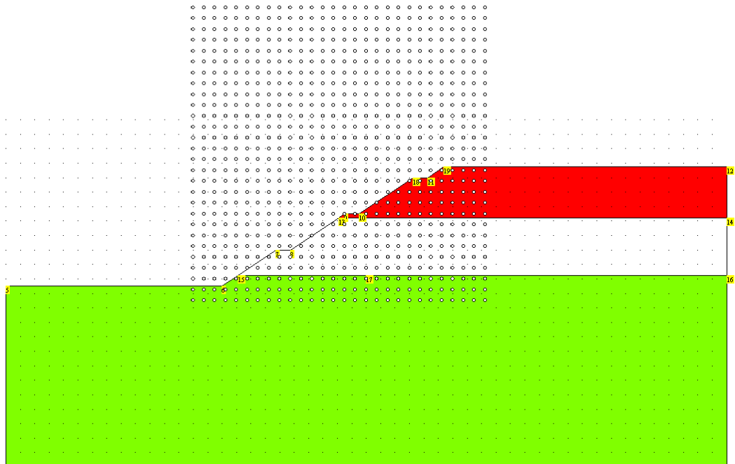
Figura 3.2: Mappa dei centri delle superfici di rottura
