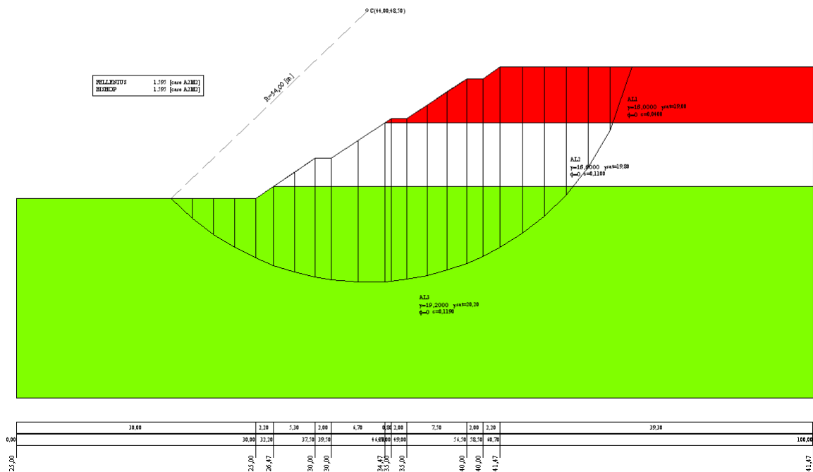
Figura 3.4: Cerchio di rottura in termini di tensioni totali
