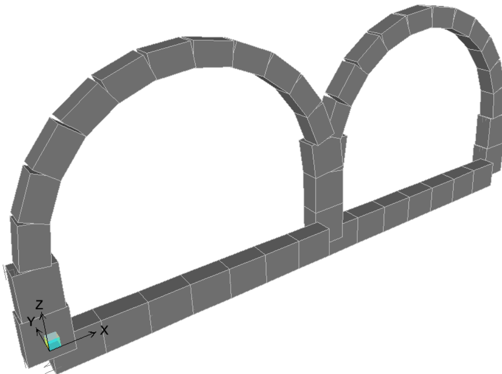
Figura 2.1: Vista 3D del modello di calcolo della galleria
