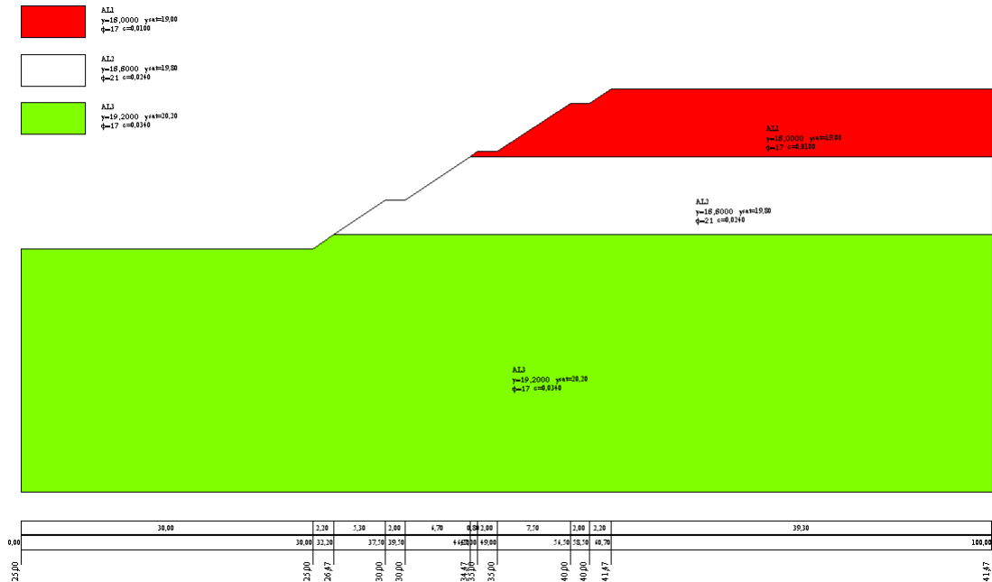
Figura 3.1: Schematizzazione del pendio
