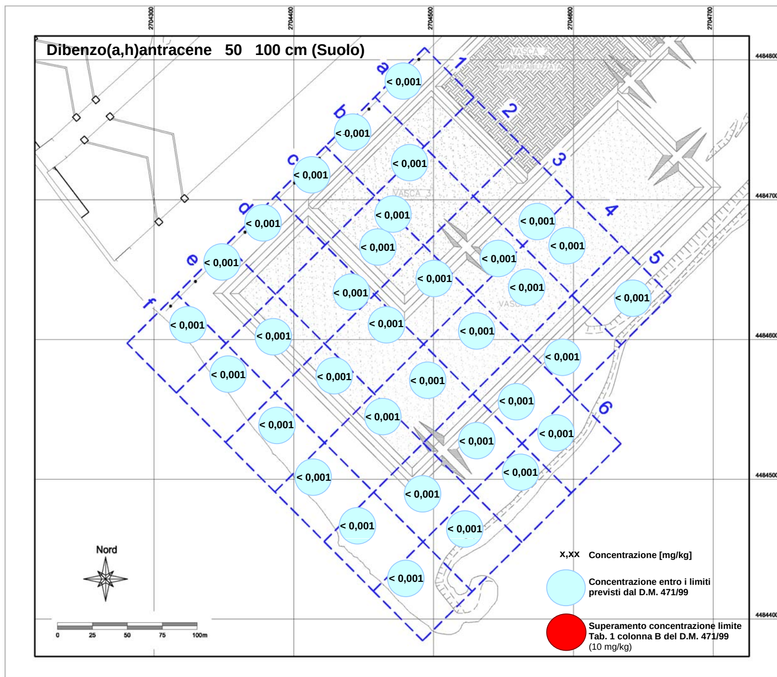
Tav.19: a) Dibenzo(ah)antracene 50 – 100 cm (Suolo)
