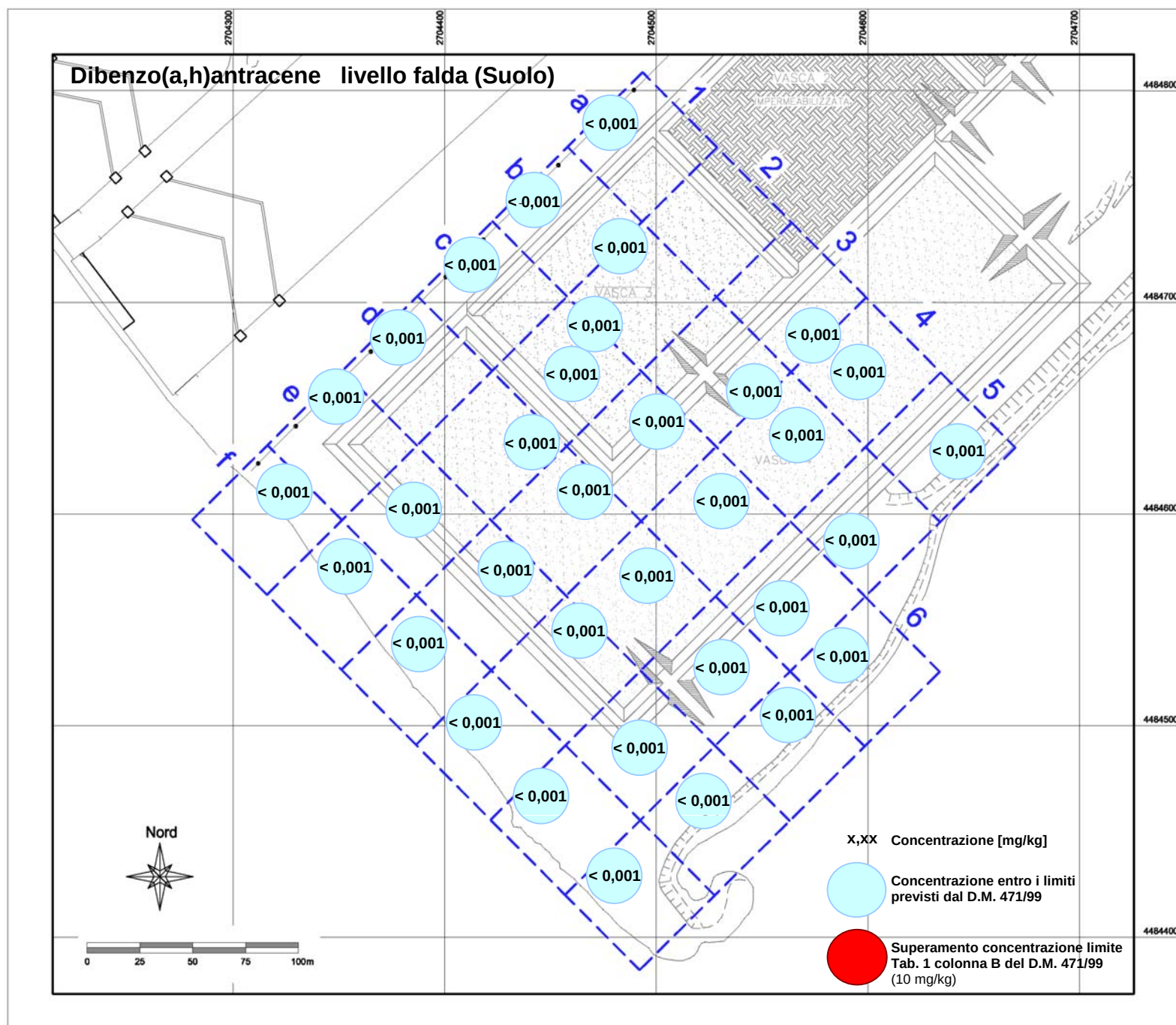
Tav. 19: b) Dibenzo(ah)antracene livello falda (Suolo)
