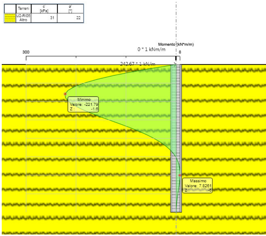
Figura 7 – Momento agente in condizione SLV
