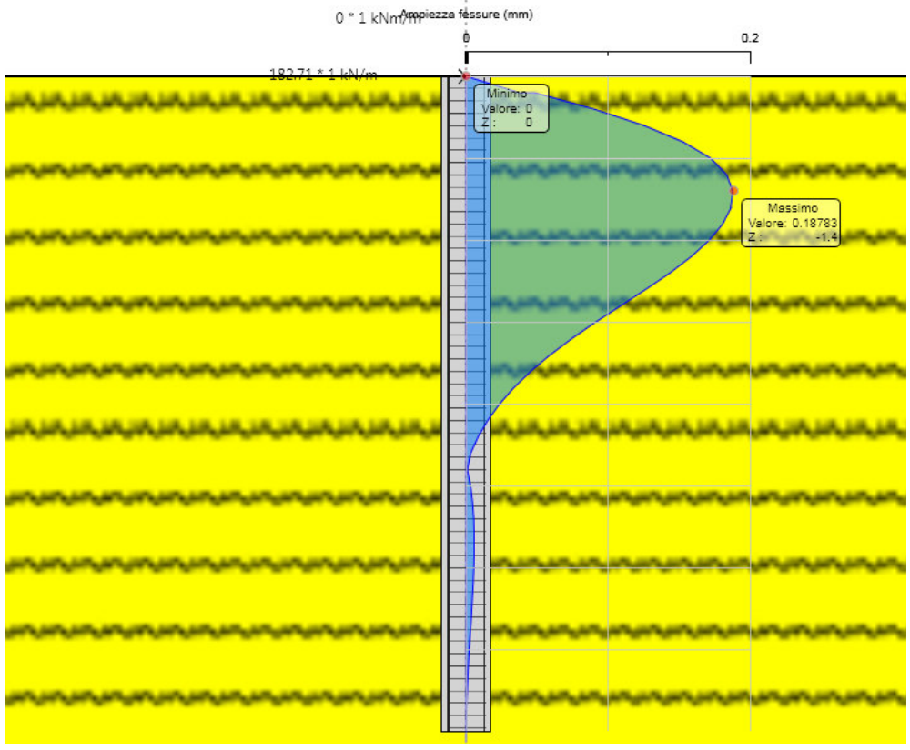
Figura 11 – Verifica a fessurazione SLE, l'ampiezza massima <0.2 mm, verifica soddisfatta.
