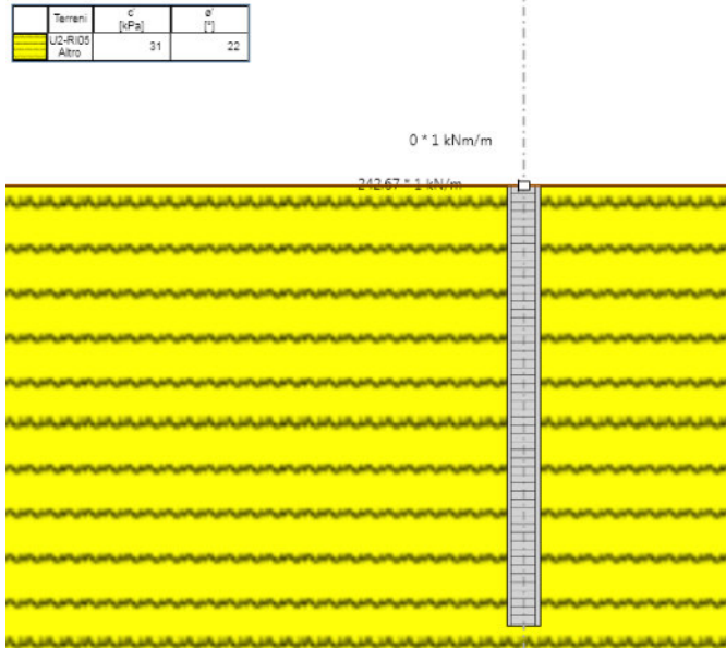
Figura 3 – Carico agente in condizione SLV
