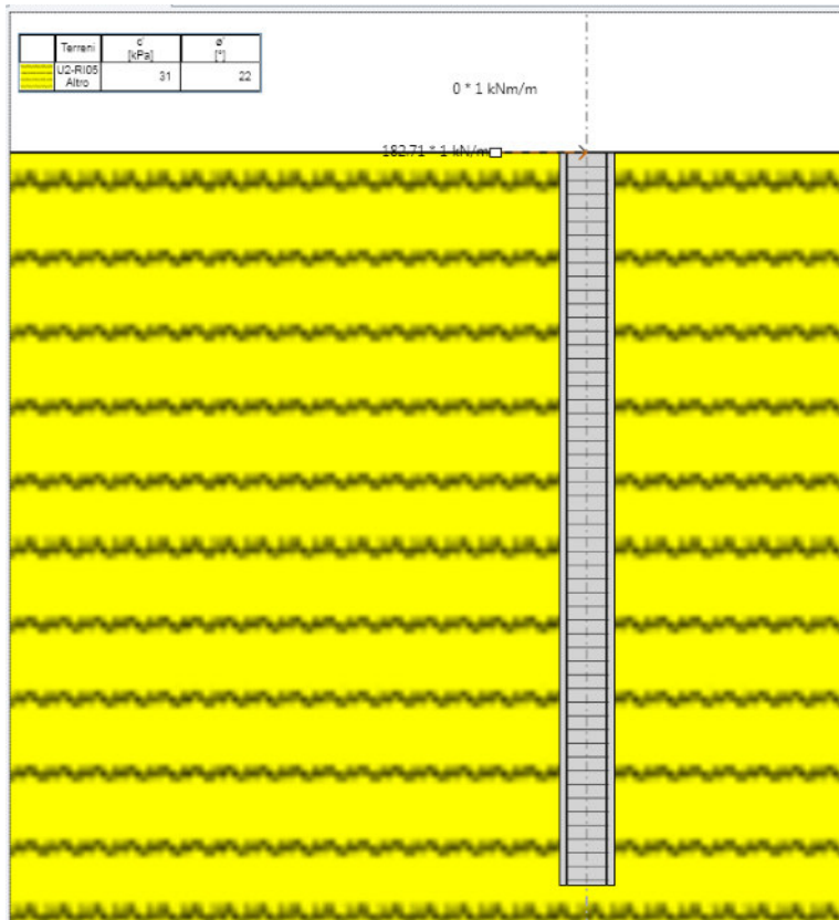
Figura 1 – Carico agente in condizione SLE
