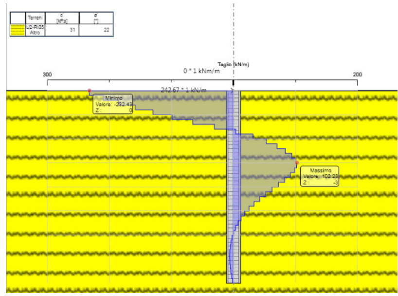
Figura 8 – Taglio agente in condizione SLV
