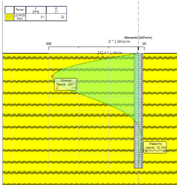
Figura 5 – Momento agente in condizione SLU
