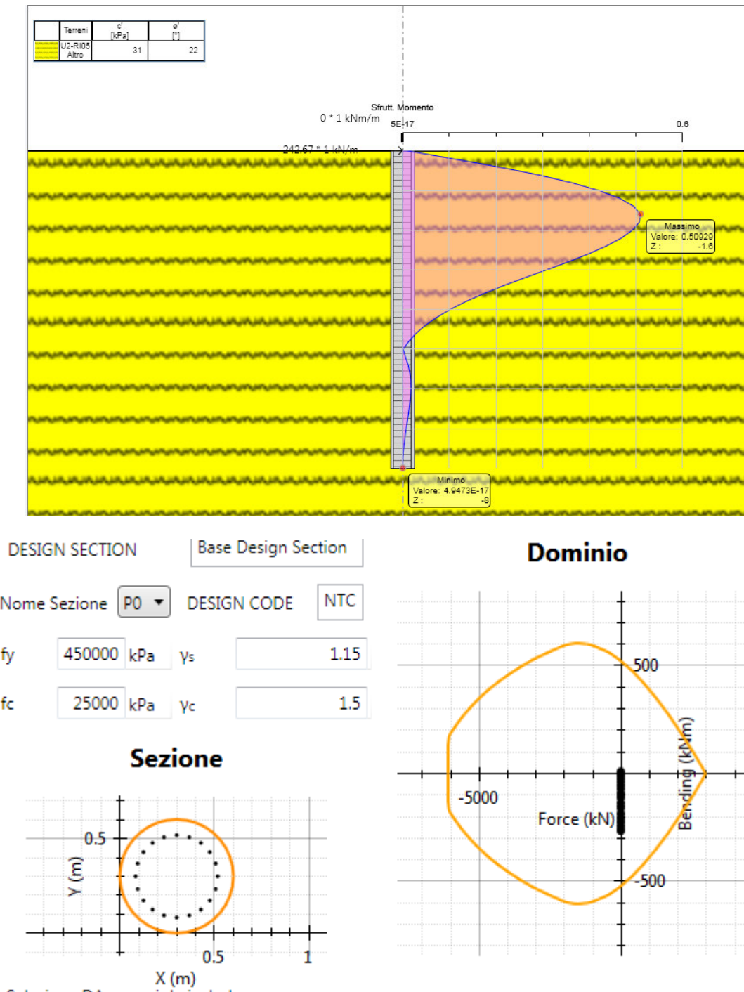
Figura 10 – Verifica a pressoflessione SLV.
