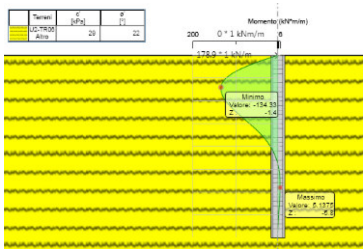
Figura 4 – Memento agente in condizione SLE
