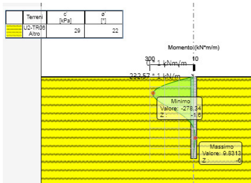
Figura 5 – Memento agente in condizione SLU
