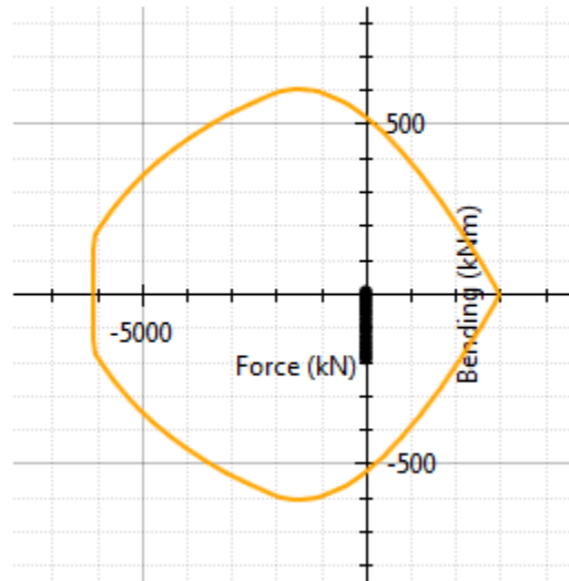
Figura 9 – Verifica a pressoflessione SLU.
