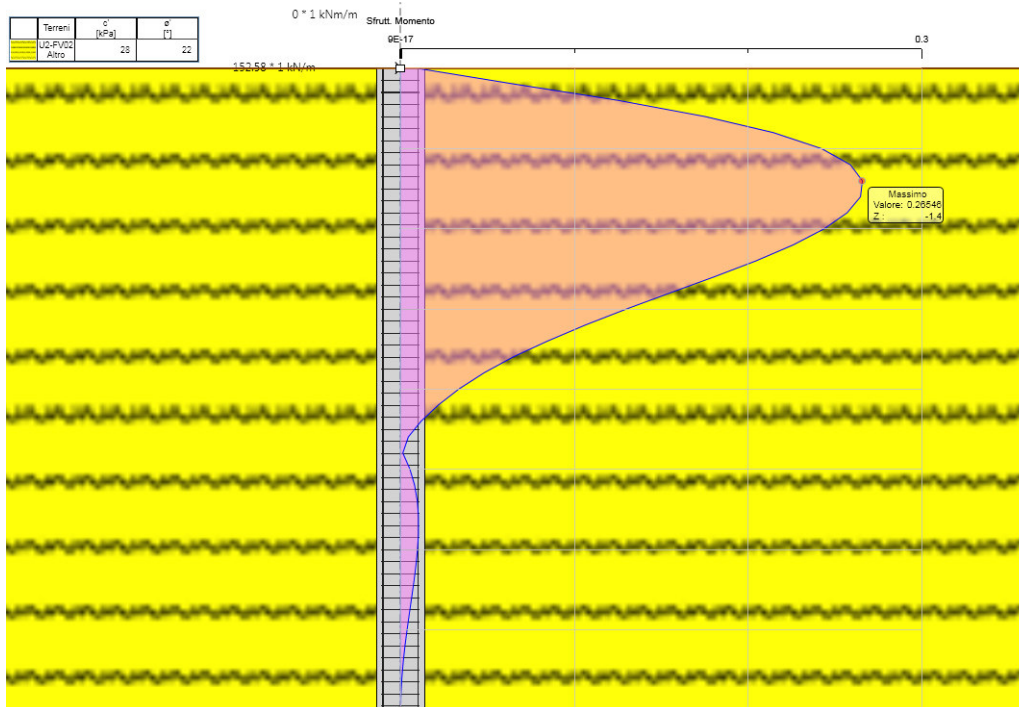
Figura 9 – Verifica a pressoflessione SLU.
