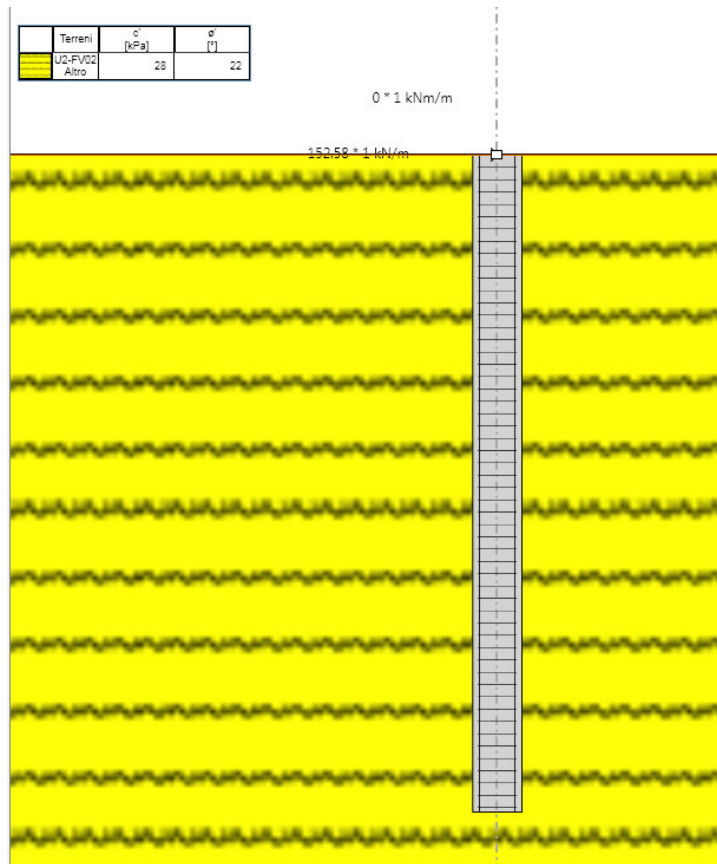
Figura 3 – Carico agente in condizione SLV
