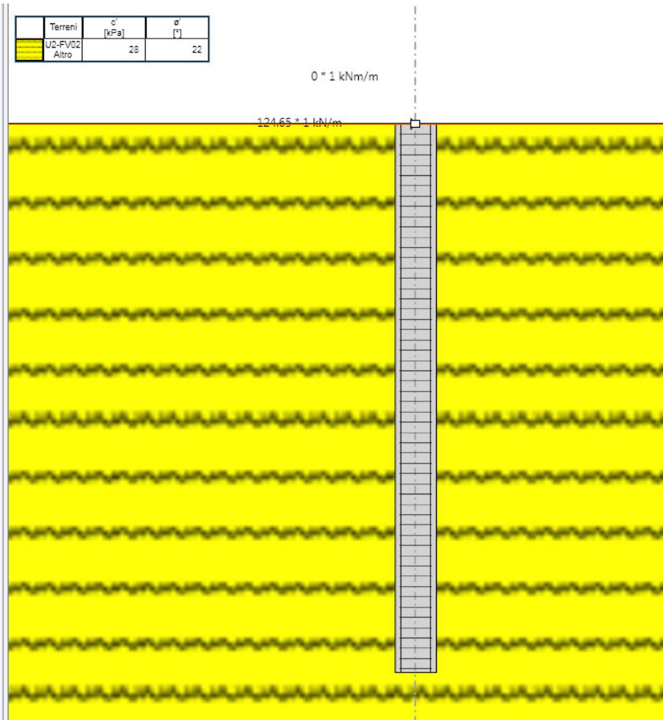
Figura 1 – Carico agente in condizione SLE
