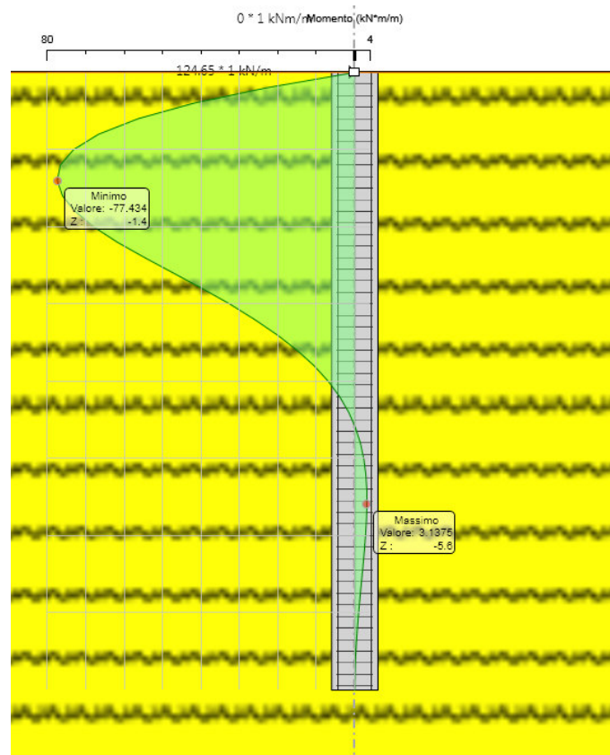
Figura 4 – Momento agente in condizione SLE
