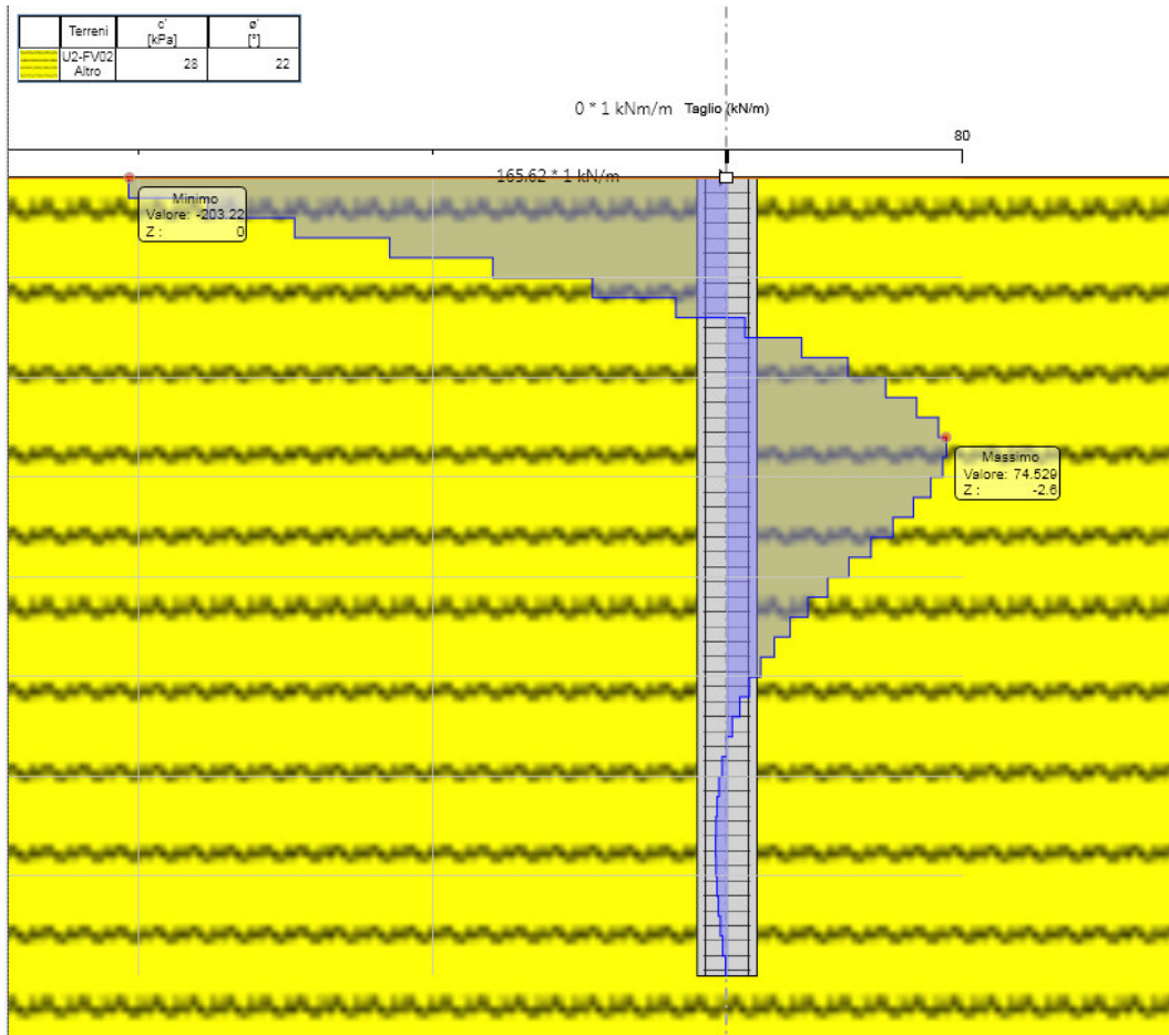
Figura 6 – Taglio agente in condizione SLU
