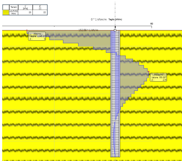
Figura 8 – Taglio agente in condizione SLV
