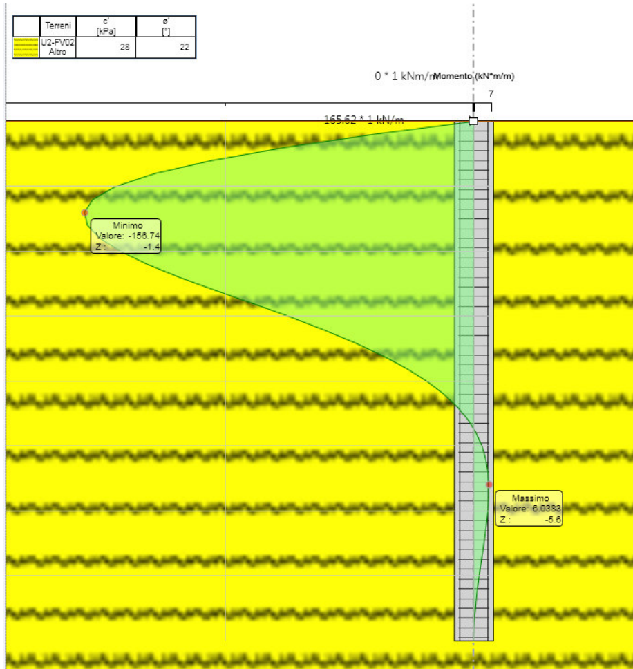
Figura 5 – Momento agente in condizione SLU
