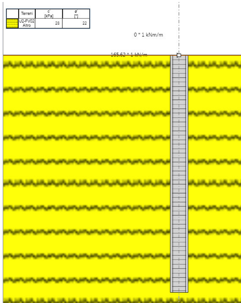
Figura 2 – Carico agente in condizione SLU
