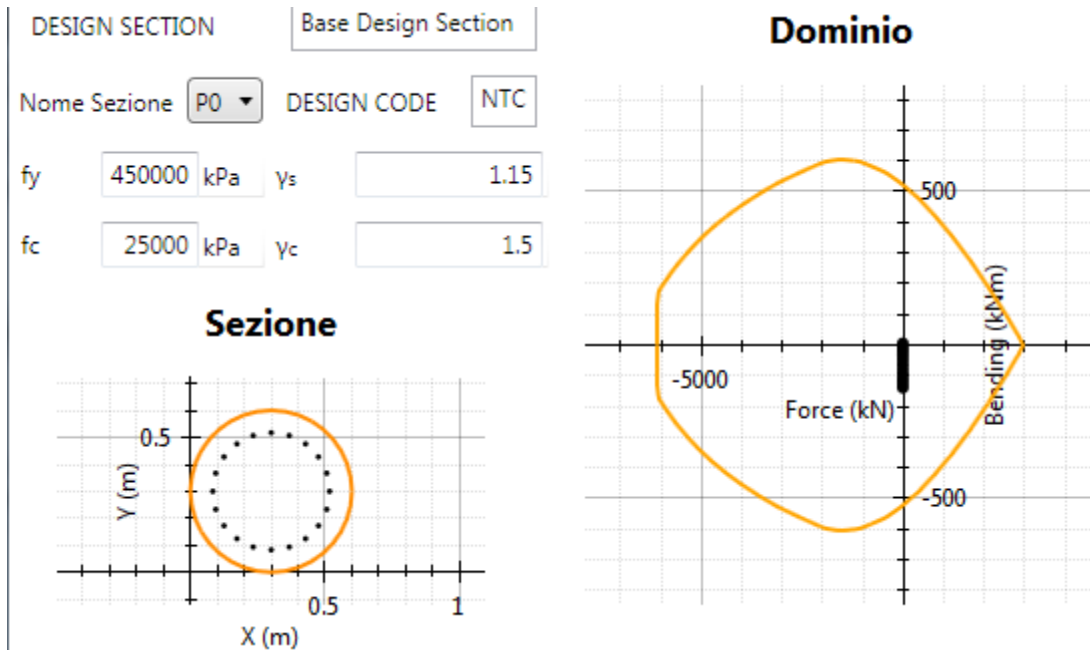
Figura 10 – Verifica a pressoflessione SLV.
