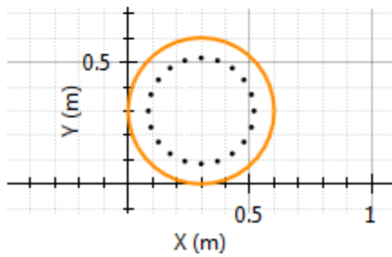
Figura 9 – Verifica a pressoflessione SLU.
