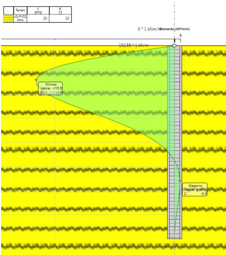
Figura 7 – Momento agente in condizione SLV
