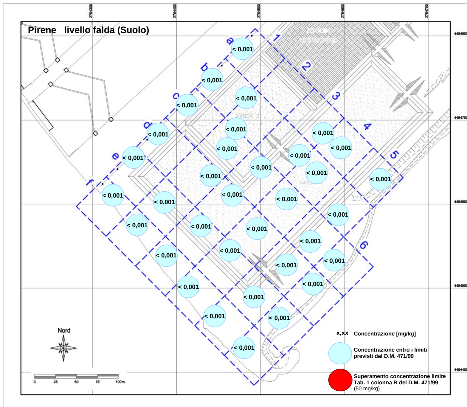
Tav. 21: b) Pirene livello falda (Suolo)
