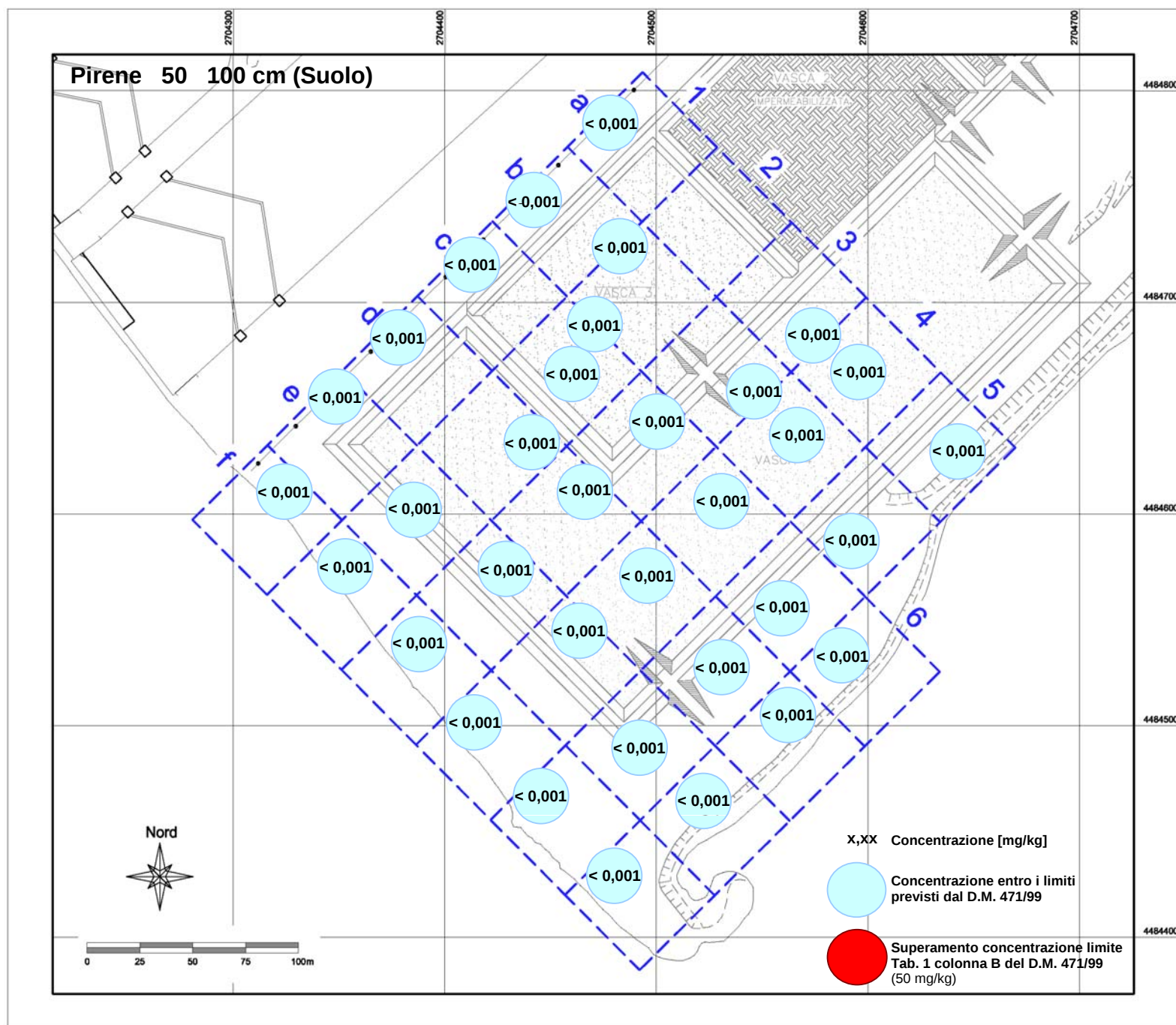
Tav.21: a) Pirene 50 – 100 cm (Suolo)
