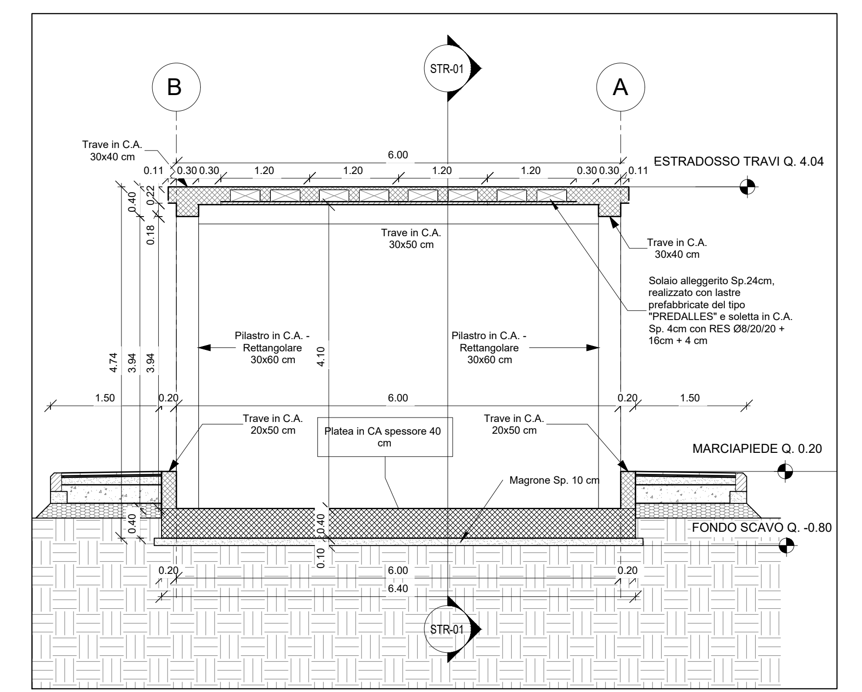
Sezione Trasversale STR-2 1 : 50
