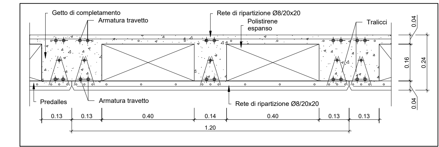
Dettaglio Solai Copertura 1 : 10
