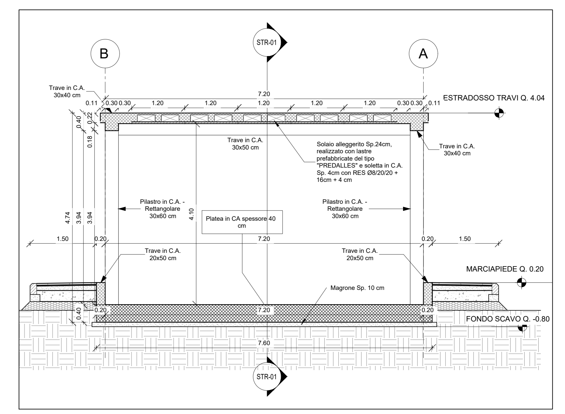
Sezione Trasversale STR-2
