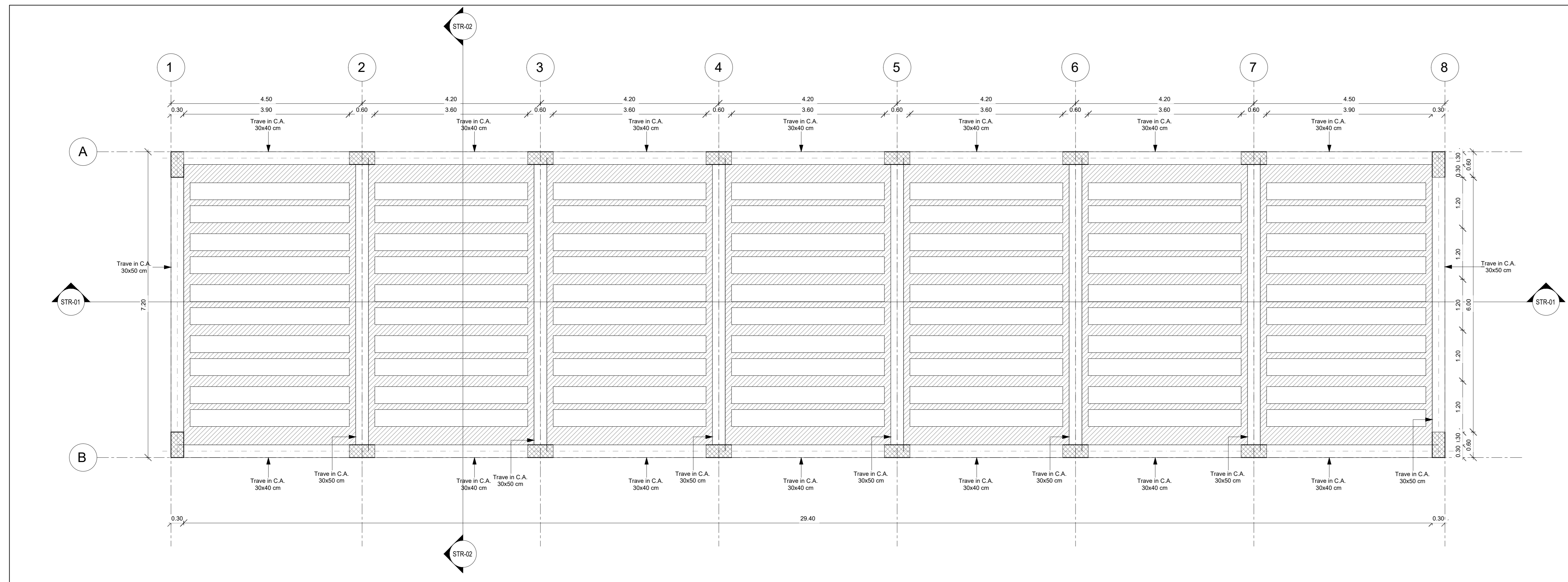
Pianta Copertura
