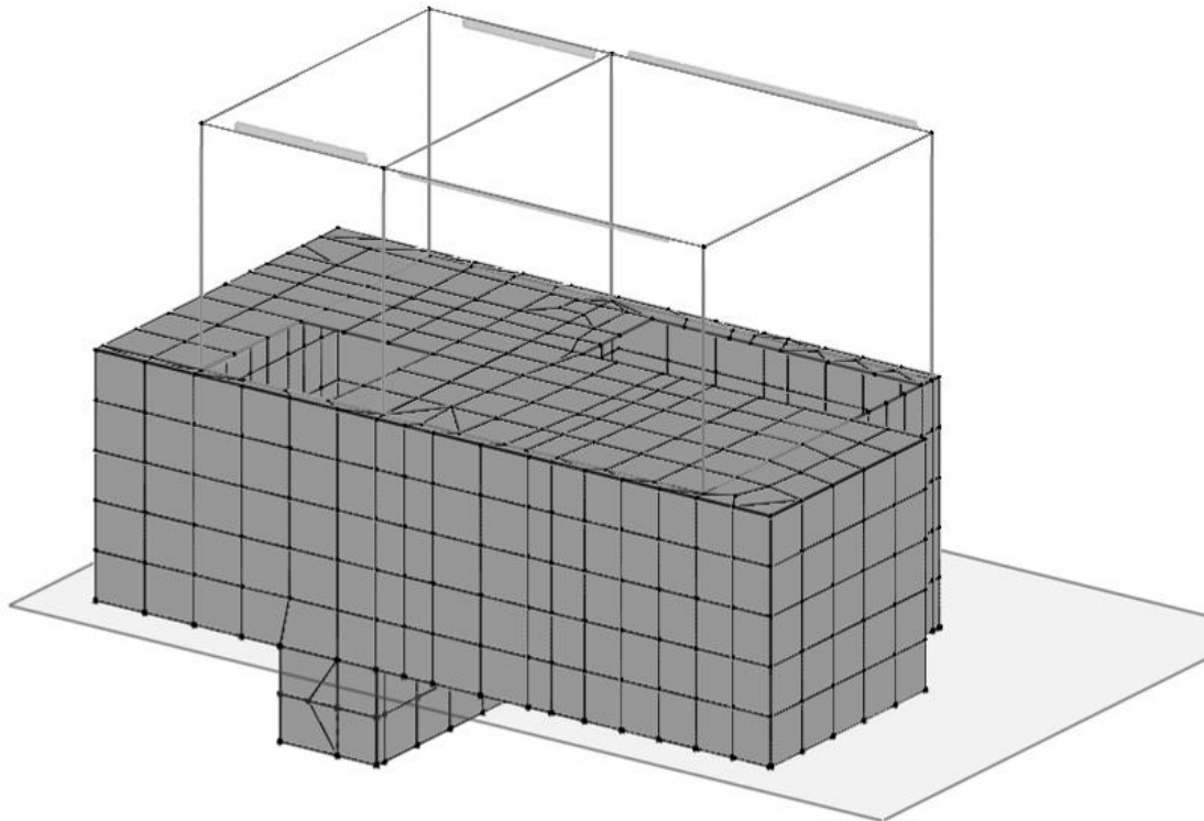
Figura 7.1-7 Diagramma della torsione T – COMB_INV_SLU.
