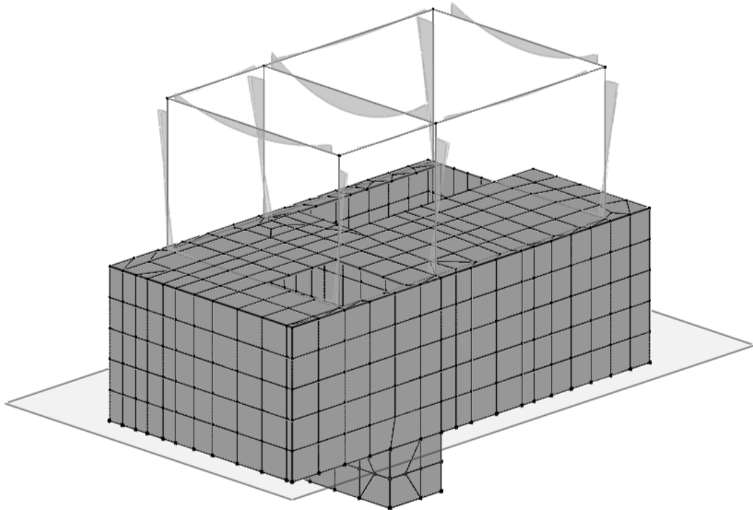
Figura 7.1-2 Diagramma dei momenti M3 – COMB_INV_SLV.
