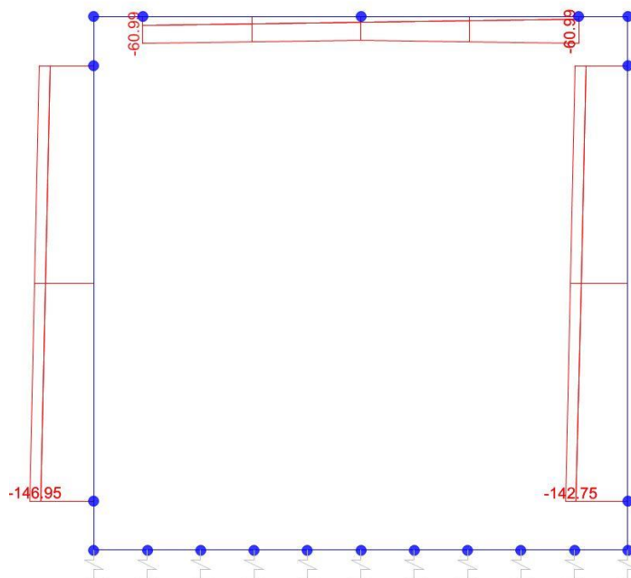
Sforzo normale
