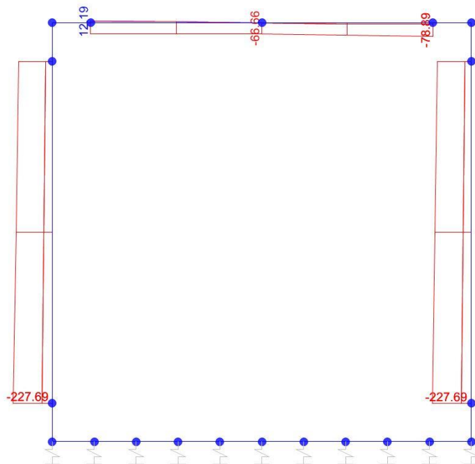
Sforzo normale
