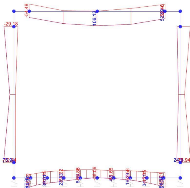
Momento Flettente
