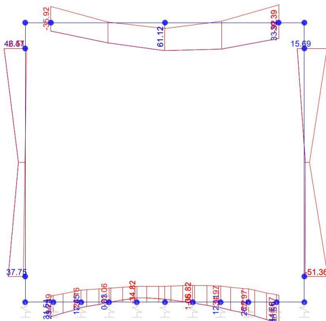
Momento Flettente
