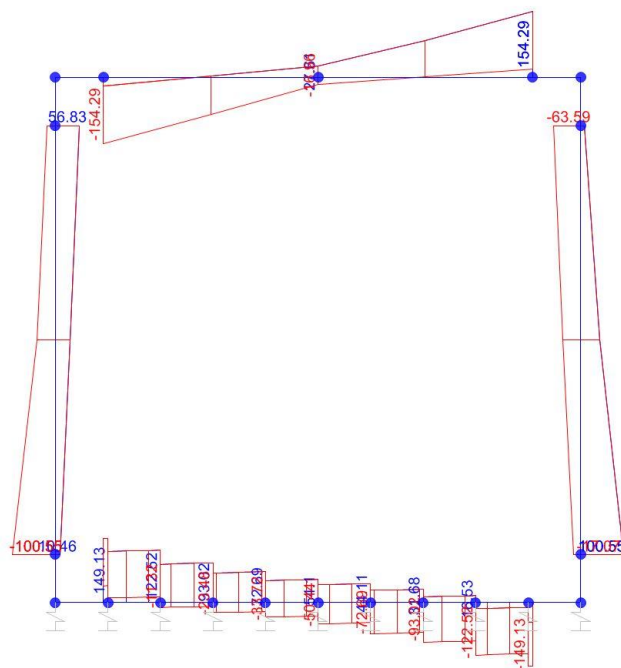
Taglio
