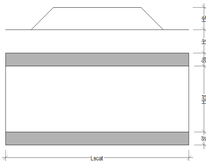
Figura 1. Sezione longitudinale dello scatolare
