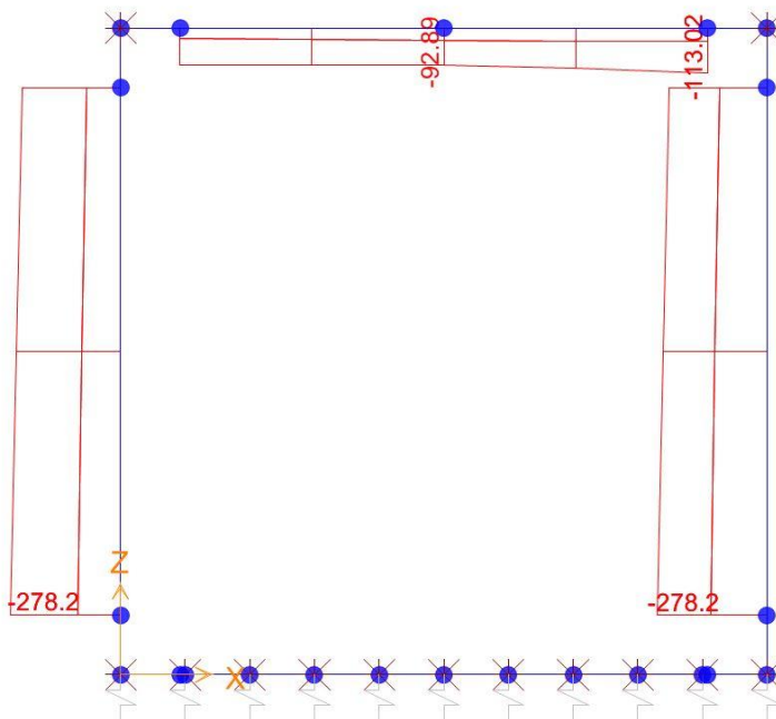
Sforzo normale
