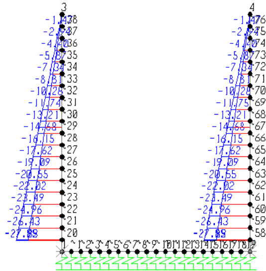
Fig. 12 – Inviluppo azioni assiali SLU
