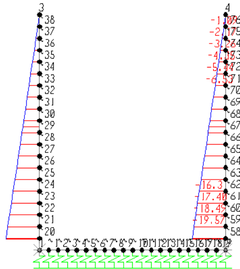
Fig. 17 – Involuppo azioni assiali SLE rara
