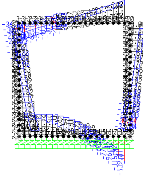
Fig. 6 – Involuppo sforzi taglienti SLV
