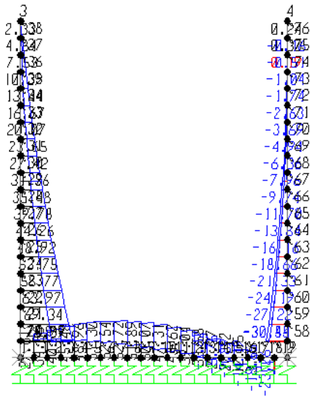
Fig. 14 – Inviluppo sforzi taglianti SLV
