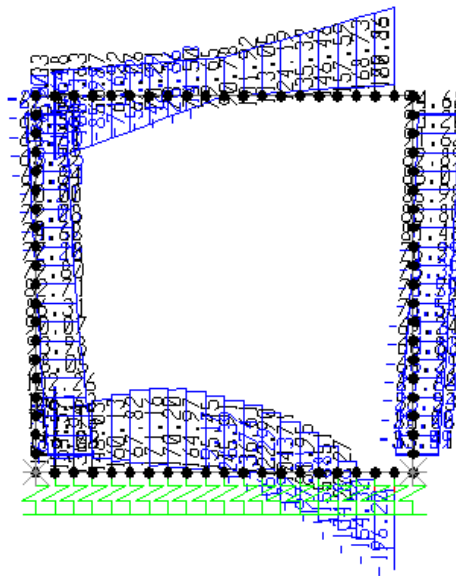
Fig. 3 – Involuppo sforzi taglienti SLU
