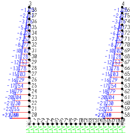
Fig. 15 – Inviluppo azioni assiali SLV
