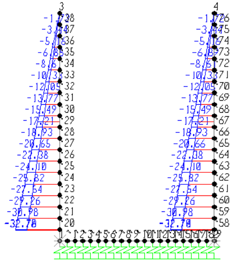
Fig. 9 – Inviluppo azioni assiali SLU
