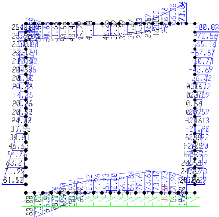
Fig. 5 – Involuppo momenti flettenti SLE rara
