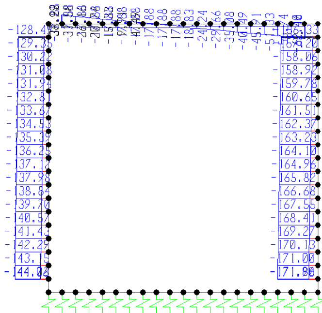
Fig. 6 – Involuppo azioni assiali SLE rara
