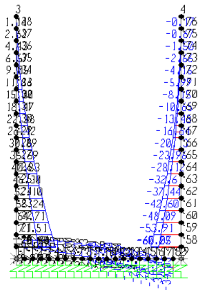
Fig. 8 – Involuppo sforzi taglienti SLU
