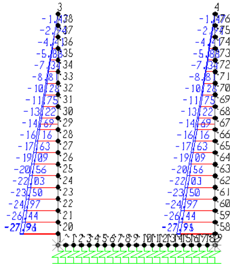
Fig. 12 – Involuppo azioni assiali SLV
