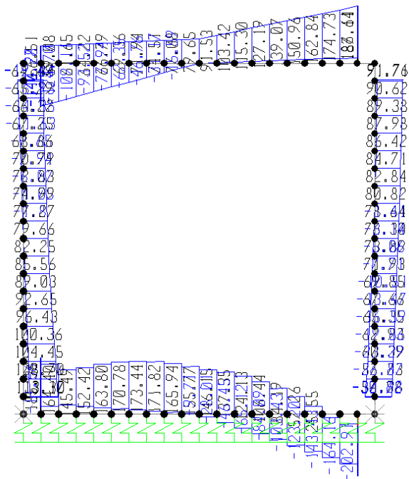
Fig. 3 – Involucro sforzi taglienti SLU-SLV
