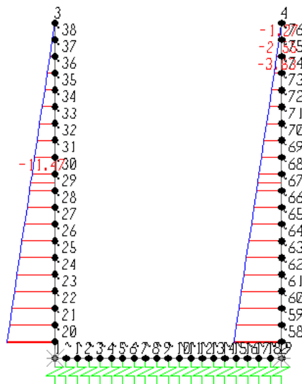
Fig. 14 – Inviluppo azioni assiali SLE rara
