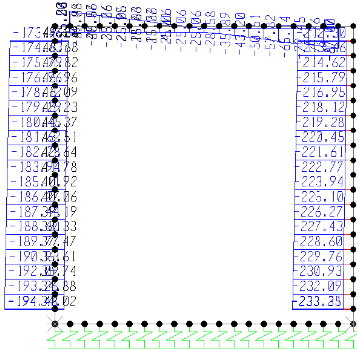
Fig. 4 – Involuppo azioni assiali SLU-SLV
