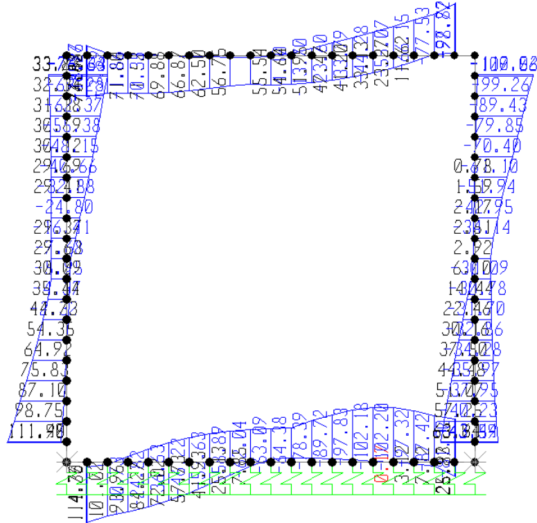
Fig. 2 – Involucro momenti flettenti SLU-SLV
