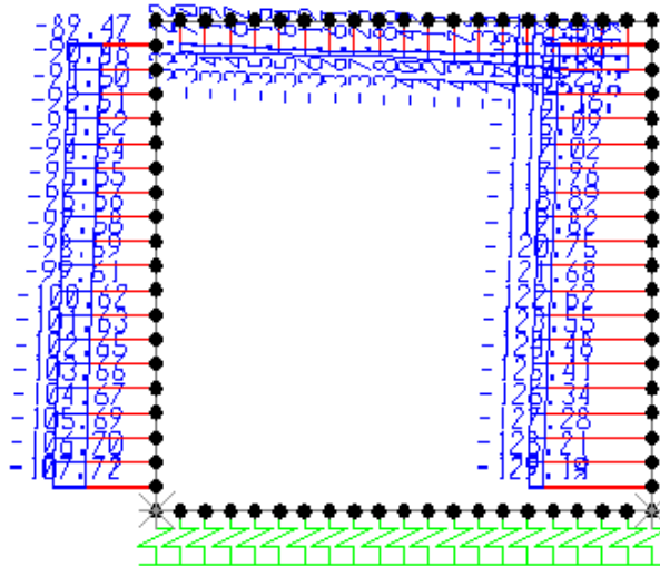
Fig. 7 – Involuppo azioni assiali SLV
