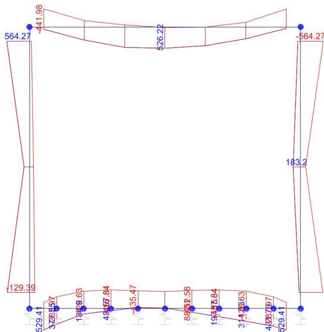
Momento Flettente
