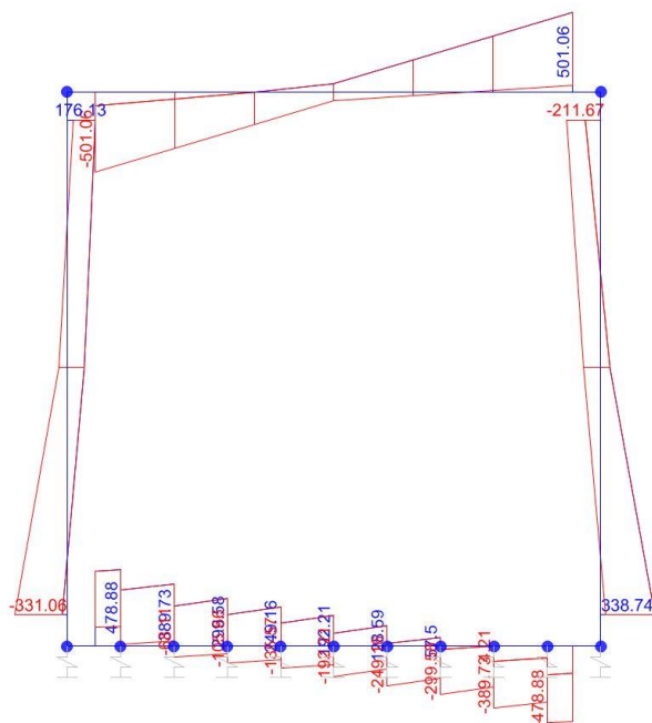
Taglio
