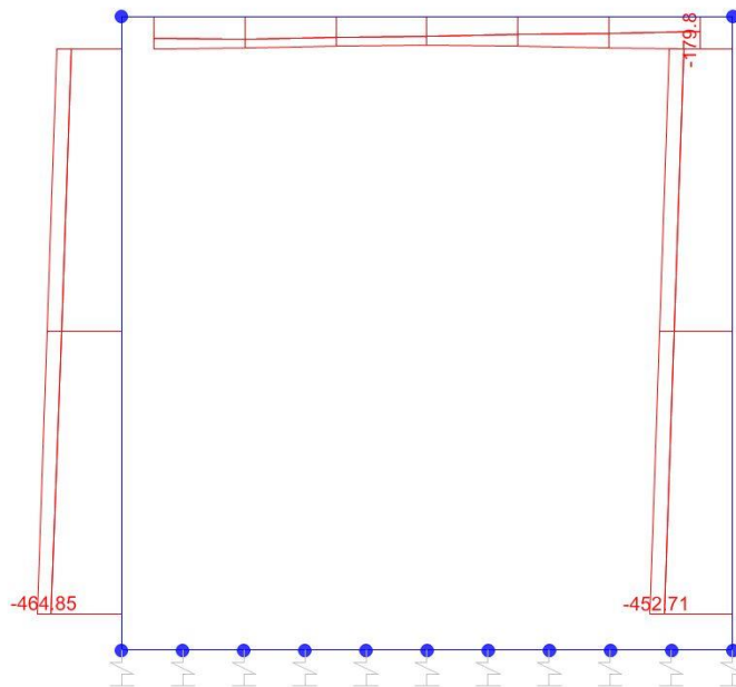
Sforzo normale
