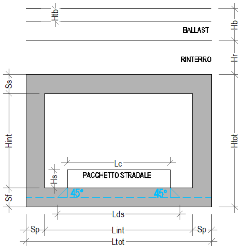
Figura 2. Sezione trasversale dello scatolare
