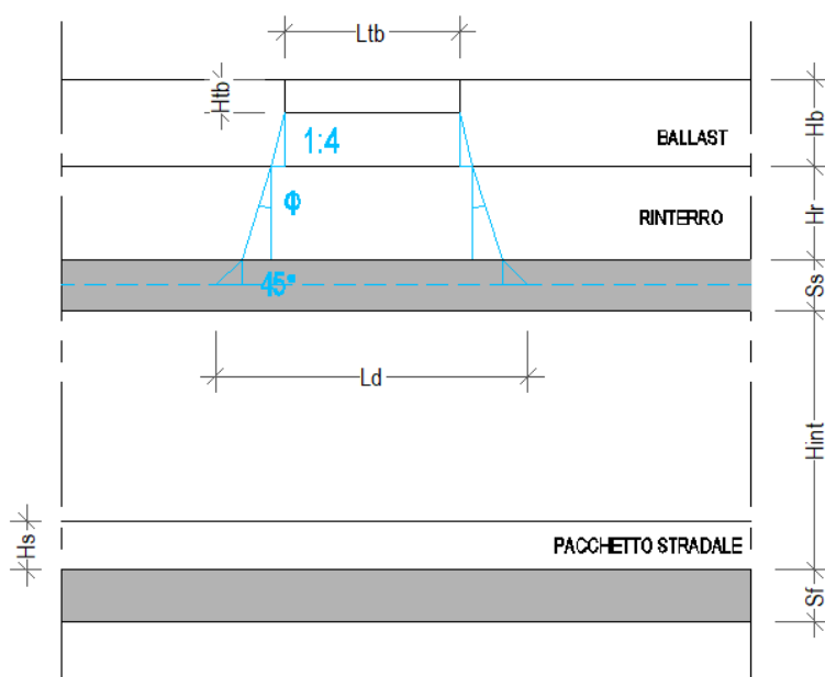
Figura 1. Sezione longitudinale dello scatolare
