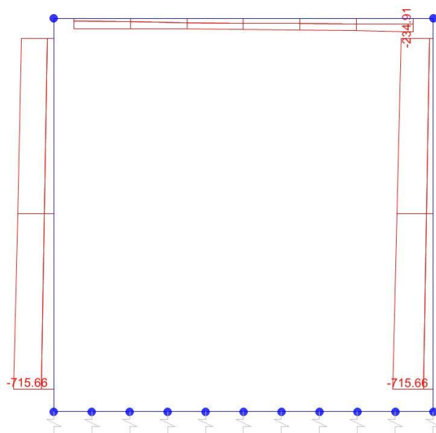
Sforzo normale
