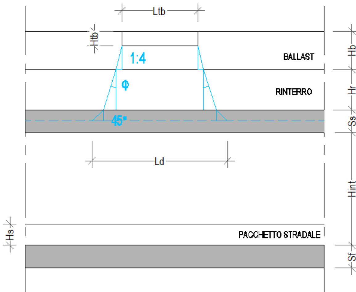
Figura 7. Schema modalità di diffusione dei carichi ferroviari
