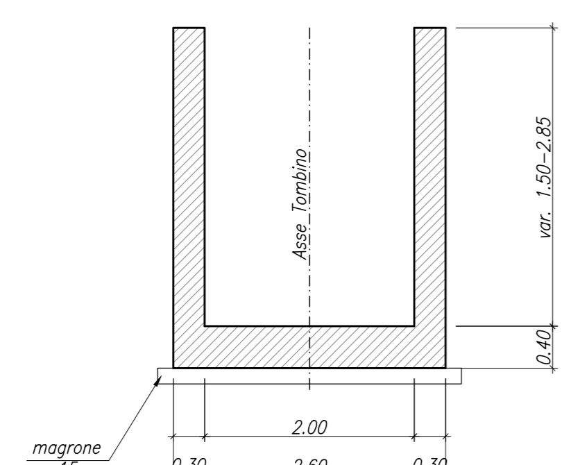
TOMBINO STRADALE IN21 SEZIONE B-B SCALA 1:50
