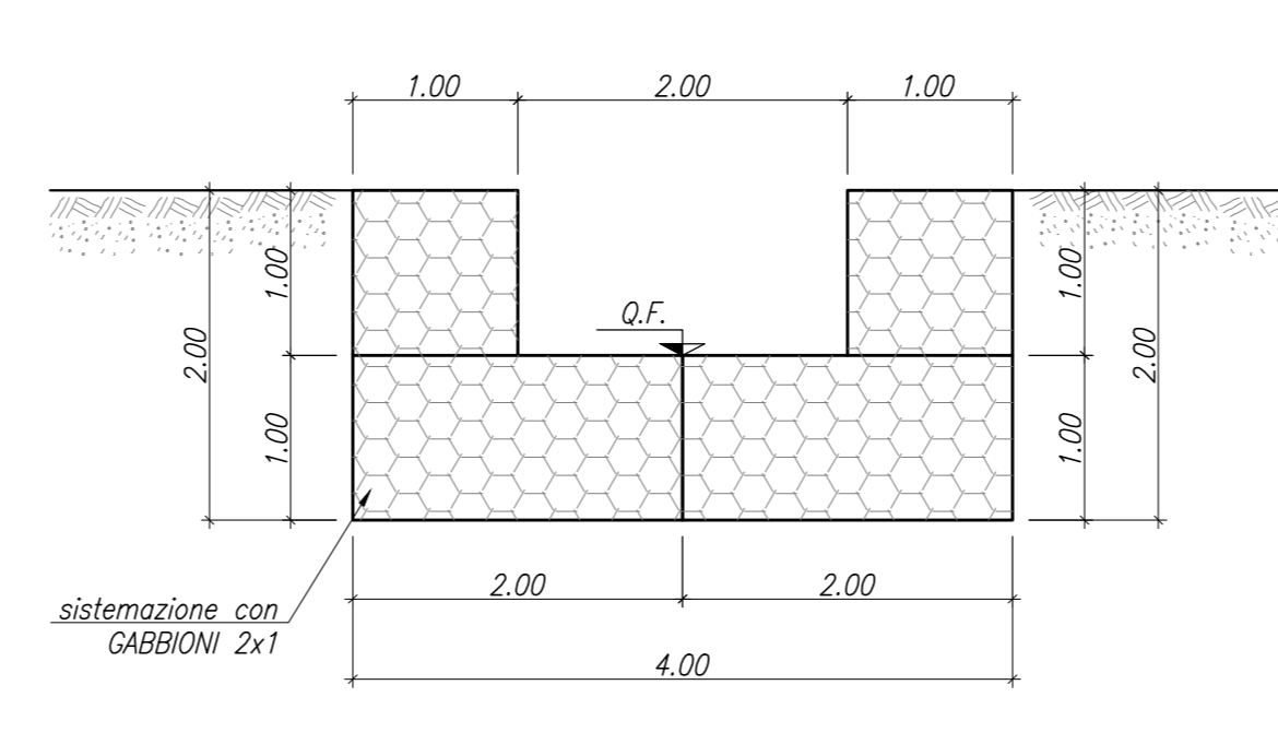
TOMBINO STRADALE IN21 SEZIONE TIPO GABBIONE 2x1 SCALA 1:50
