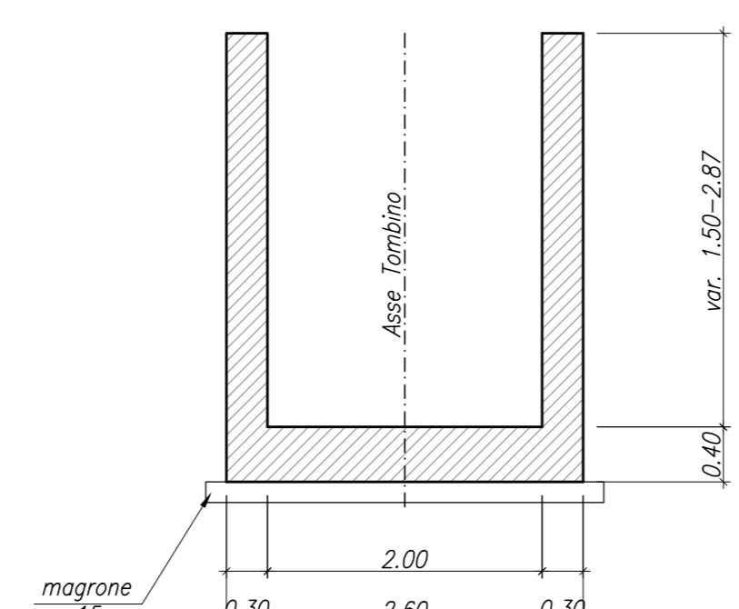
TOMBINO STRADALE IN21 SEZIONE C-C SCALA 1:50
