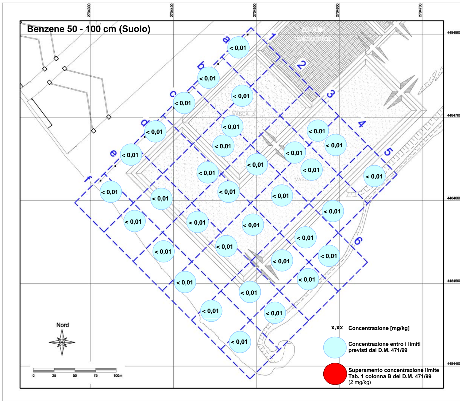
Tav. 23: a) Benzene 50 – 100 cm (Suolo)
