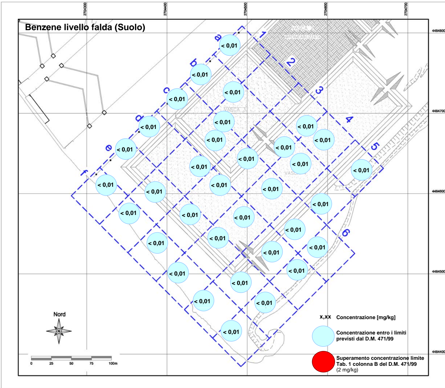
Tav. 23: b) Benzene livello falda (Suolo)
