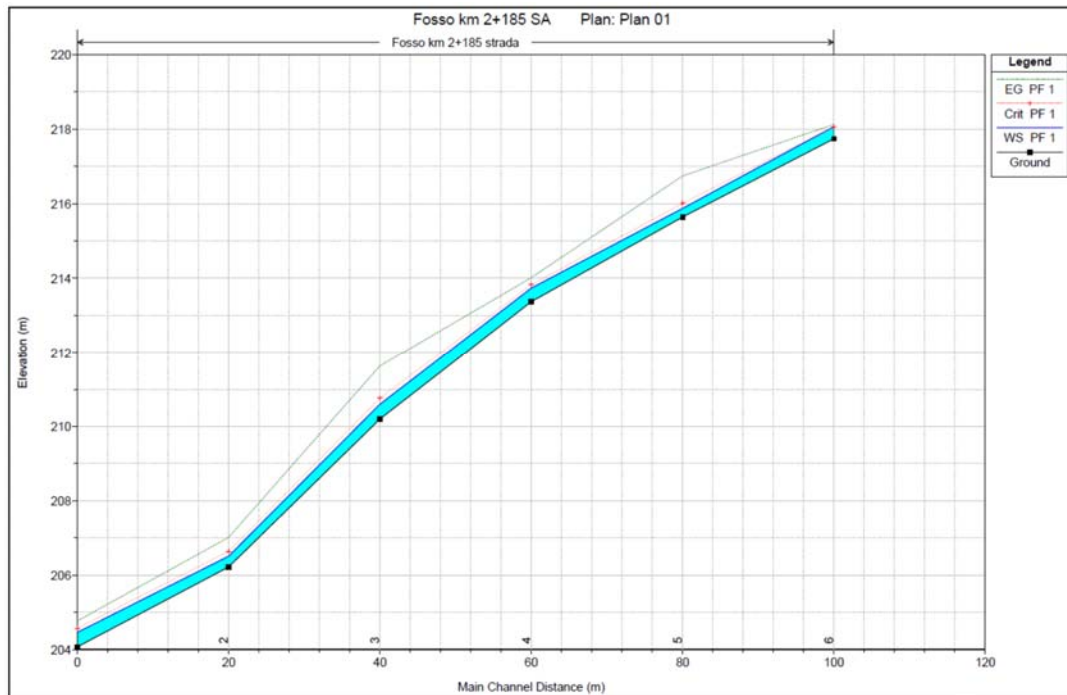
Figura 14 - Profilo di corrente AO NV02 pk 2+208
