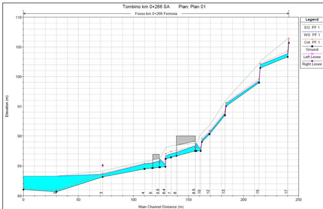
Figura 3 - Profilo di corrente AO pk 0+265
