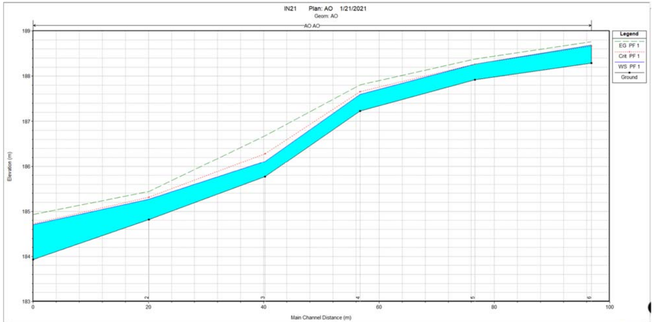
Figura 11 - Profilo di corrente AO NV02 pk 1+370
