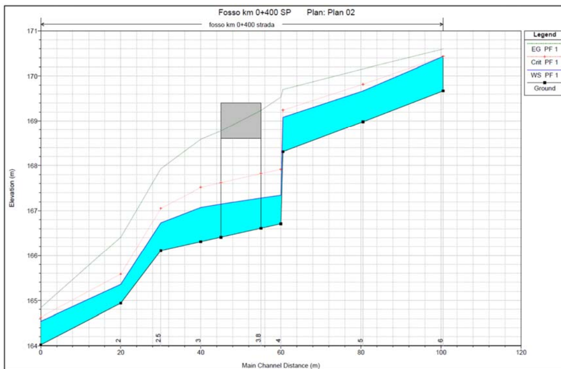
Figura 29 - Profilo di corrente PO NV02 pk 0+420
