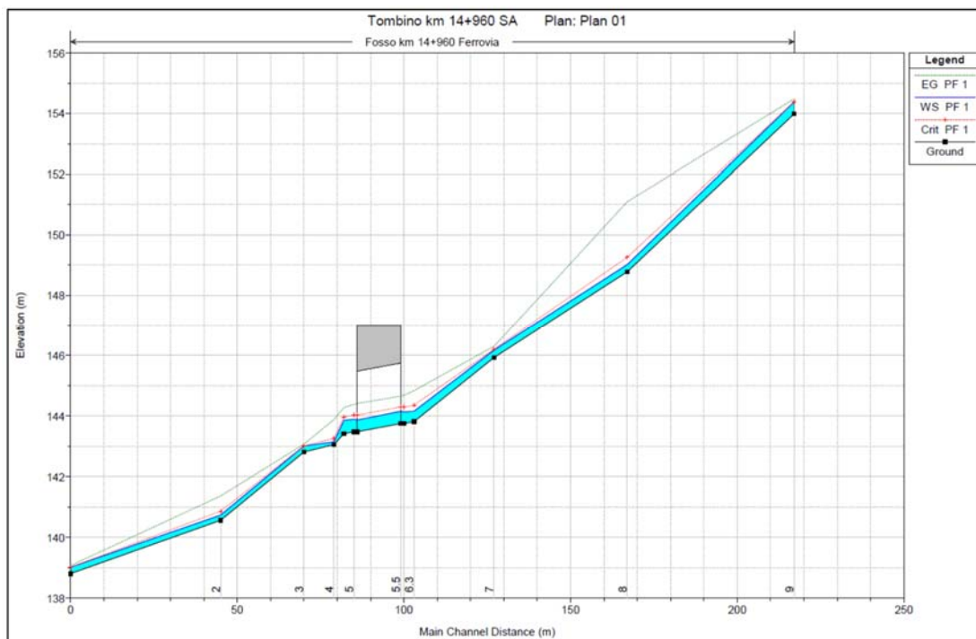
Figura 23 - Profilo di corrente PO pk 14+960
