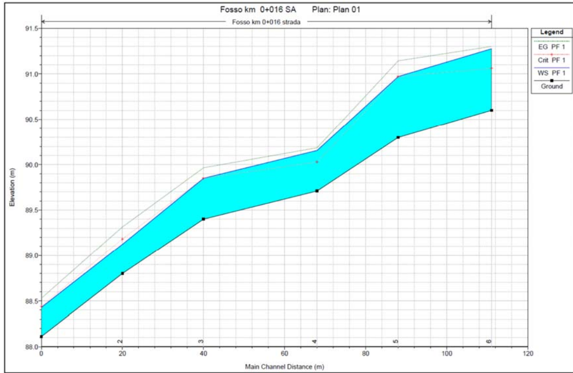
Figura 6 - Profilo di corrente AO NV01 pk 0+016
