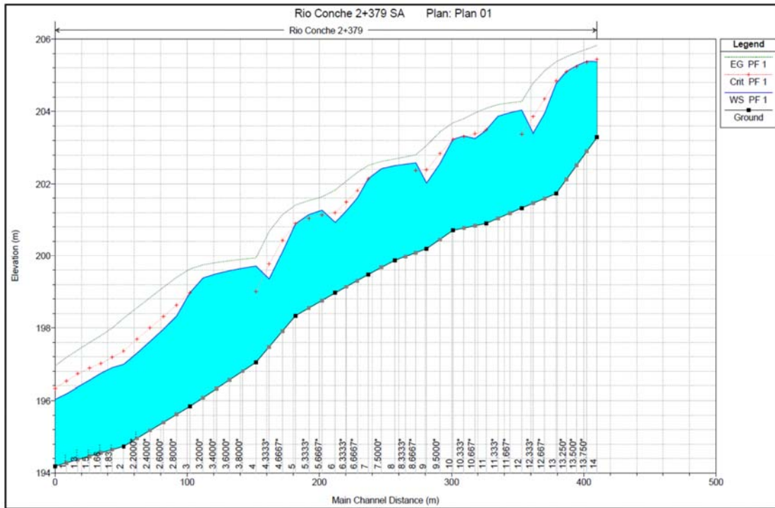
Figura 16 - Profilo di corrente AO NV02 pk 2+402
