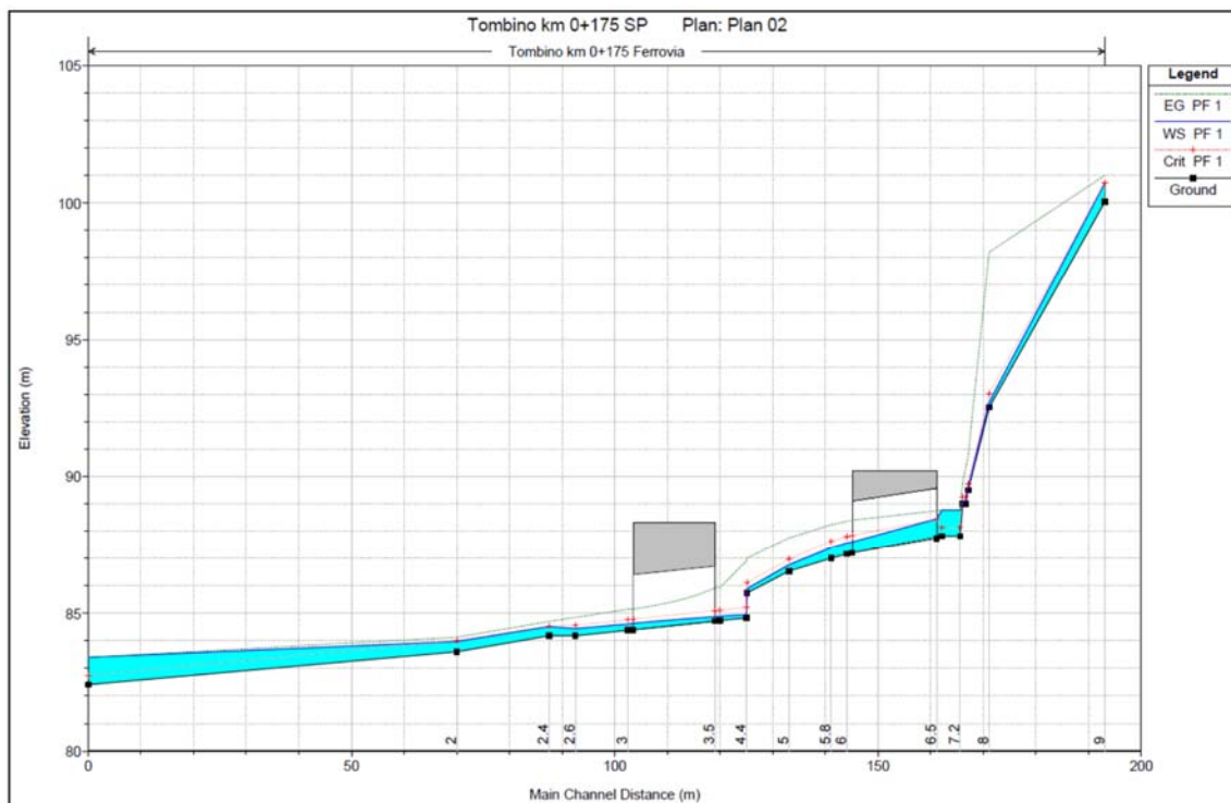
Figura 17 - Profilo di corrente PO pk 0+176
