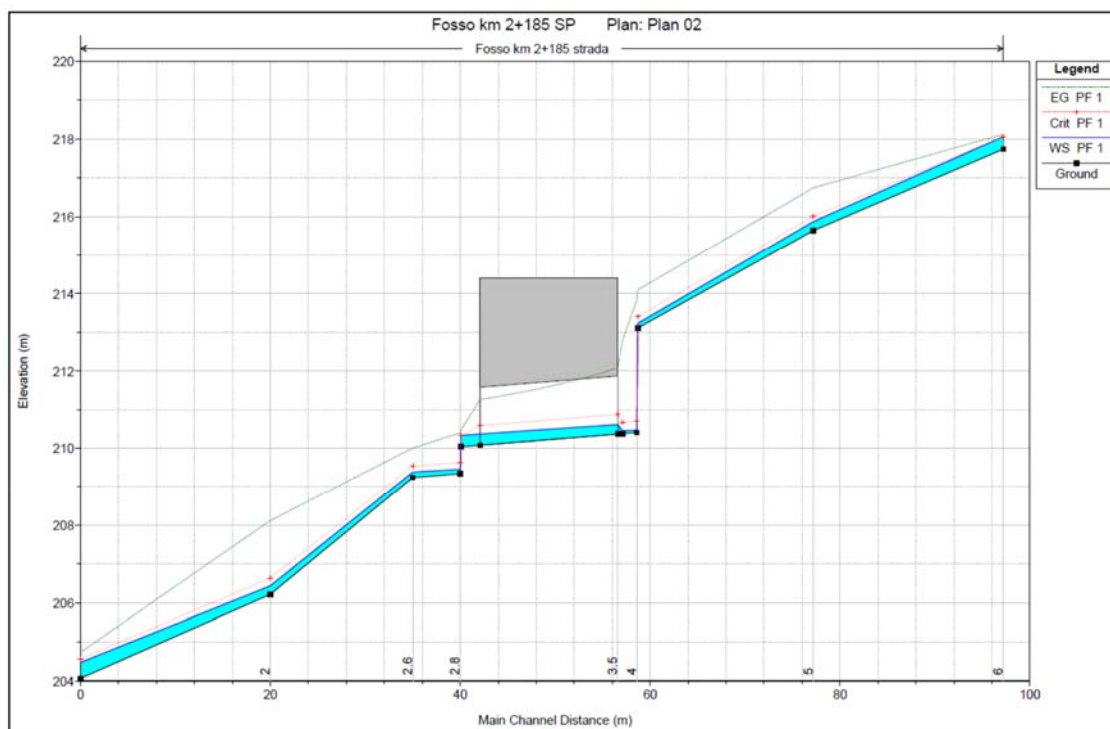
Figura 35 - Profilo di corrente PO NV02 pk 2+208
