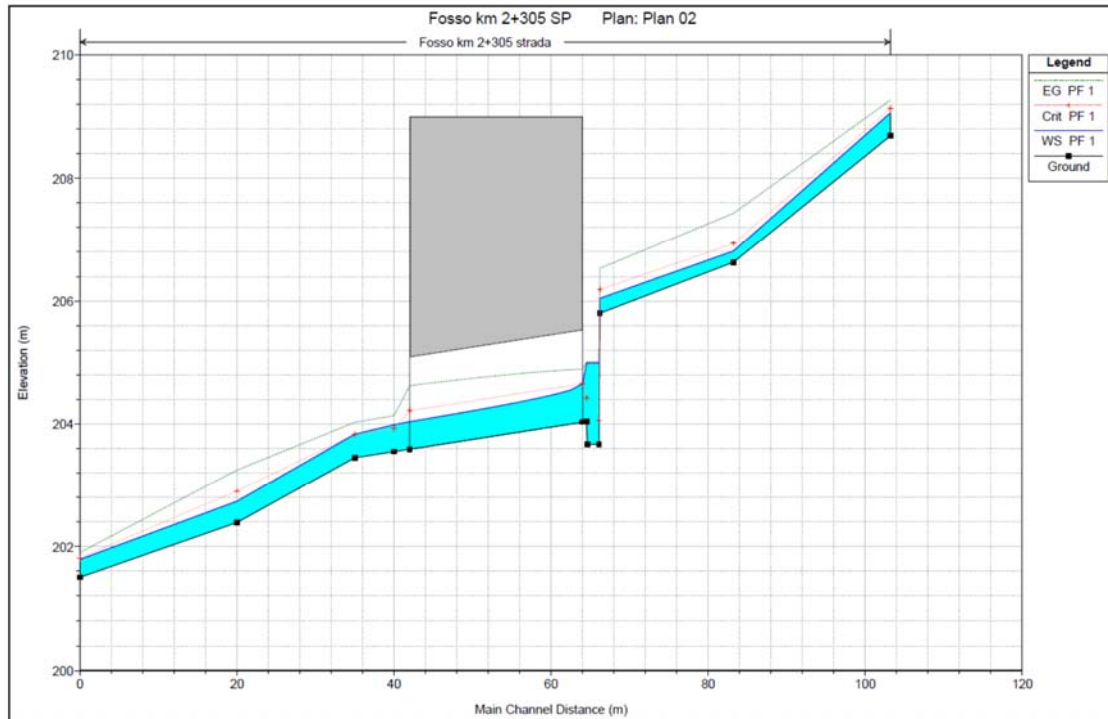
Figura 36 - Profilo di corrente PO NV02 pk 2+339
