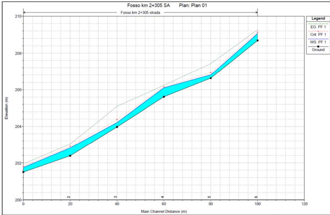
Figura 15 - Profilo di corrente AO NV02 pk 2+339
