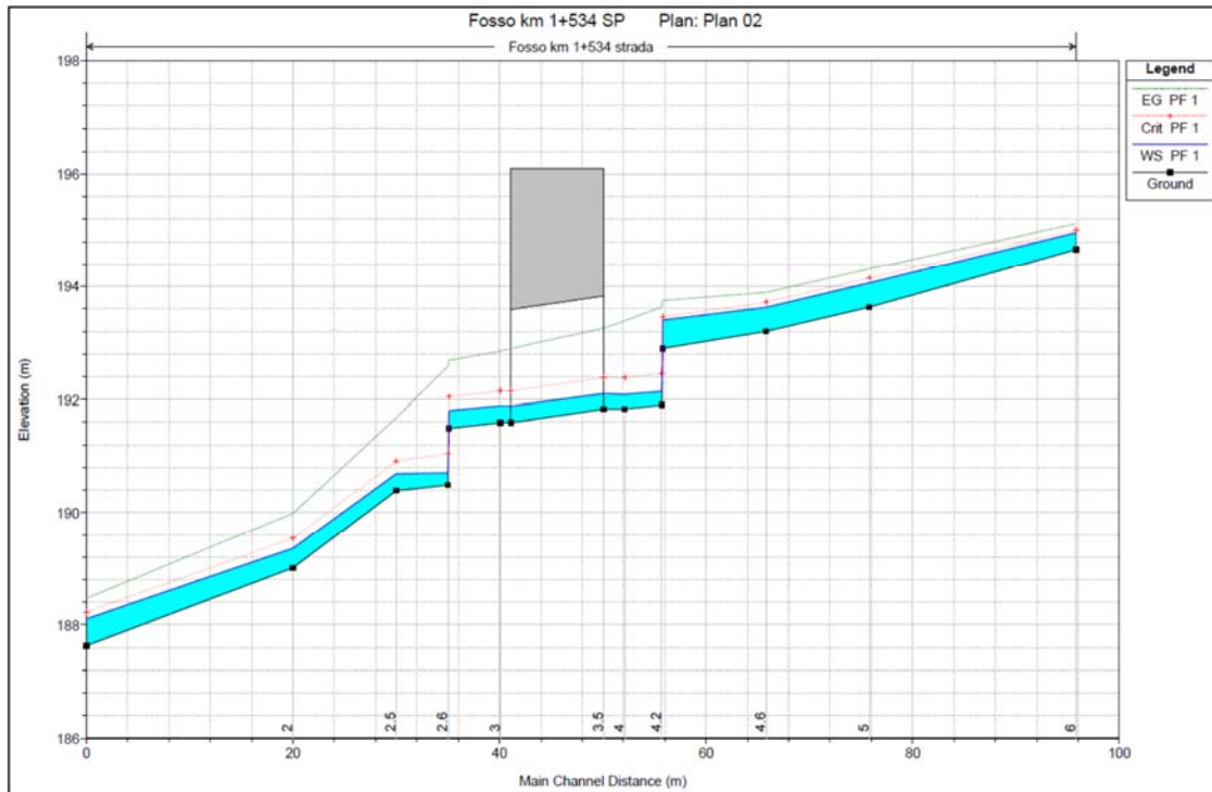
Figura 33 - Profilo di corrente PO NV02 pk 1+554
