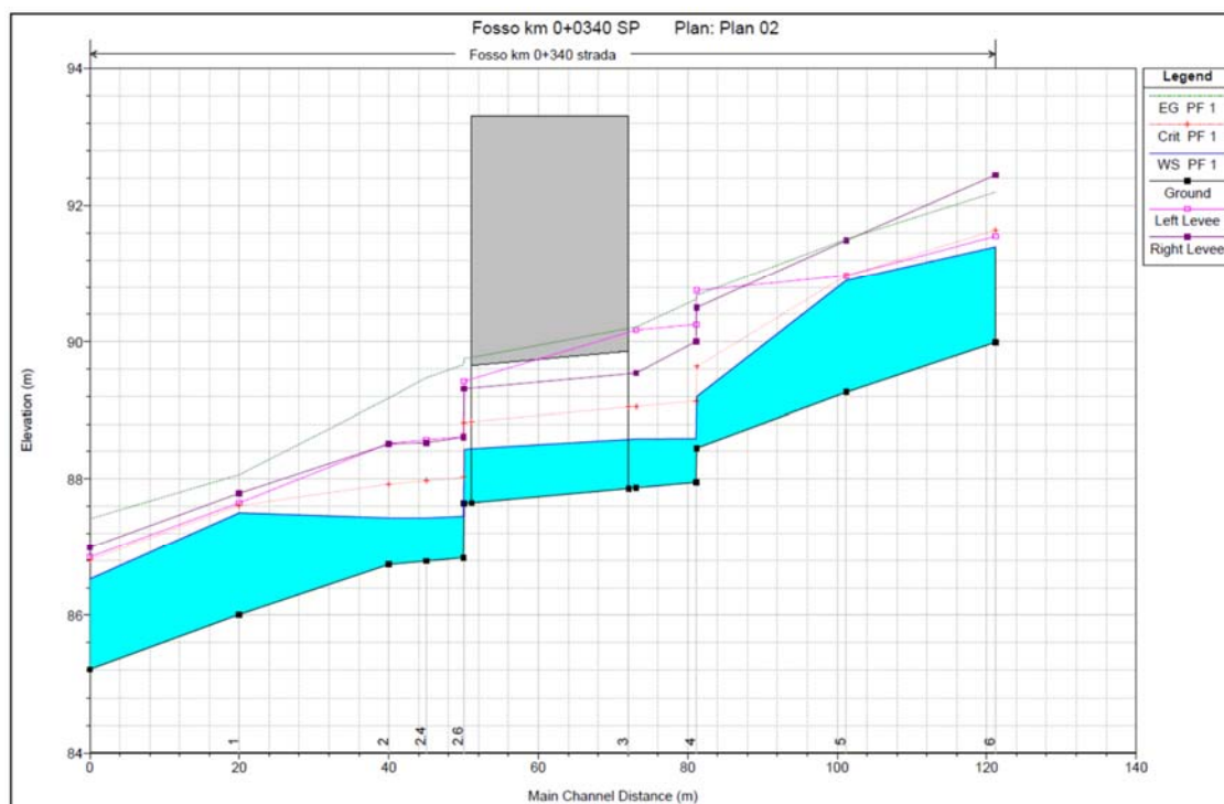
Figura 28 - Profilo di corrente PO NV01 pk 0+340
