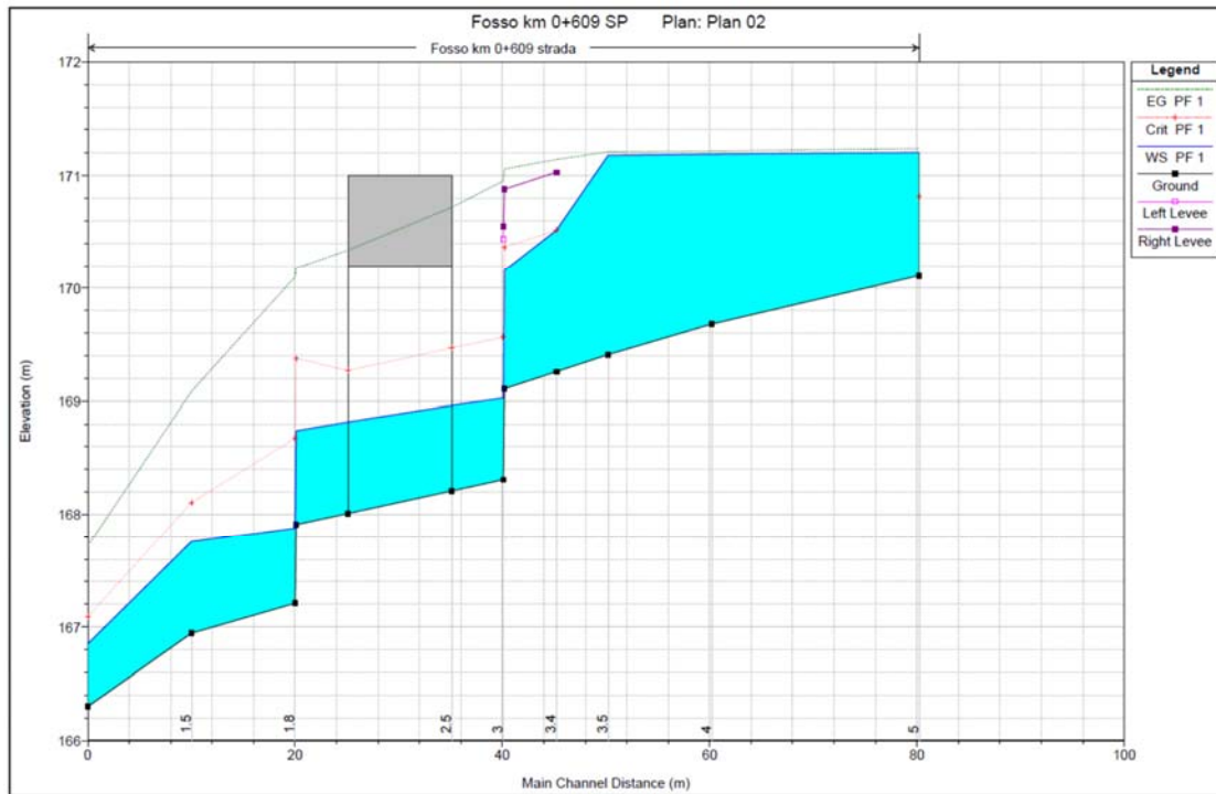
Figura 30 - Profilo di corrente PO NV02 pk 0+631
