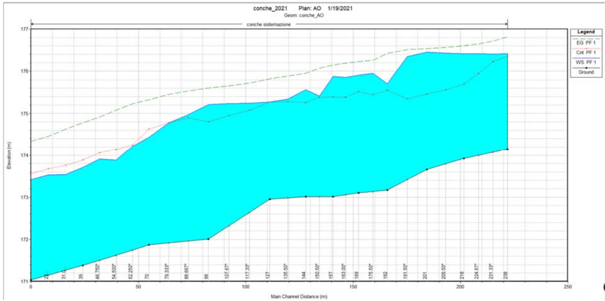
Figura 10 - Profilo di corrente AO NV02 pk 1+028
