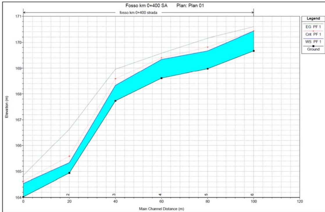
Figura 8 - Profilo di corrente AO NV02 pk 0+420
