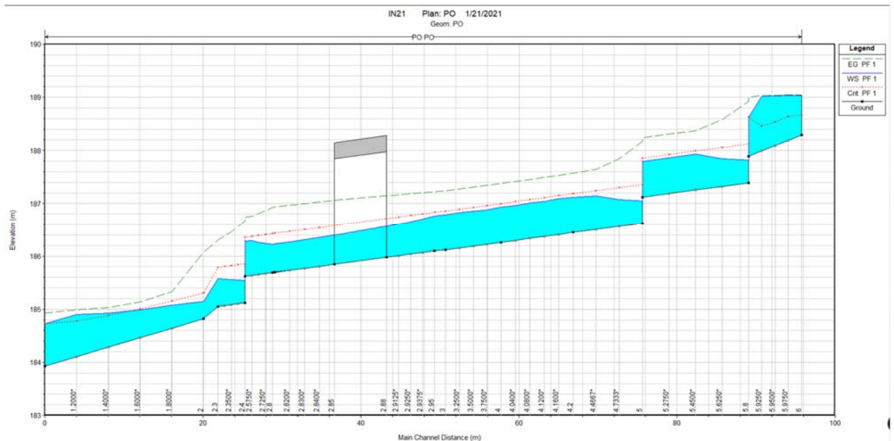
Figura 32 - Profilo di corrente PO NV02 pk 1+370
