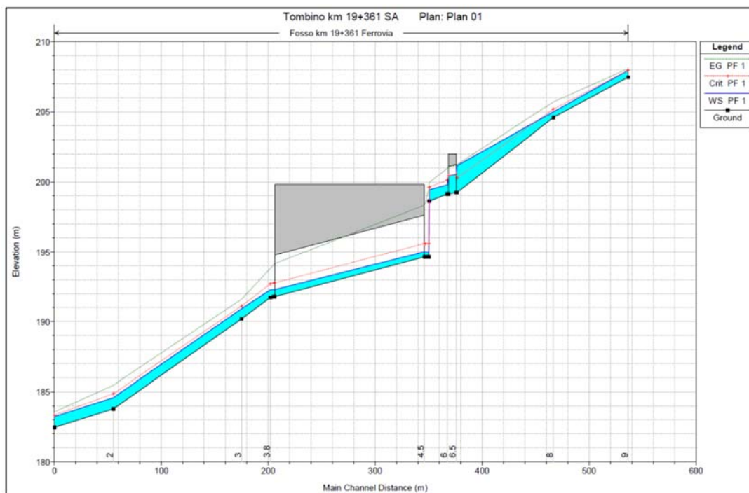
Figura 25 - Profilo di corrente PO pk 19+391
