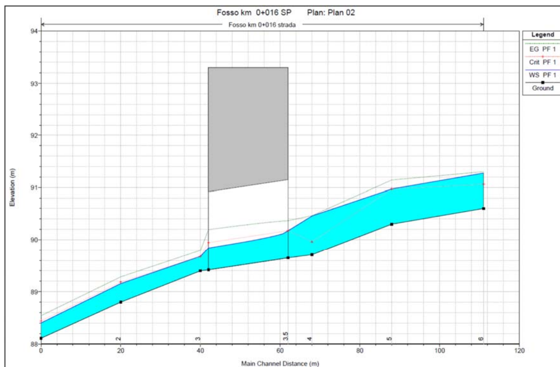
Figura 27 - Profilo di corrente PO NV01 pk 0+016
