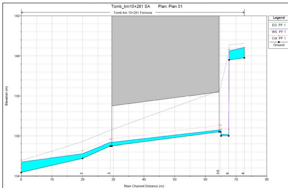
Figura 22 - Profilo di corrente PO pk 10+281
