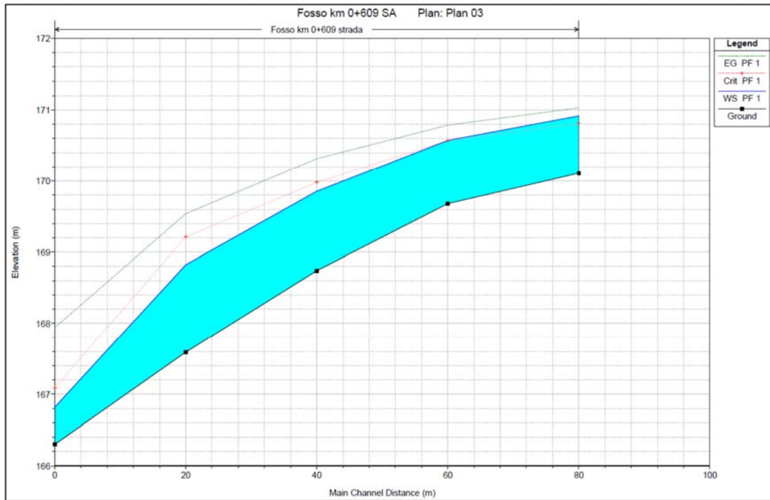
Figura 9 - Profilo di corrente AO NV02 pk 0+631
