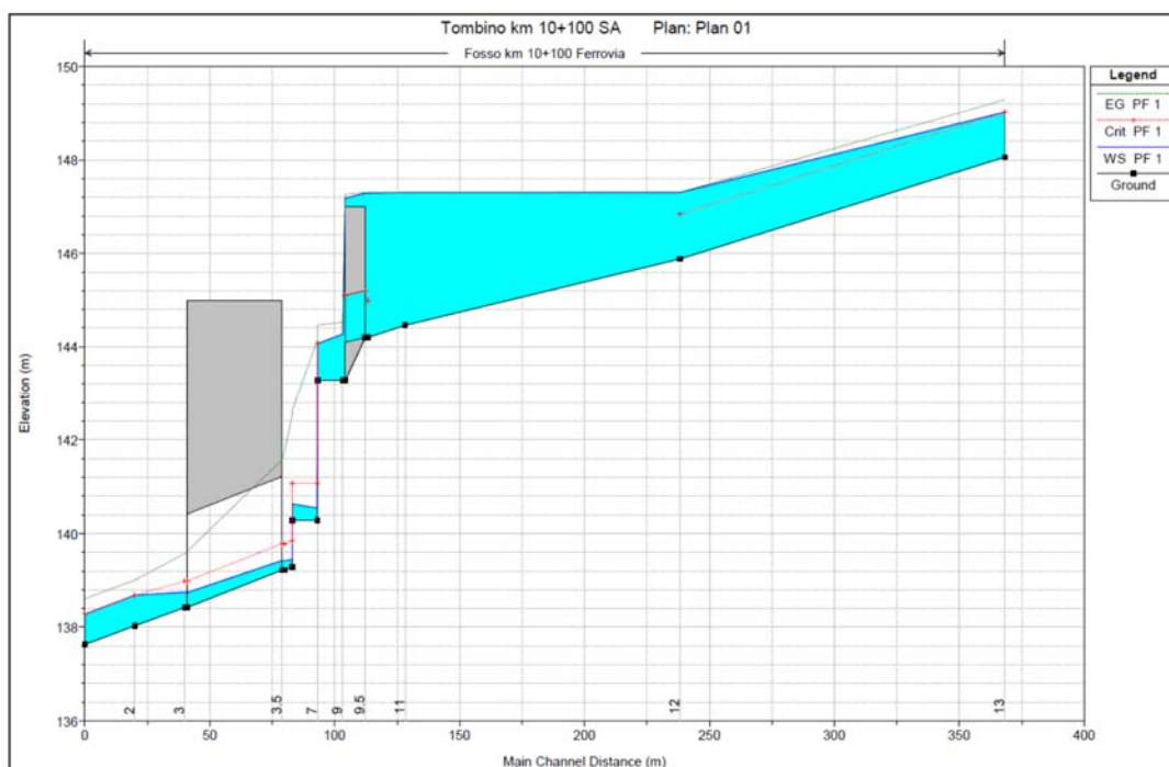
Figura 21 - Profilo di corrente PO pk 10+101
