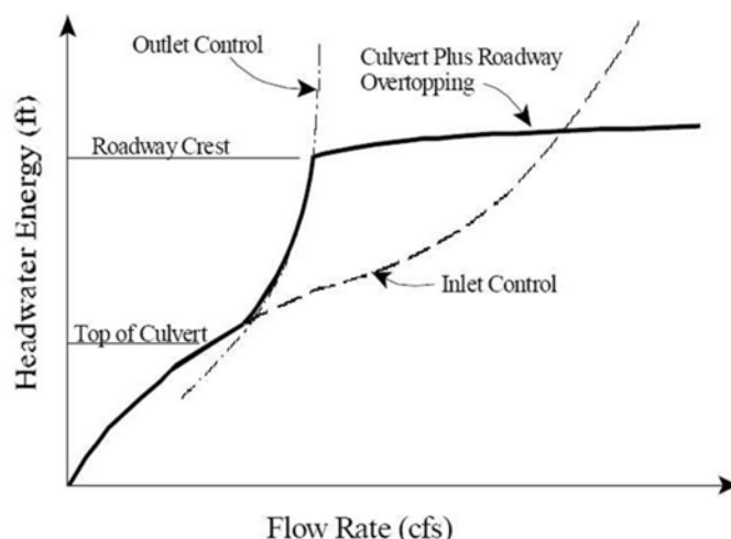
Figura 11 – Diagramma di funzionamento del tombino/ponticello.
