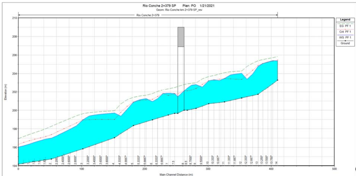
Figura 37 - Profilo di corrente PO NV02 pk 2+402
