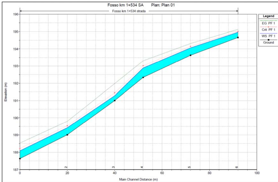
Figura 12 - Profilo di corrente AO NV02 pk 1+554
