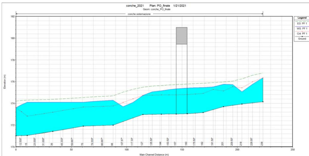
Figura 31 - Profilo di corrente PO NV02 pk 1+028
