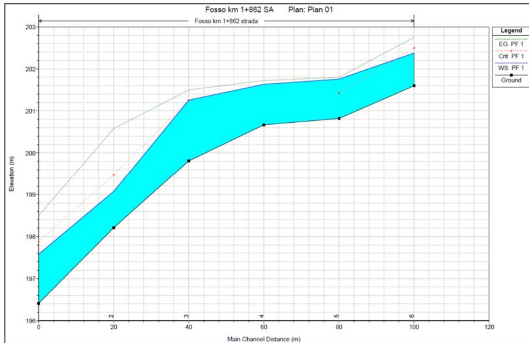
Figura 13 - Profilo di corrente AO NV02 pk 1+883
