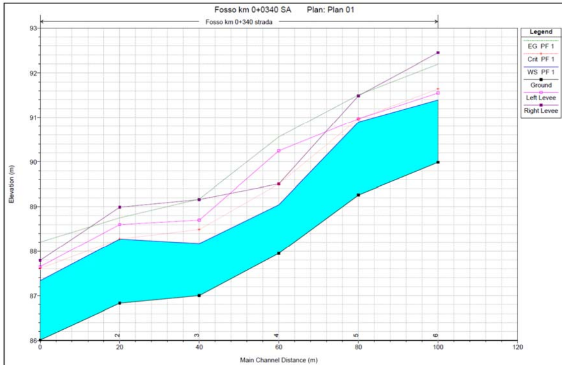
Figura 7 - Profilo di corrente AO NV01 pk 0+340
