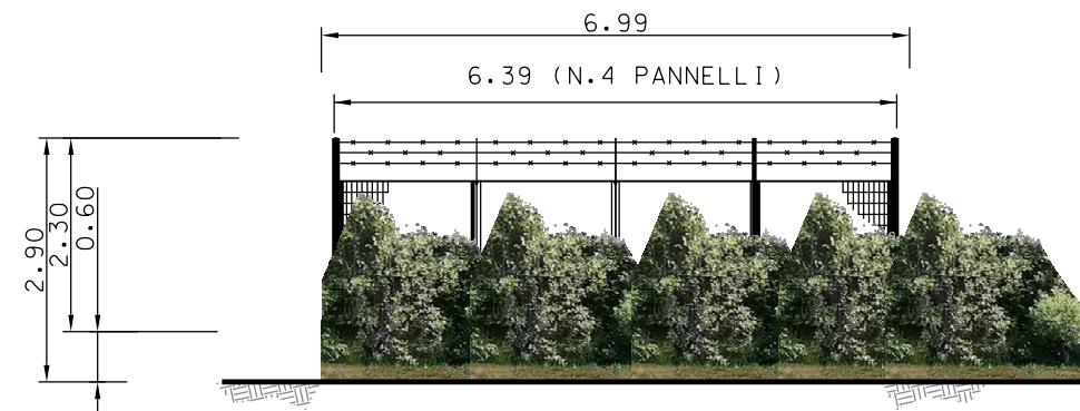
PROSPETTO - B -
