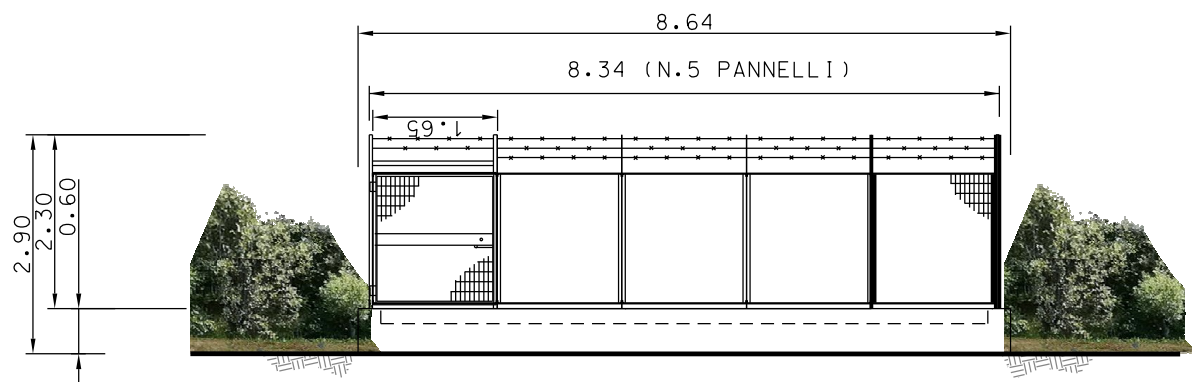
PROSPETTO - A -
