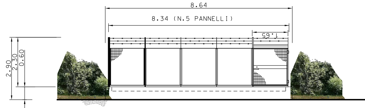
PROSPETTO - A -
