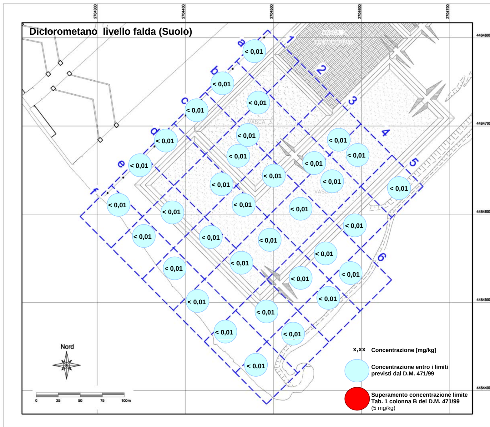
Tav. 30: b) Diclorometano livello falda (Suolo)
