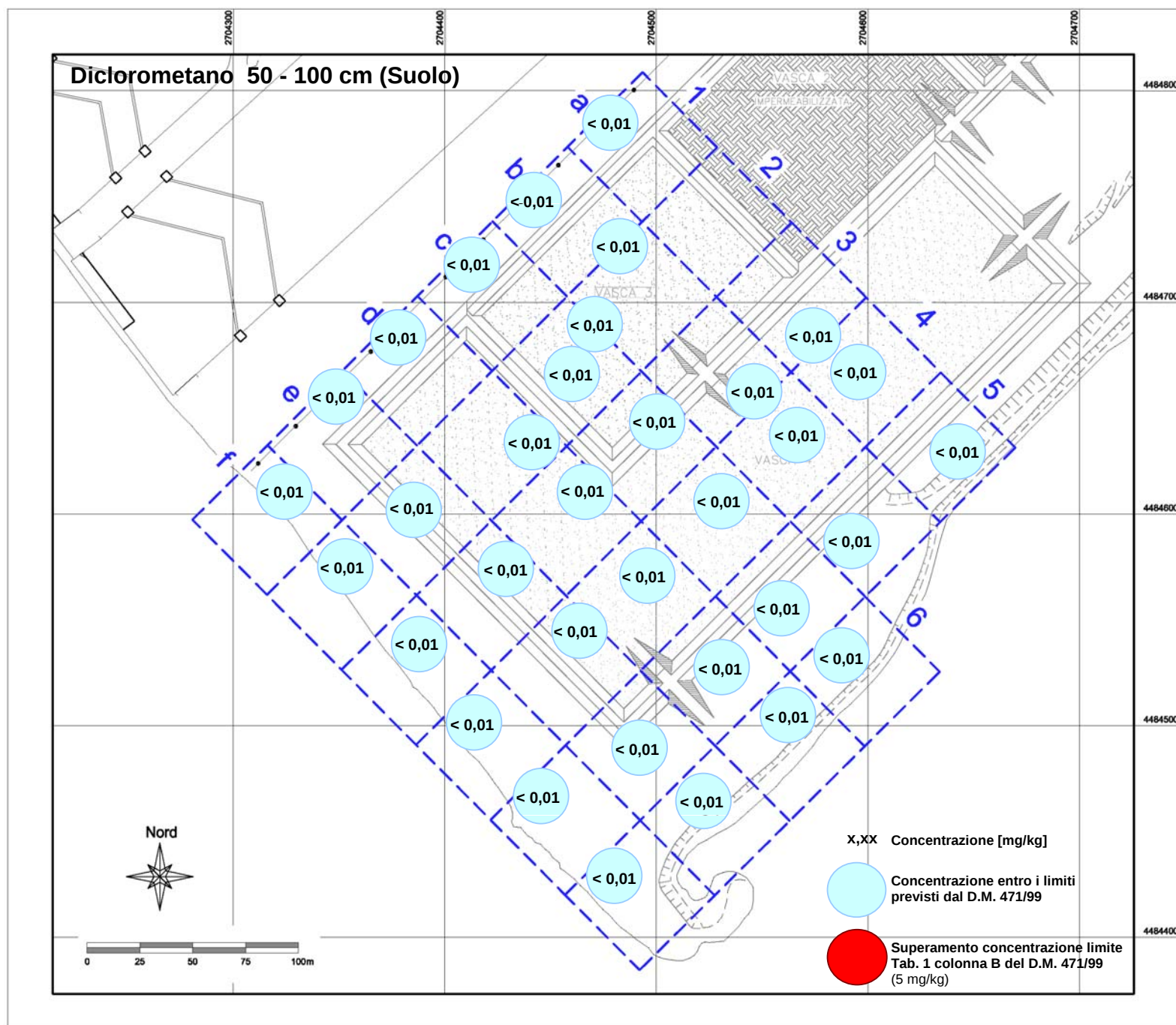
Tav. 30: a) Diclorometano 50 – 100 cm (Suolo)
