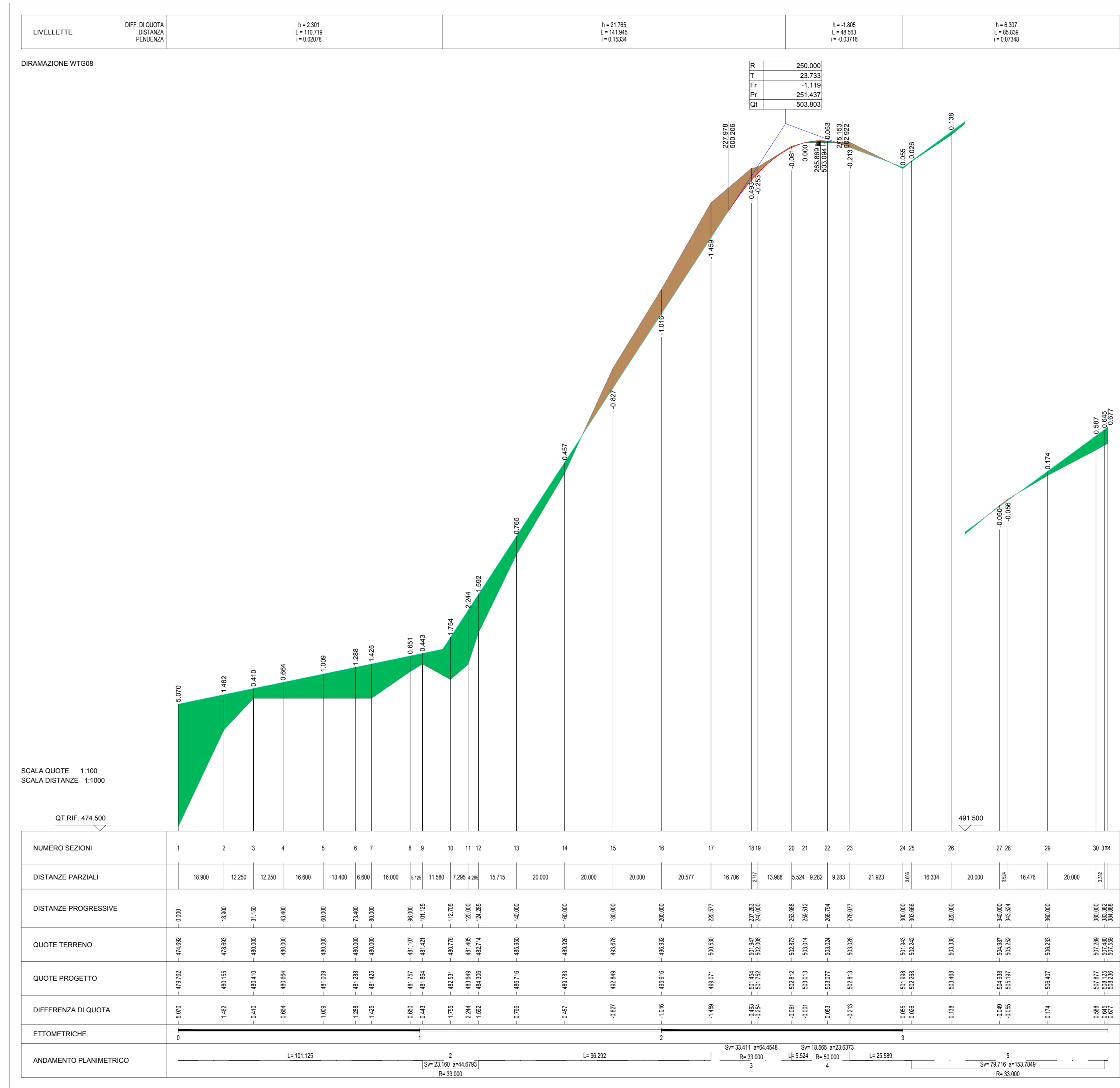
PROFILO LONGITUDINALE VIABILITA' DI SERVIZIO PIAZZOLA
