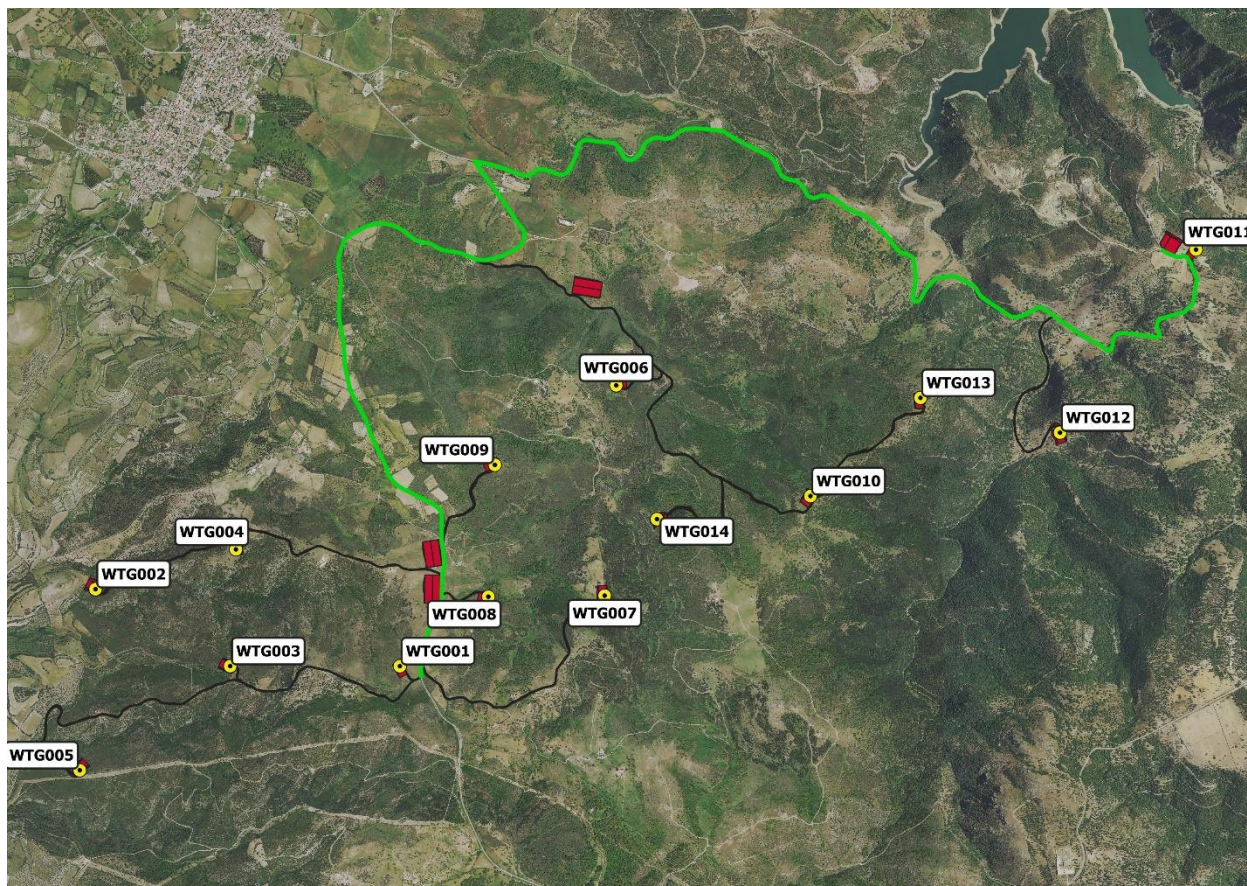
Figura 1: Layout degli aerogeneratori, viabilità interna e viabilità esistente esterna su ortofoto
