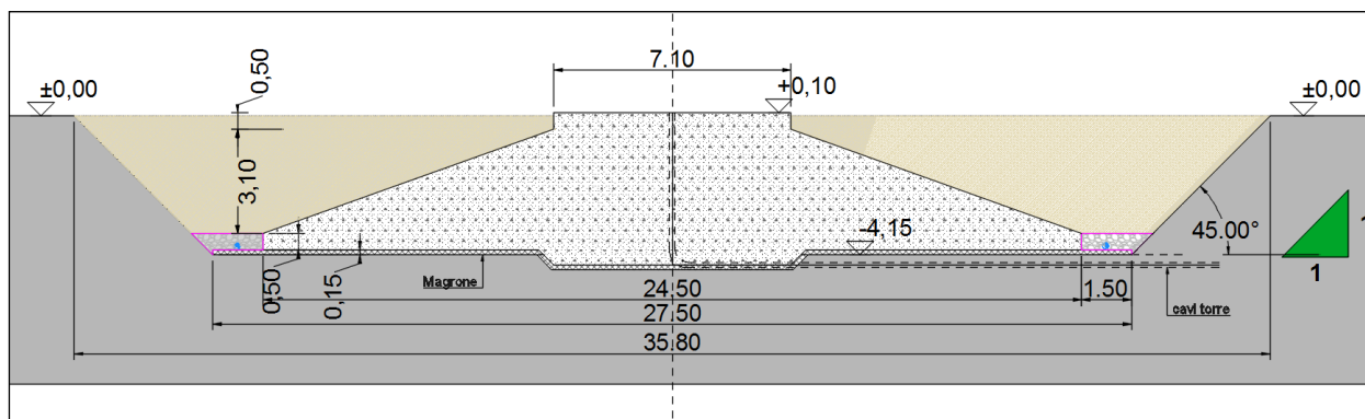
Figura 10 – Schema plinto fondazione aerogeneratore
