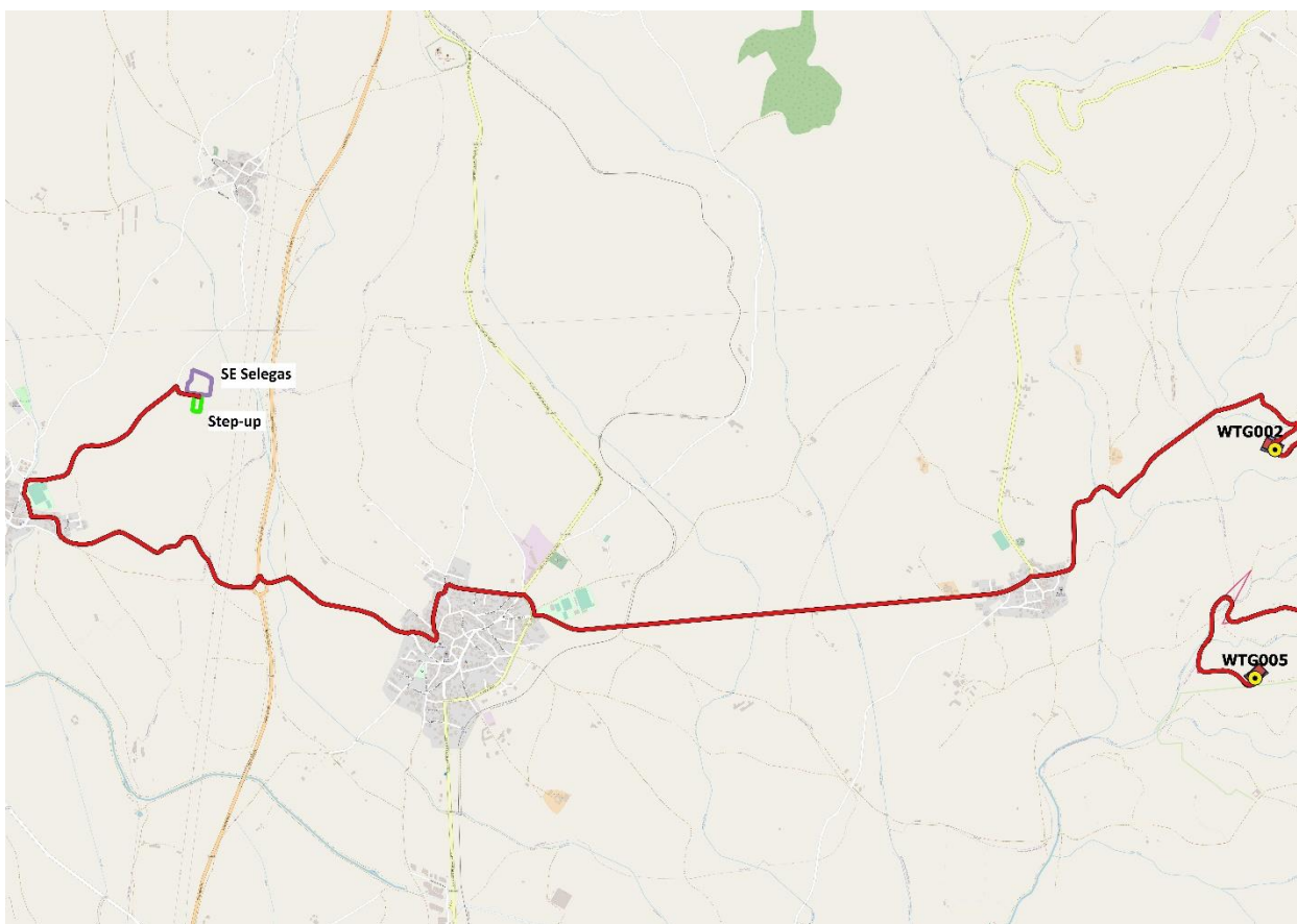
Figura 11 – Elettrodotta interrato verso la SE "Selegas"
