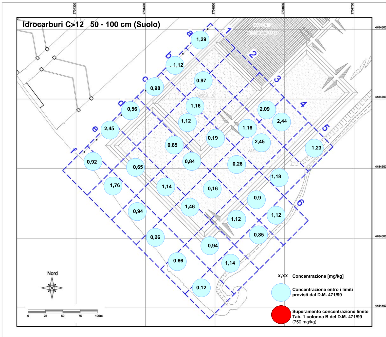
Tav. 37: a) Idrocarburi C>12 50 – 100 cm (Suolo)
