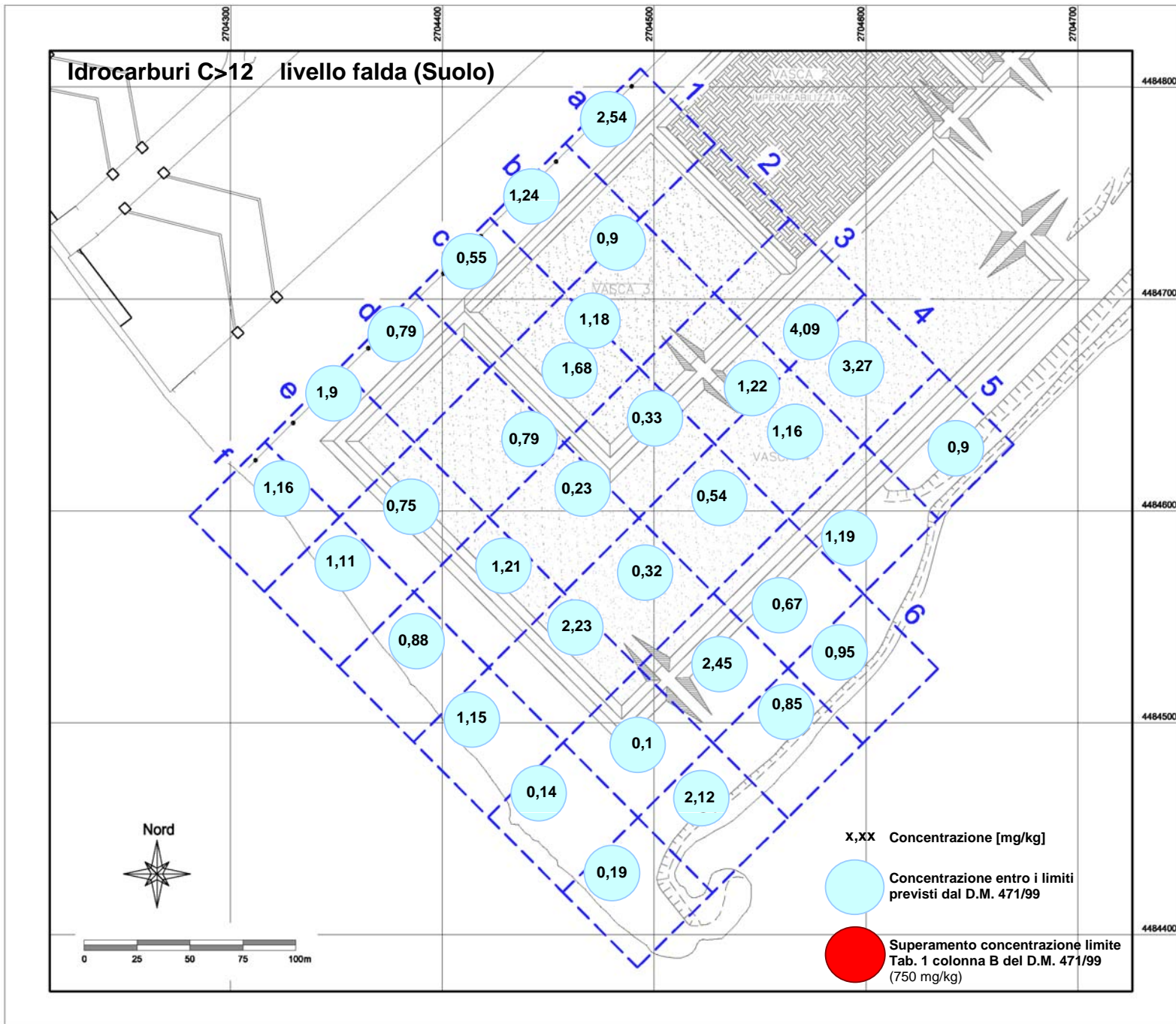
Tav. 37: b) Idrocarburi C>12 livello falda (Suolo)
