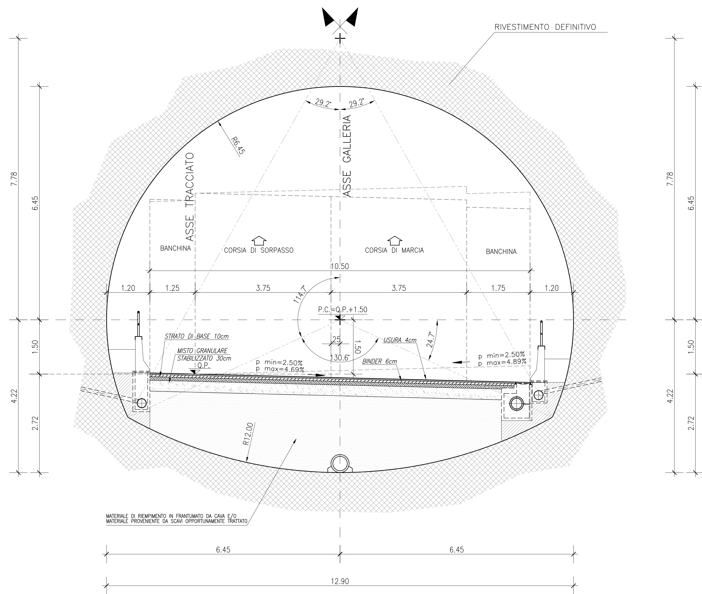
SEZIONE TIPO CORRENTE SCALA 1/50
