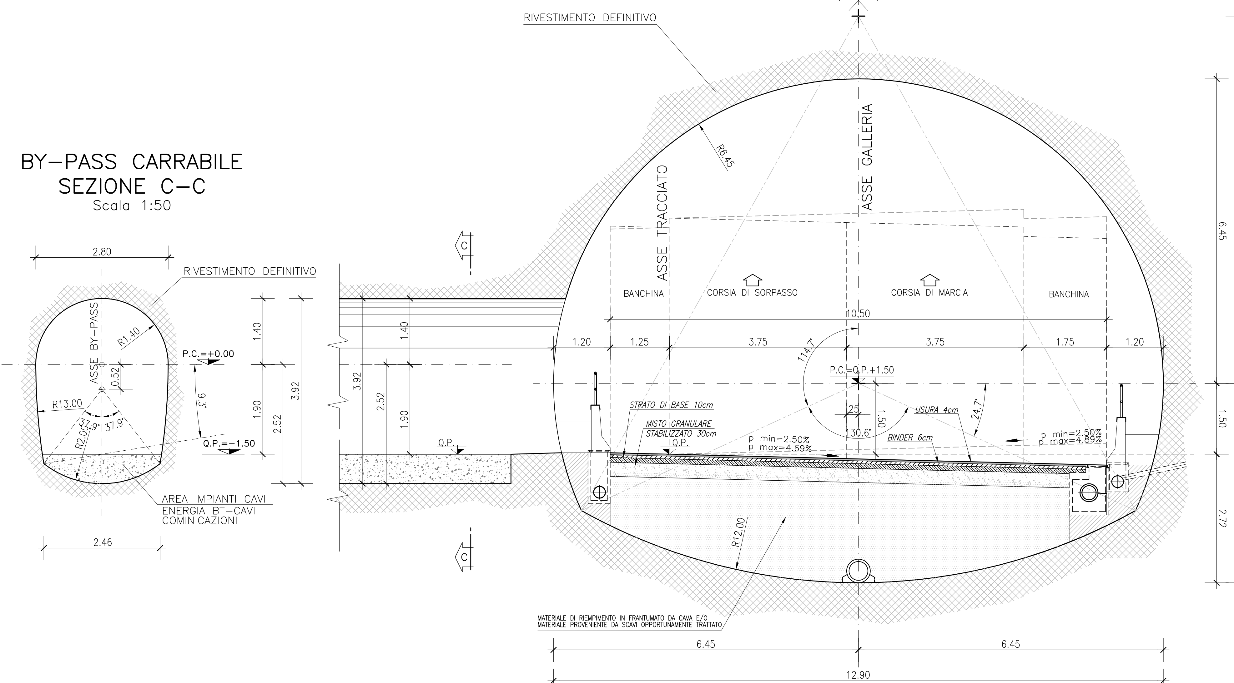
SEZIONE TIPO CON BY-PASS PEDONALE (BPP) SCALA 1:50
