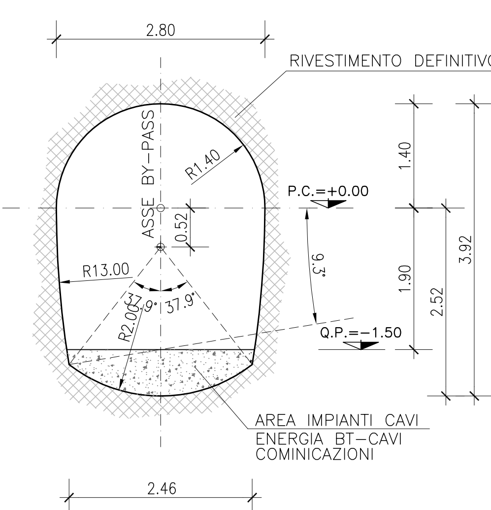
BY-PASS CARRABILE SEZIONE C-C Scala 1:50
