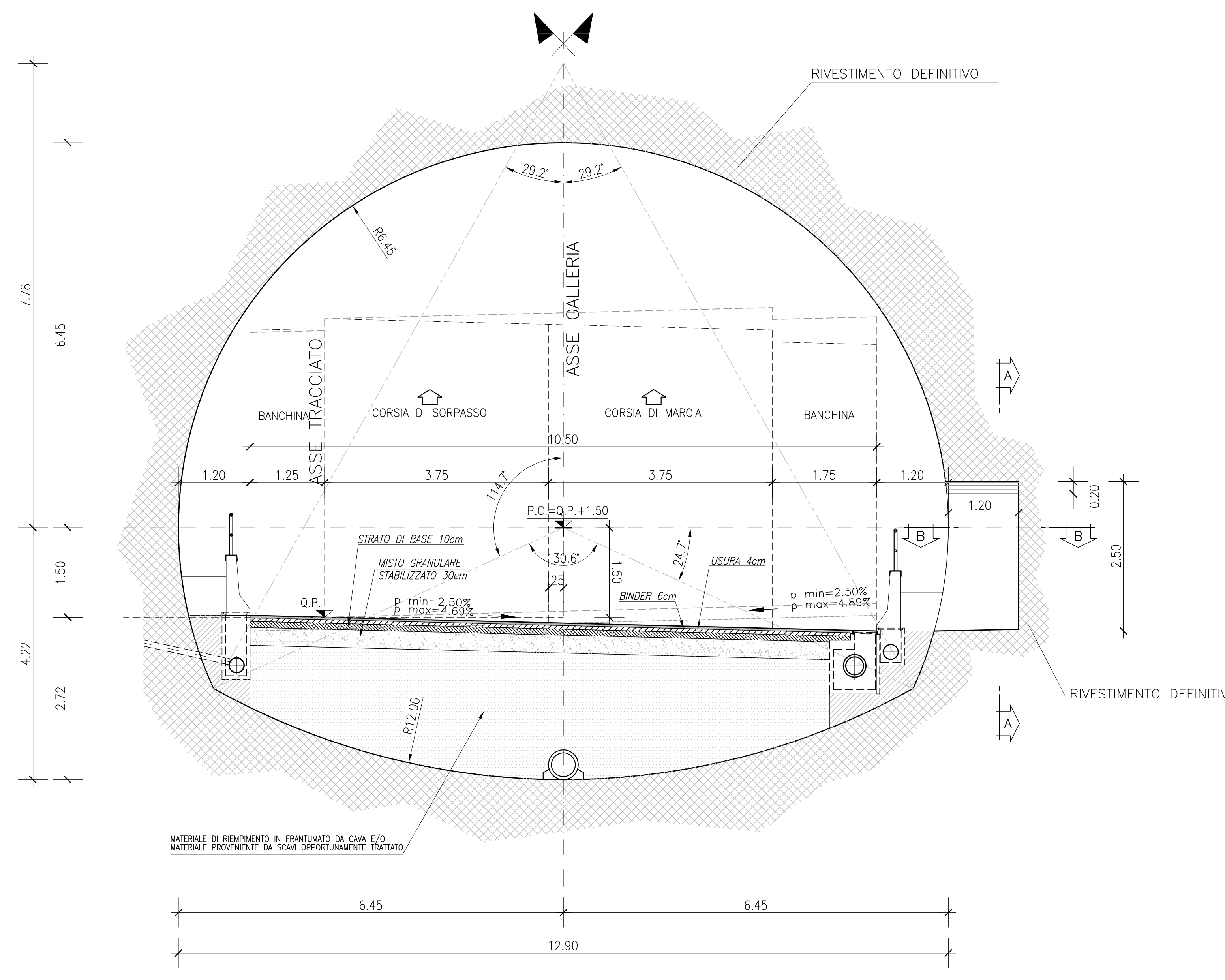
SEZIONE TIPO CON NICCHIA SCALA 1/50
