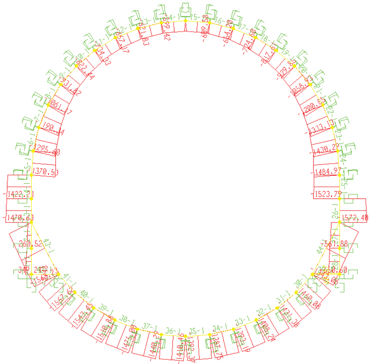
Diagramma azione assiale – SLE sisma up
