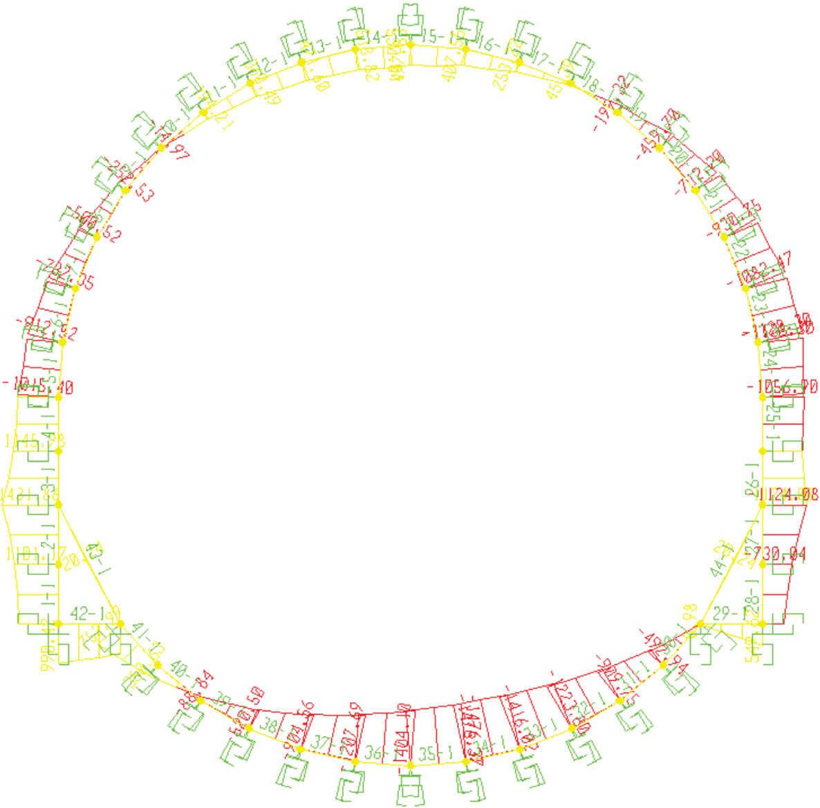
Diagramma momento flettente – SLE sisma up
