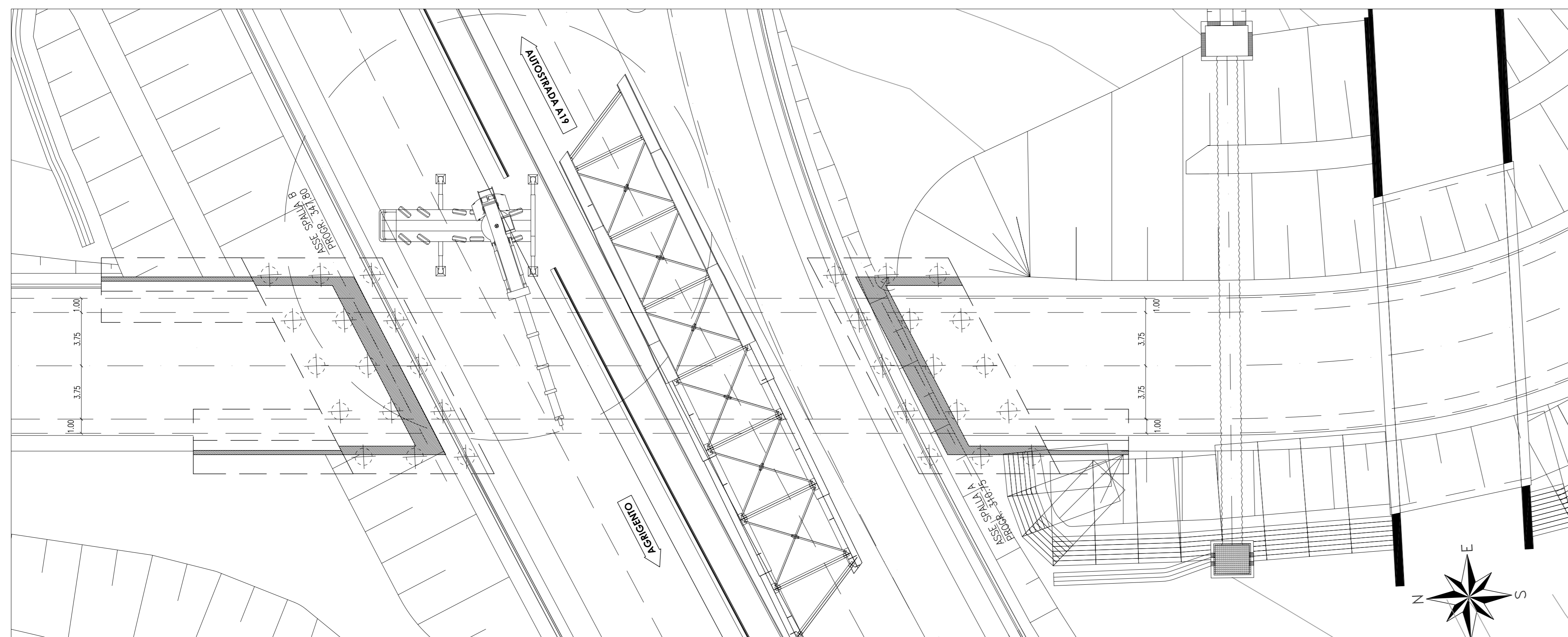
PLANIMETRIA
