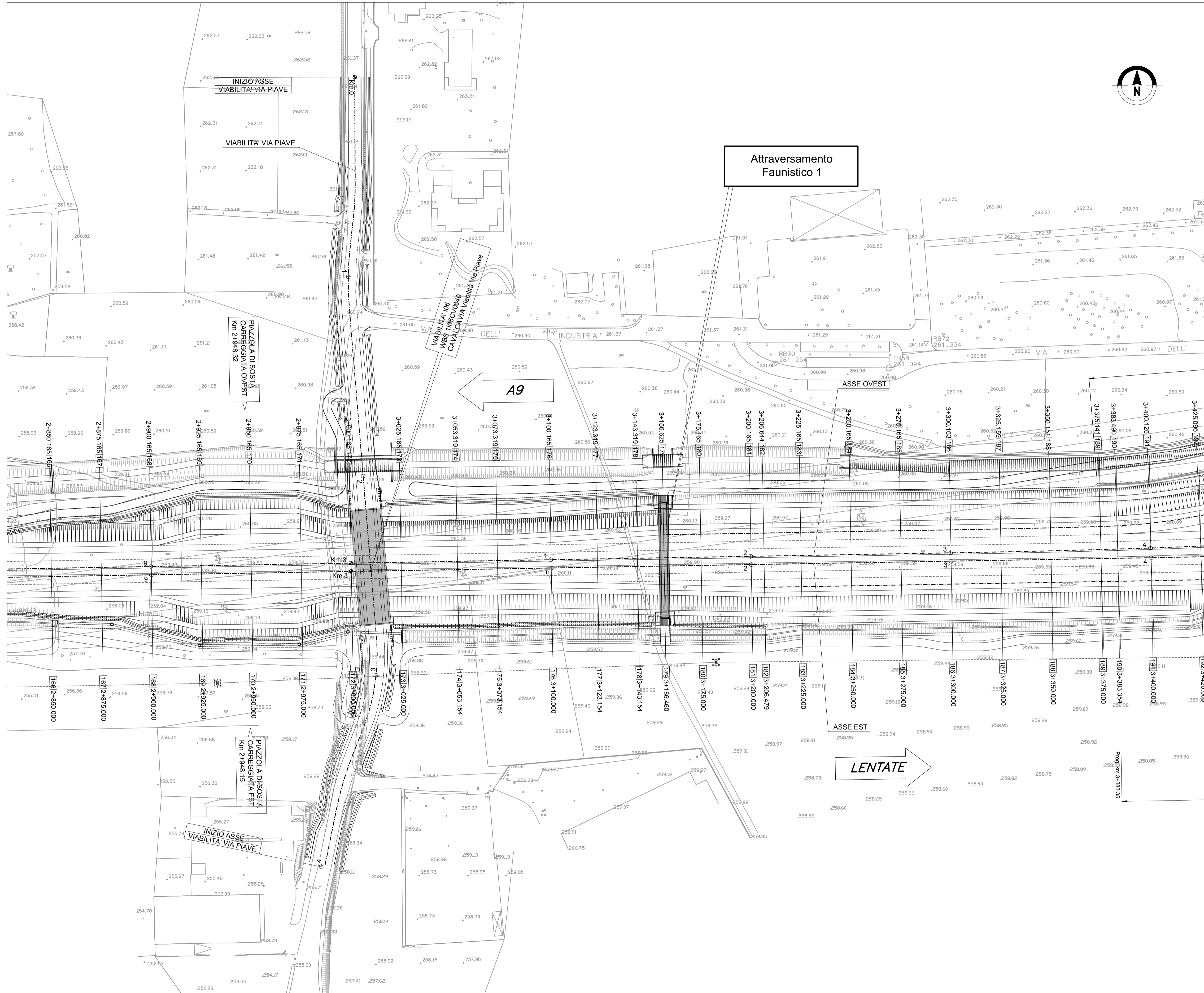
PLANIMETRIA SCALA 1 : 1000
