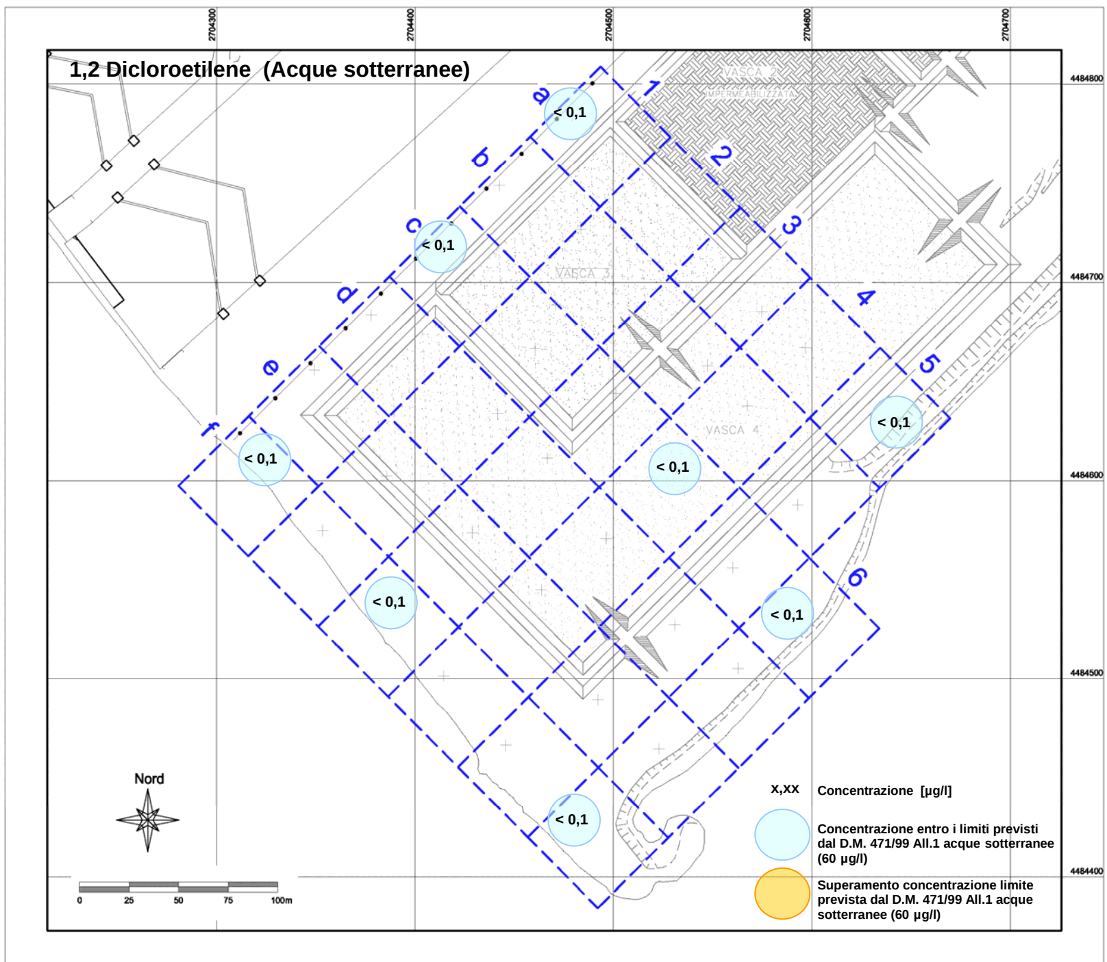
Tav. 71: 1,2 Dicloroetilene (Acque sotterranee)
