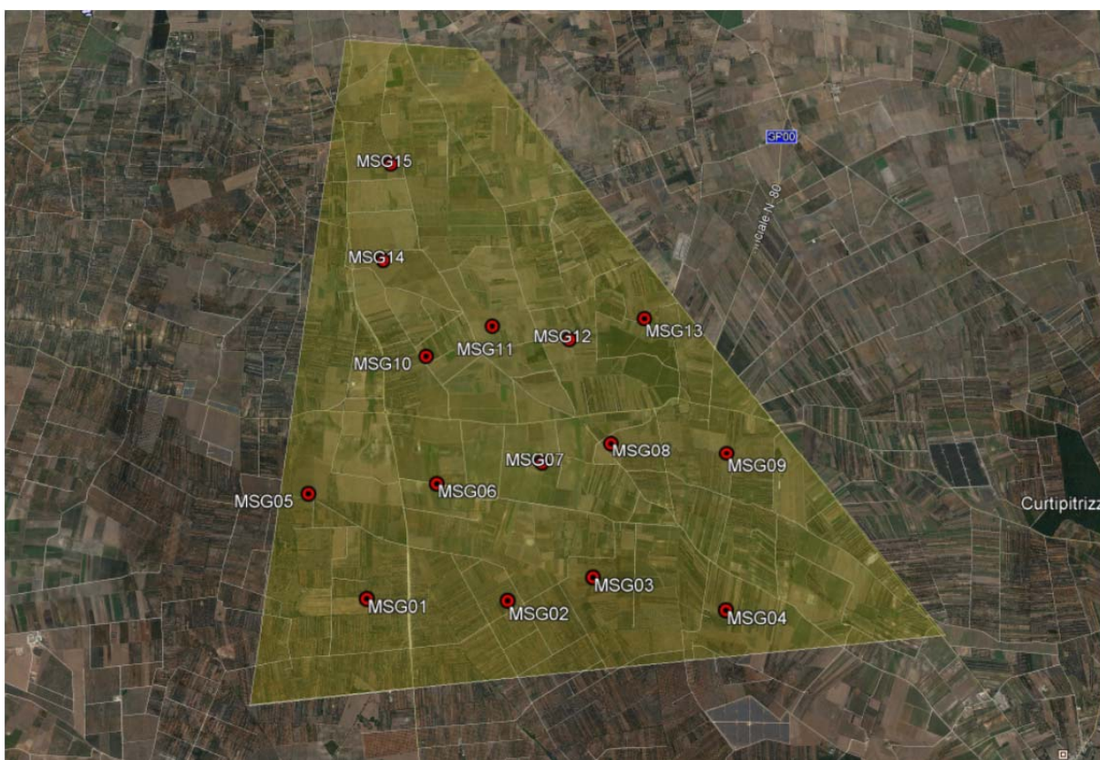
Geometria di impianto- Gli aerogeneratori sono confinati in un'area di forma quadrangolare
