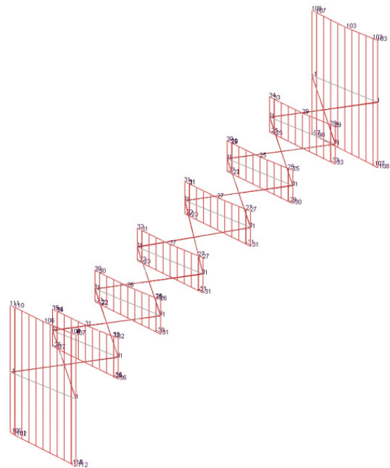
Inviluppo Taglio
