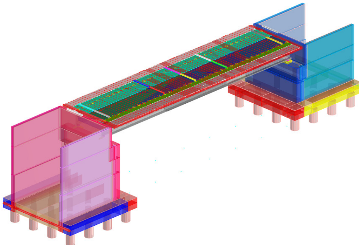
Modello 3d della struttura
