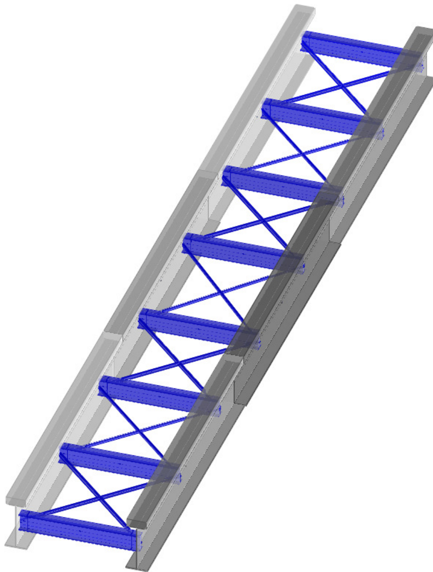
Dettaglio 3d dell'impalcato metallico
