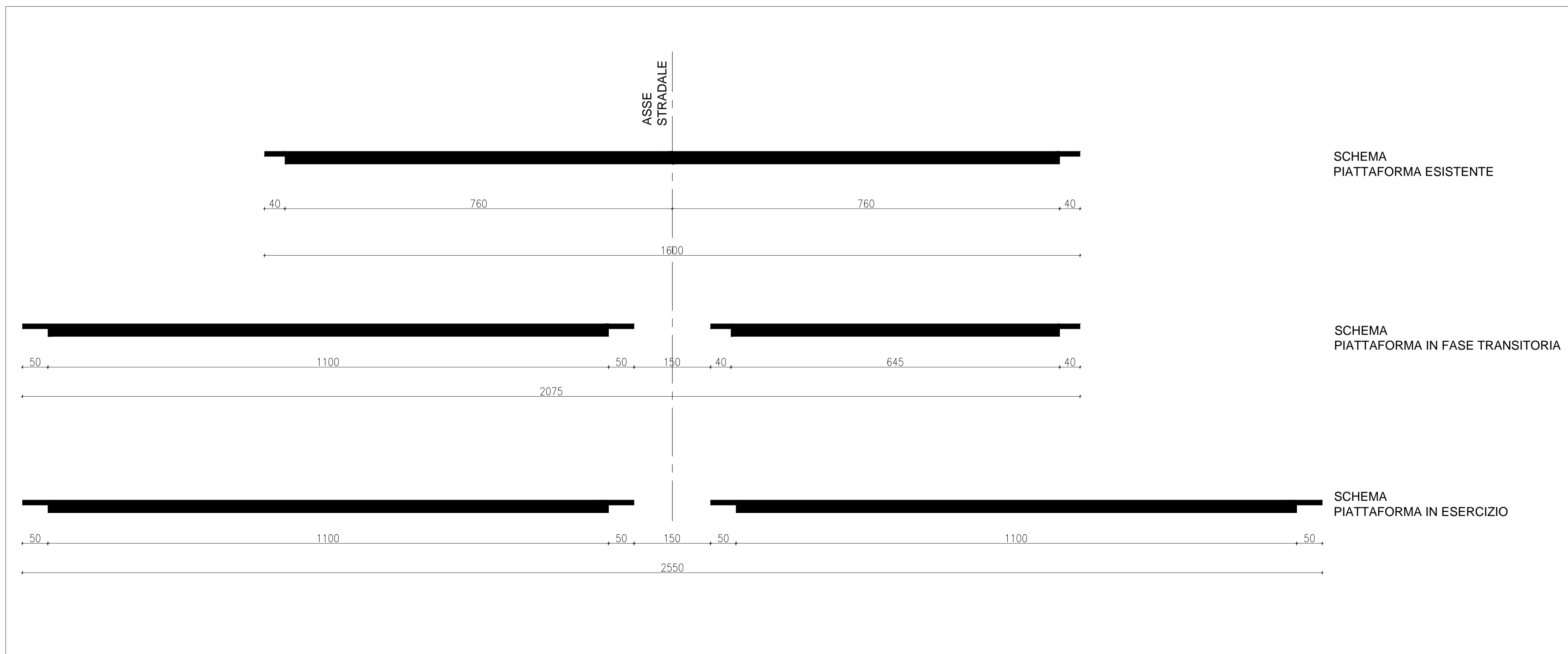
SCHEMA DISPOSIZIONI PIATTAFORMA STRADALE - scala 1:50
