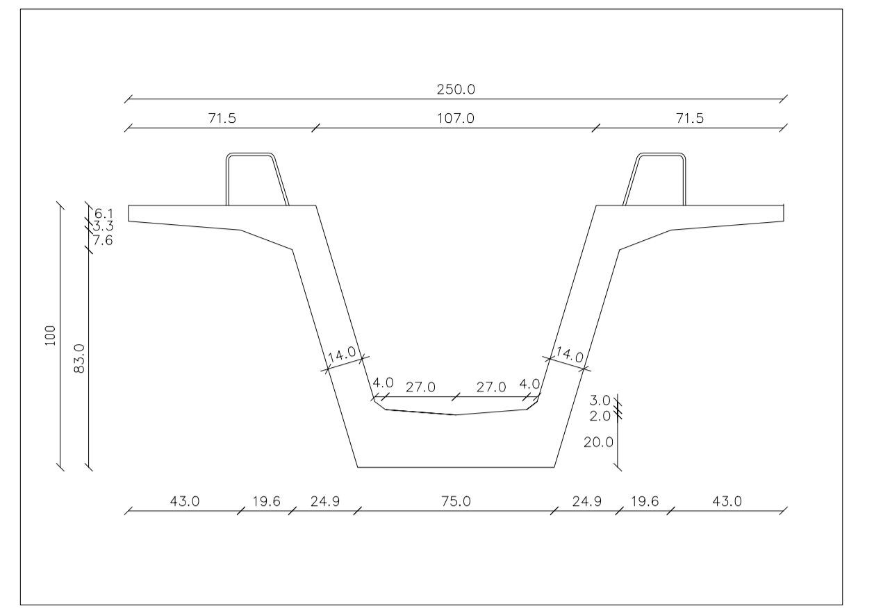
SEZIONE TRAVE PREFABBRICATA TIPO n°5 TRAVI VH100N i = 2.40 m
