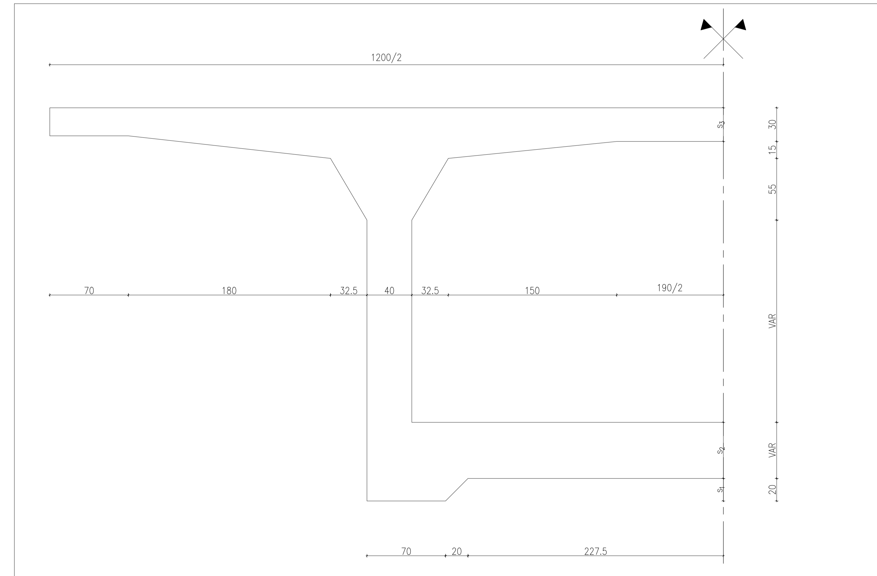
SEZIONE TIPOLOGICA TRAVE A CASSONE - scala 1:20
